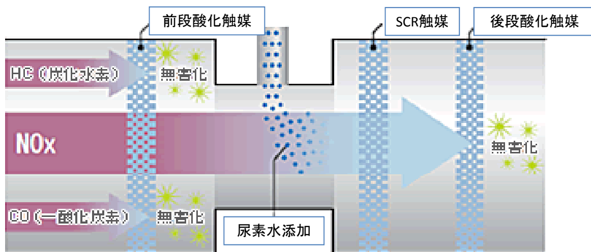
尿素SCRシステムの排出ガス処理イメージ
