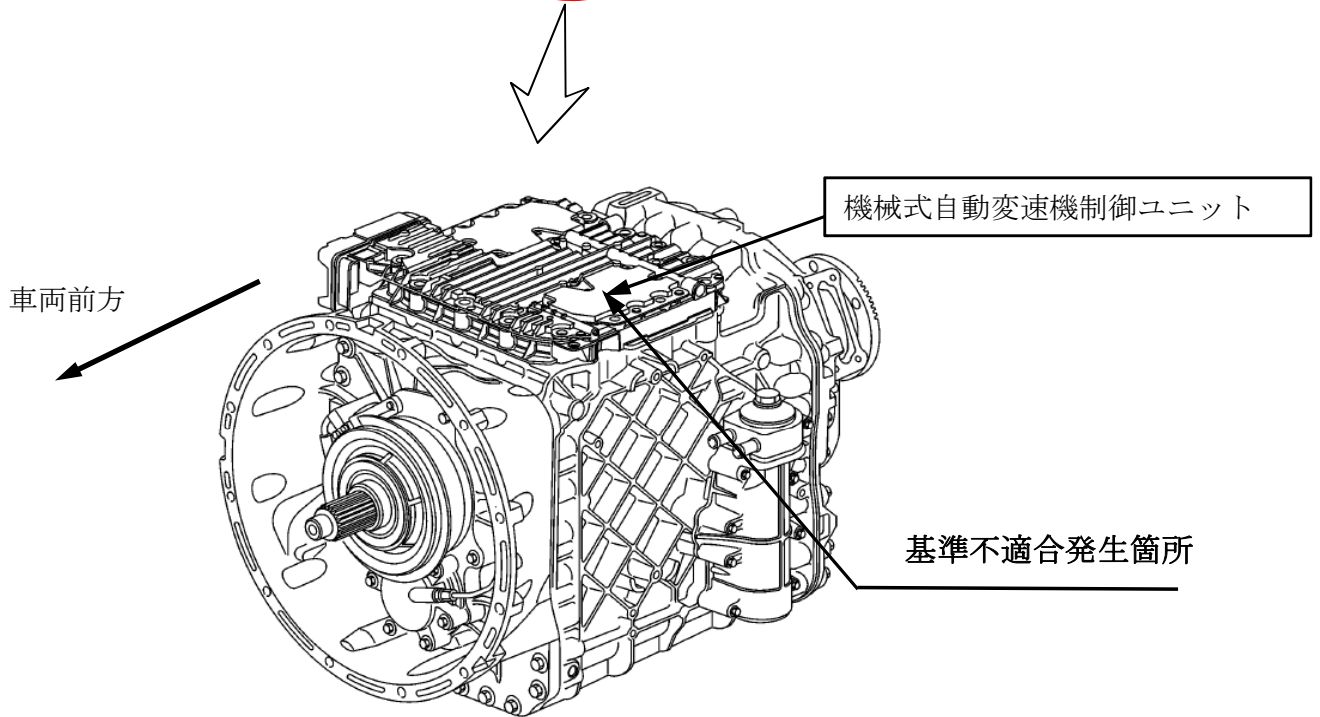
機械式自動変速機
