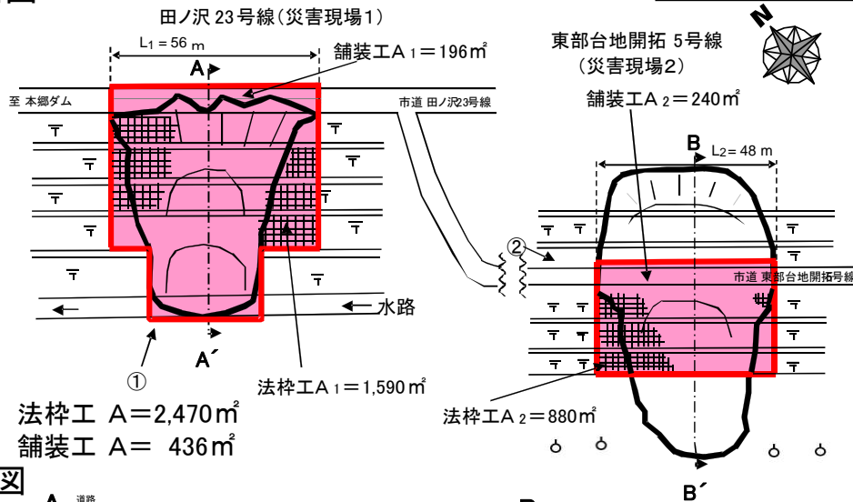
平面図
