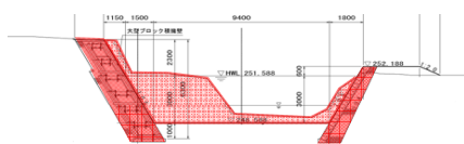
横断図(A-A')
