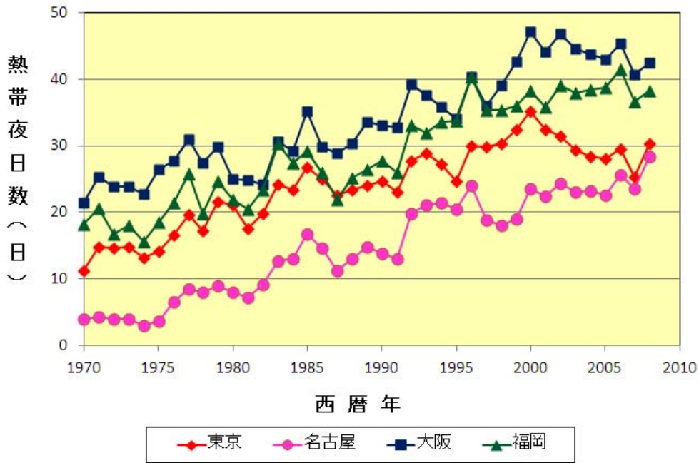
図3 4都市における熱帯夜日数(5年移動平均)(出典:気象庁) 各地点について、年間の最低気温25℃以上の日数を5年移動平均したもの
