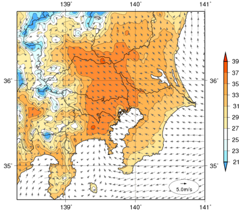
図4 首都圏の夏のヒートアイランド現象の解析結果例(出典:気象庁) 平成 22 年 8 月 17 日午後3時における気温と風の分布。
