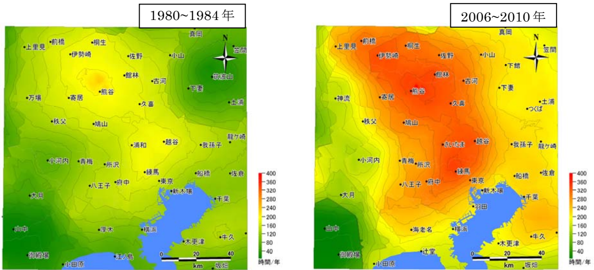
図2 関東地方における30℃以上の合計時間数の分布(出典:環境省)
