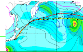
ウェザールーティングシステム
