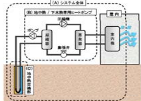
地中熱ヒートポンプ
