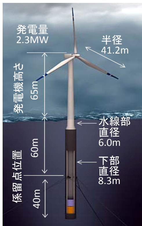
浮体式洋上風車の例
