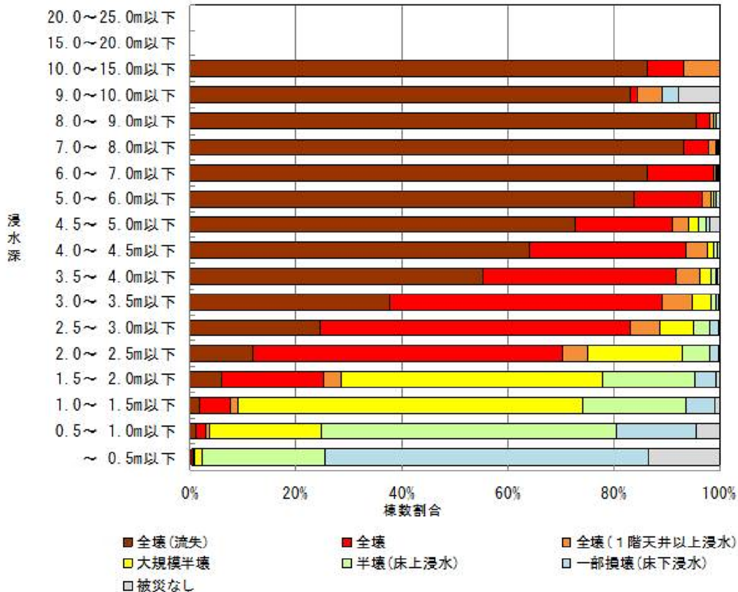
【棟数割合】 浸水深と建物被災状況の関係 (石巻市平野部以南)
