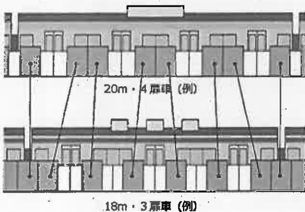
乗降位置可変ホームドア
