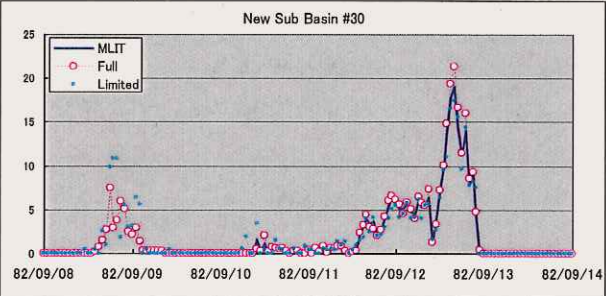
図 1d 新モデルサブ流域平均雨量 (昭和 57 年年洪水)
