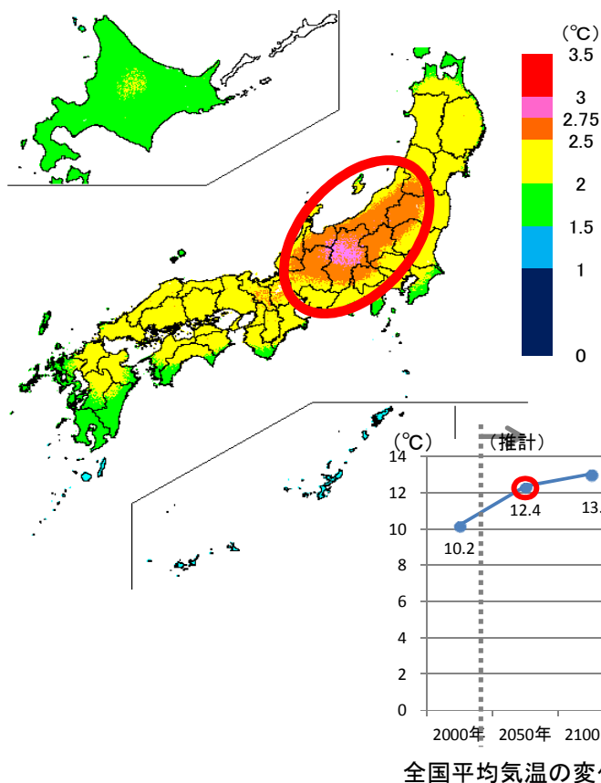
気温の上昇幅(2000年→2050年)
