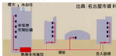
地域冷暖房システムの概要
