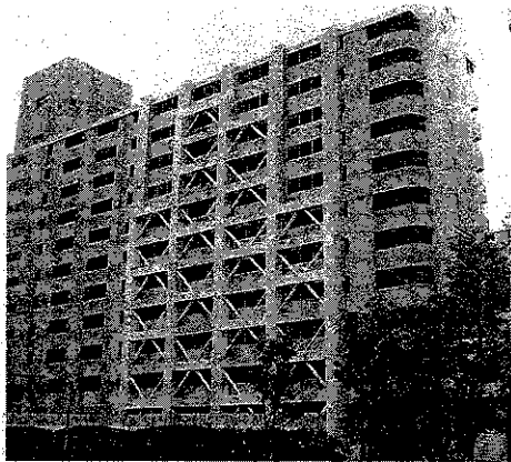
28-5号棟の耐震改修工事。左側は廊下側(10月25日写す)、右側はベランダ側(10月25日写す)の補強の様子。
