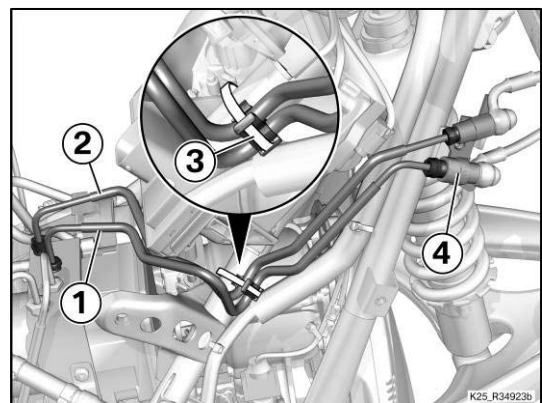
交換後の前輪用ブレーキ配管
