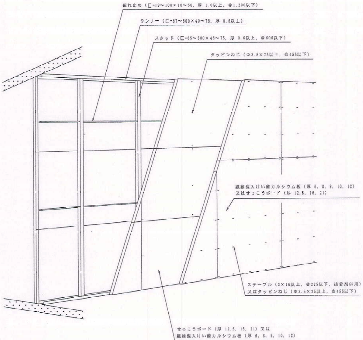
透視図
