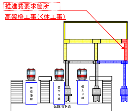
断面図 (S=1:1000)
