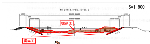
調整対象事業標準断面図
