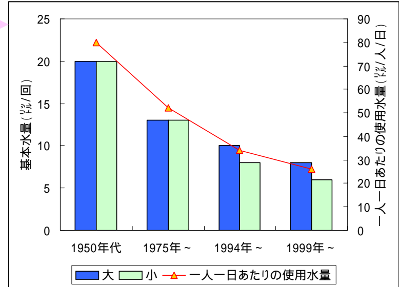
トイレの年代別使用水量の変化
