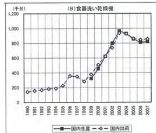
食器洗い乾燥機の国内出荷台数の内訳
