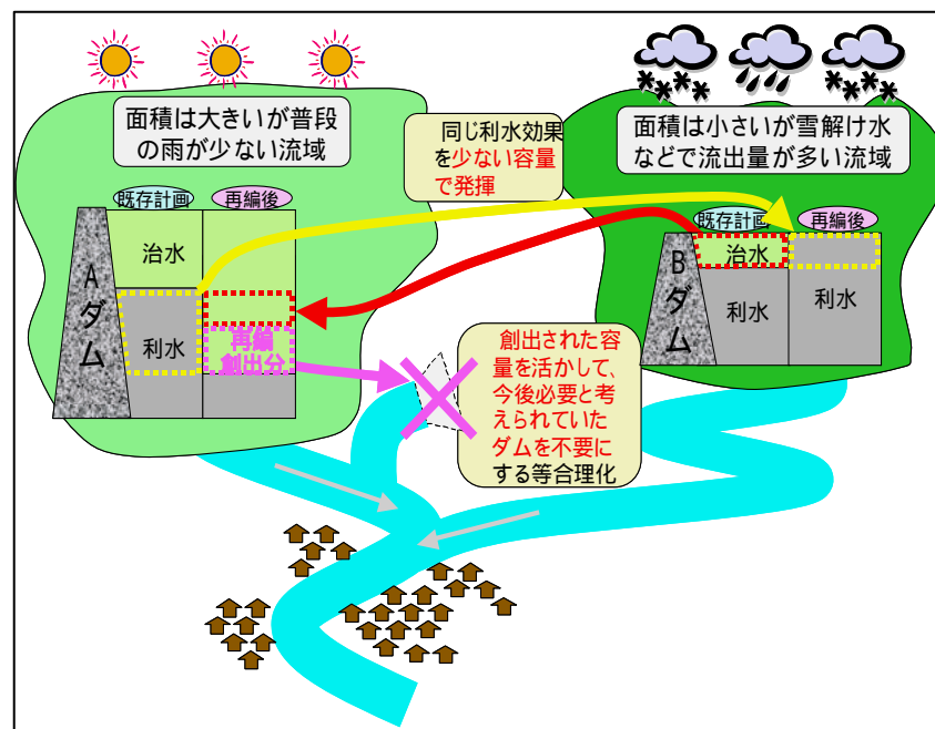
ダムの治水容量と利水容量の振り替えによる供給能力の増強 8
