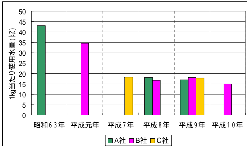
全自動洗濯機の性能向上による使用水量の変化
