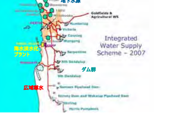
【総合水供給システム(2007年現在)】
