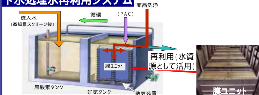
膜分離活性汚泥法のフロー
