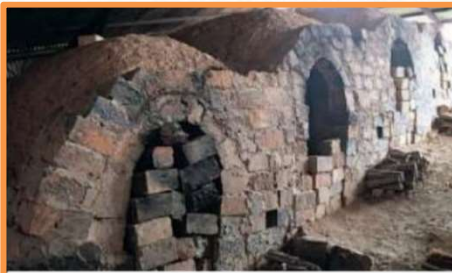
萩焼登り窯（萩焼を焼成する窯）
