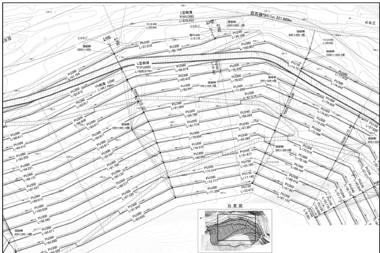
図 6-13 (2) 盛土排水計画平面図 (2/3)
