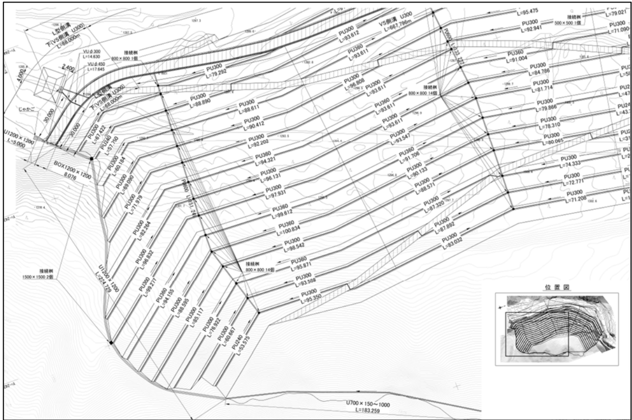
図 6-13 (1) 盛土排水計画平面図 (1/3)
