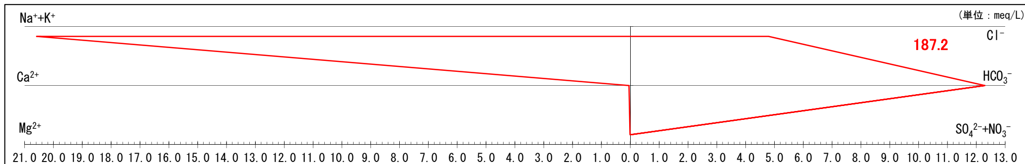
地下水 (17 田代ダム付近) 井戸深度 : GL-256m (スクリーン深度 : GL-130~-250m)
