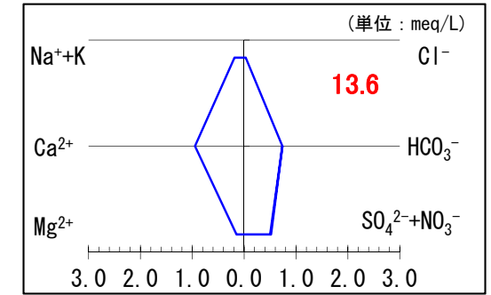
河川水 (03 大井川 (下泉橋): 川根本町) 採水標高: 210.0m
