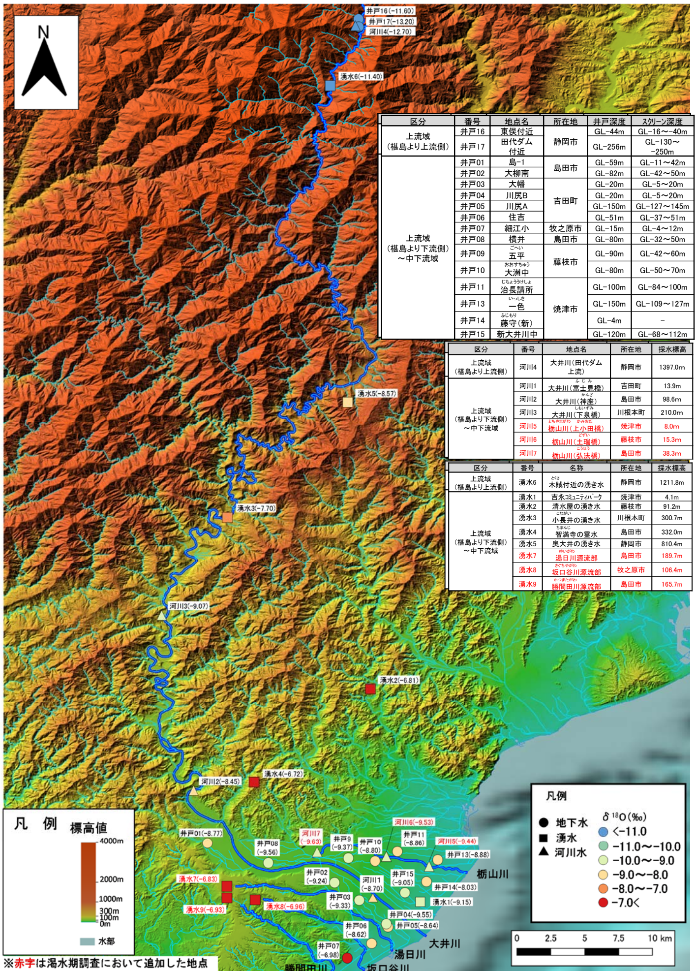
図 3-18 \delta^{18}O の測定結果の平面分布：湧水期調査
