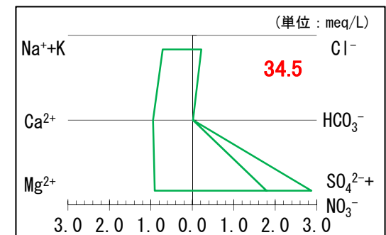
湧水 (09 勝間田川源流部 (島田市)) 採水標高 : 165.7m
