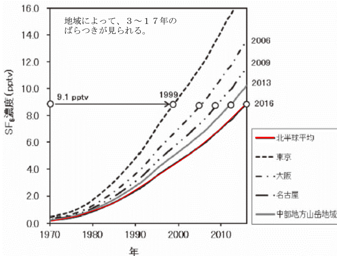
図 3-5 大気中SF 6 濃度（北半球平均値）と日本国内の補正濃度曲線
