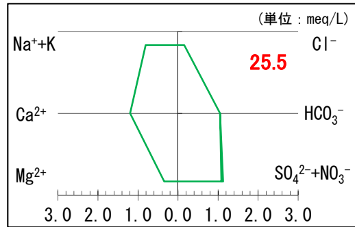
湧水 (08 坂口谷川源流部 (牧之原市)) 採水標高 : 106.4m
