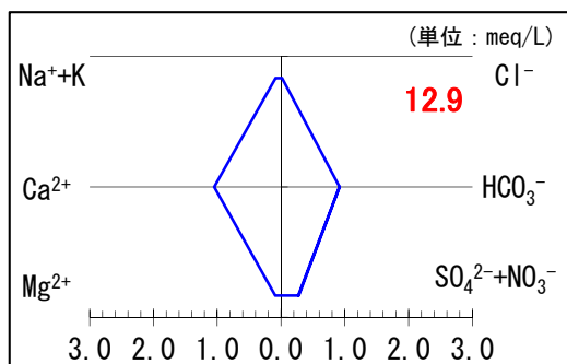
河川水 (04 大井川 (田代ダム上流) 採水標高 : 1,397m)
