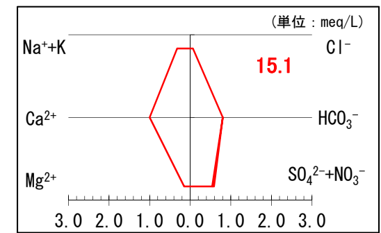
地下水 (03 大幡 (吉田町))
