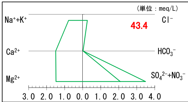
湧水 (07 湯日川源流部 (島田市)) 採水標高 : 189.7m
