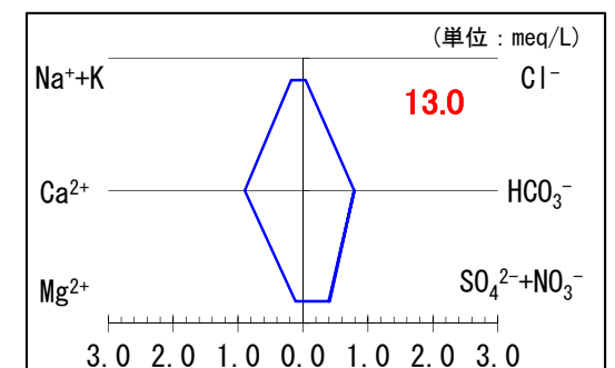
河川水 (07 栃山川 (弘法橋): 島田市) 採水標高: 38.3m
