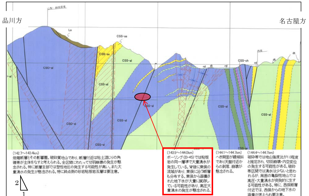
図 10-12 地質縦断図と施工上の留意点
