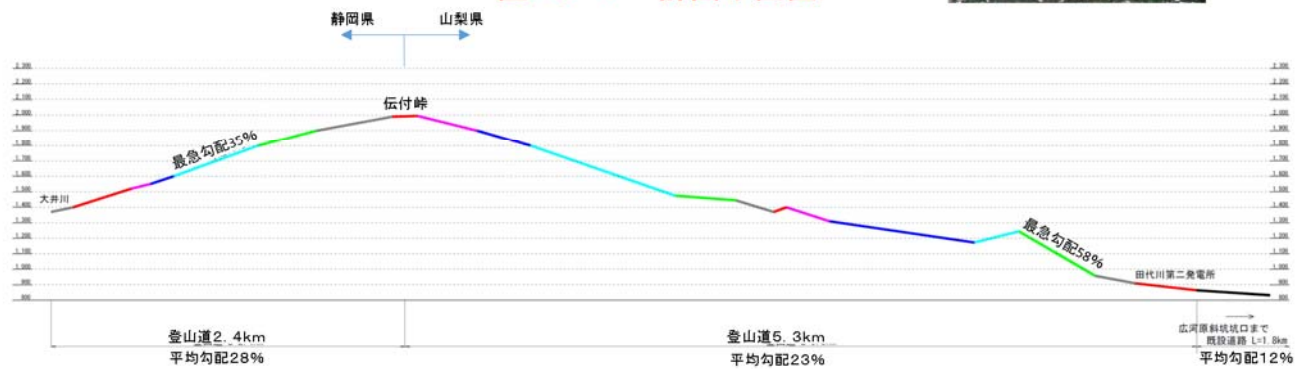
図 8-2 計画縦断面図
