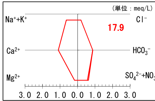
地下水 (11 治長請所 (焼津市)) 井戸深度：GL-100m (スクリーン深度：GL-84～100m)
