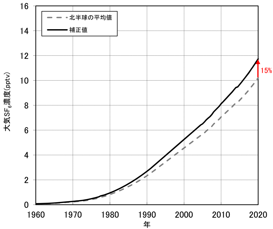
図 3-1 2 大気中の SF 6 濃度の経年変化曲線 (北半球平均値) の補正結果 : 豊水期調査
