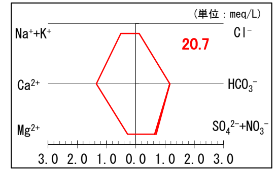
地下水 (13 一色 (焼津市)) 井戸深度：GL-150m (スクリーン深度：GL-109～127m)
