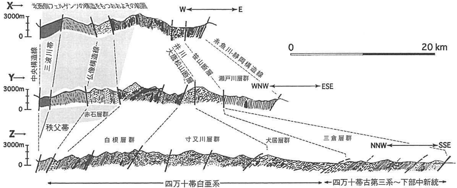
図 2-30 赤石山地秩父帯・四万十帯の模式断面図
