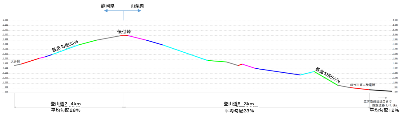
図 4.60 計画縦断面図
