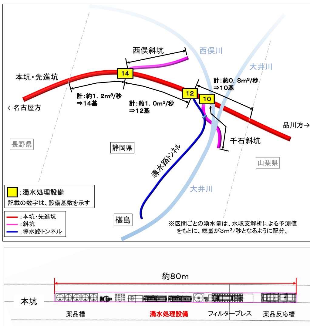
図 4.47 濁水処理設備の配置計画 (仮に3m 3 /秒の濁水が発生した場合)
