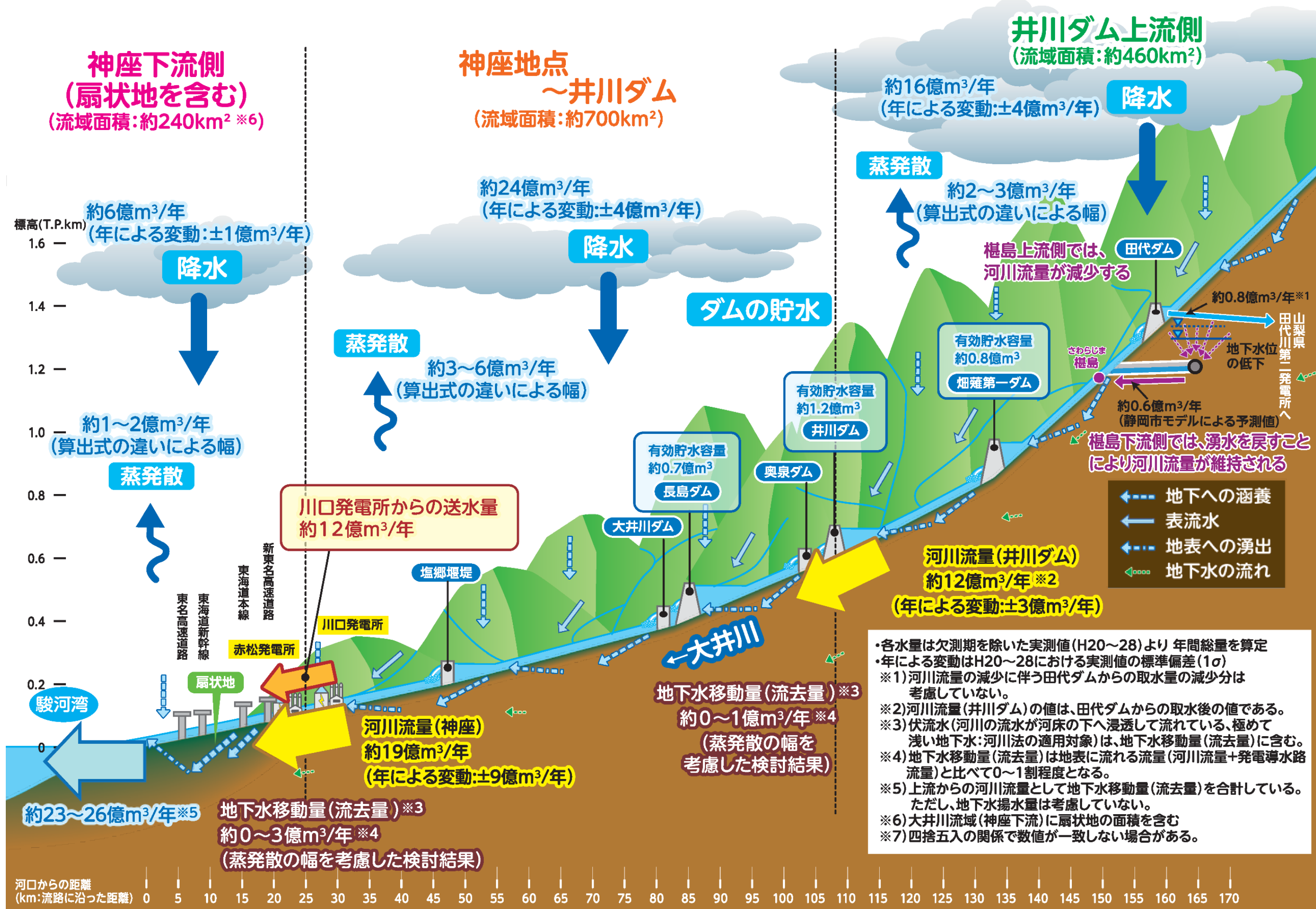
図 4.33 大井川流域の水循環の概要図 (掘削完了時の水循環量)
