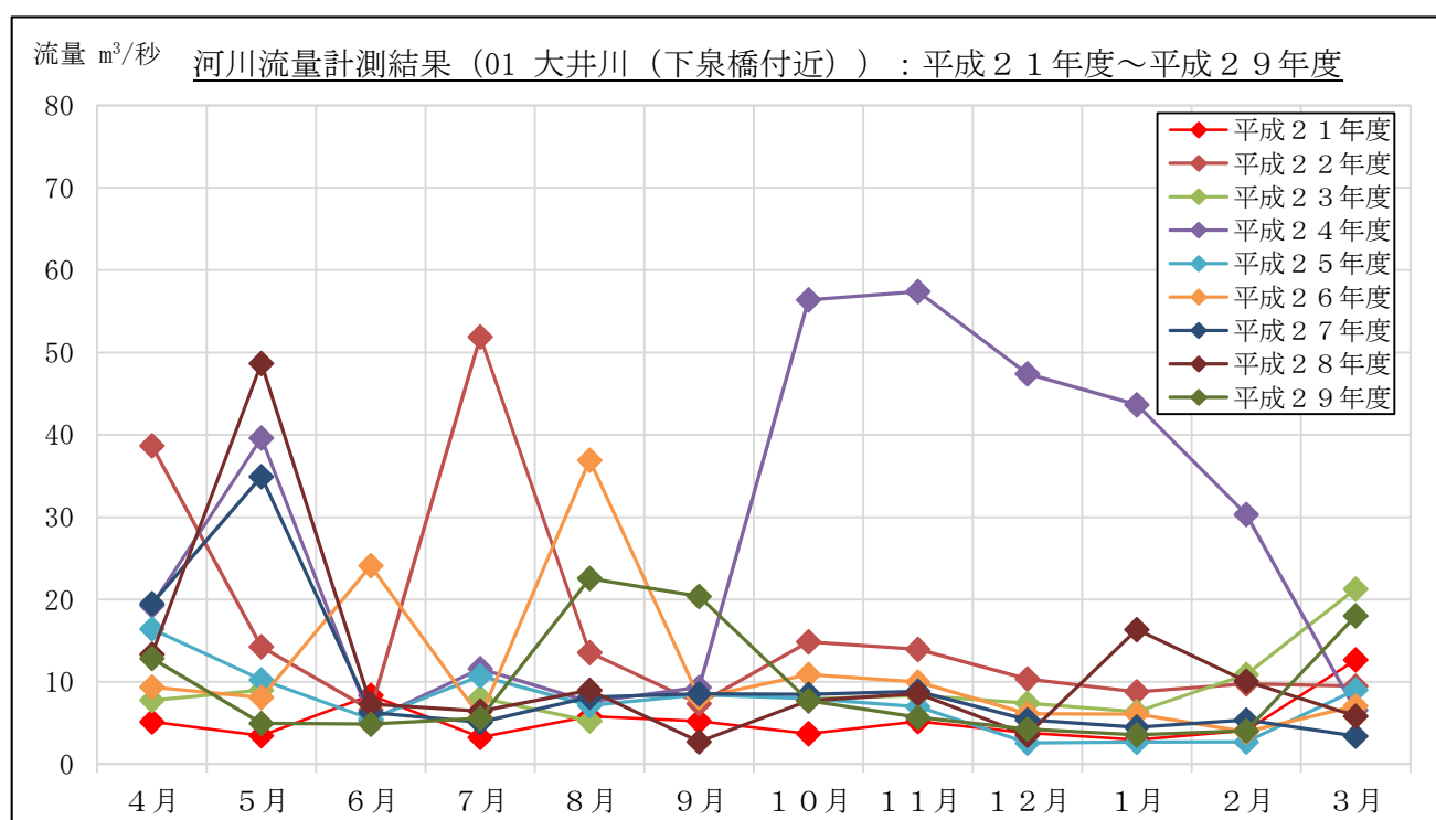
図 2-10 流量計測結果：01 大井川 (下泉橋付近)
