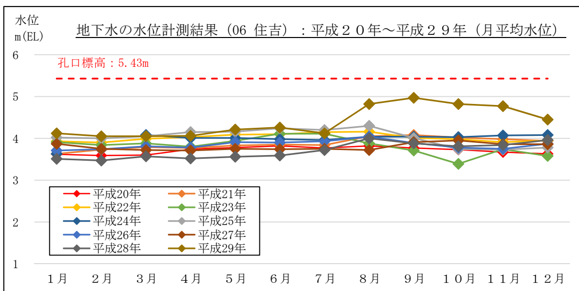
図 2-21 地下水の水位計測結果 (月平均水位) : 06 住吉 (吉田町住吉)
