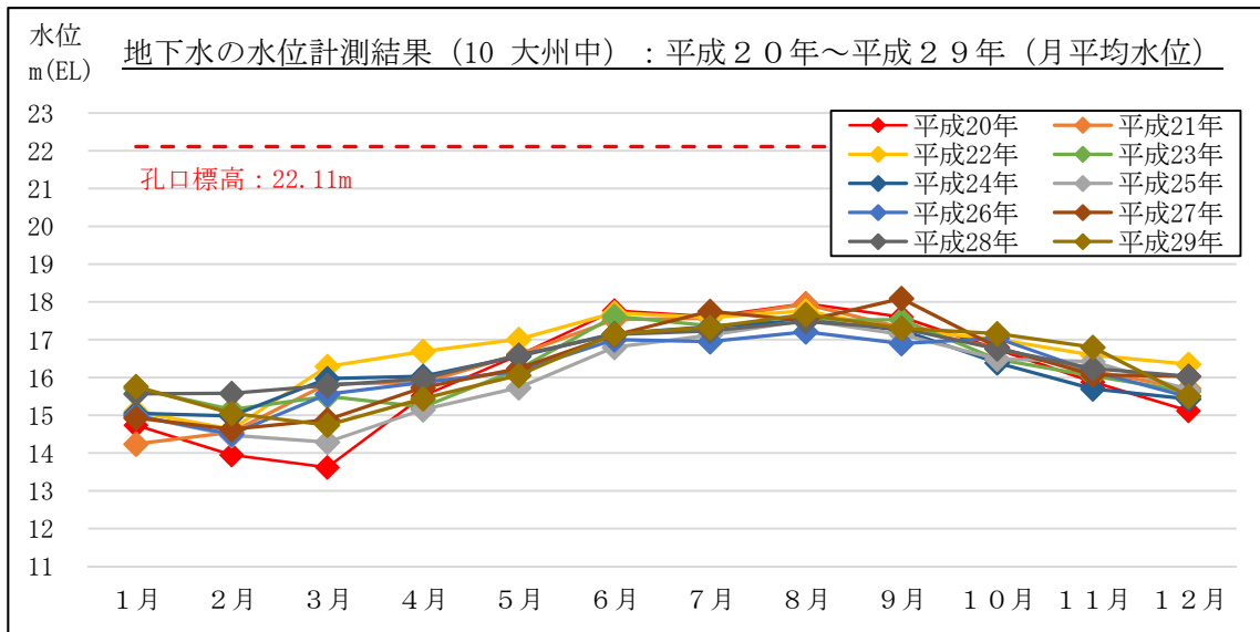
図 2-25 地下水の水位計測結果 (月平均水位) : 10 大州中 (藤枝市弥左工門)
