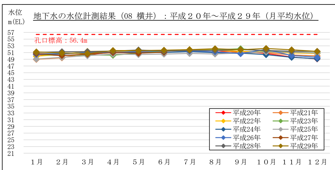
図 2-2 3 地下水の水位計測結果 (月平均水位) : 08 横井 (島田市横井)
