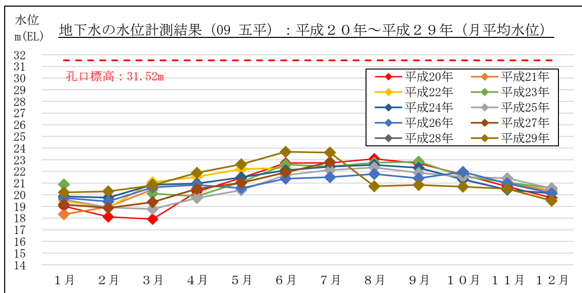
図 2-2 4 地下水の水位計測結果 (月平均水位) : 09 五平 (藤枝市大西町)
