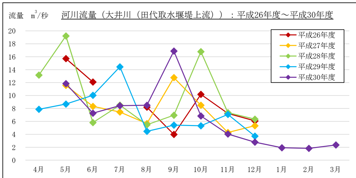
図 2-6 流量計測結果（月1回計測：田代取水堰堤上流）
