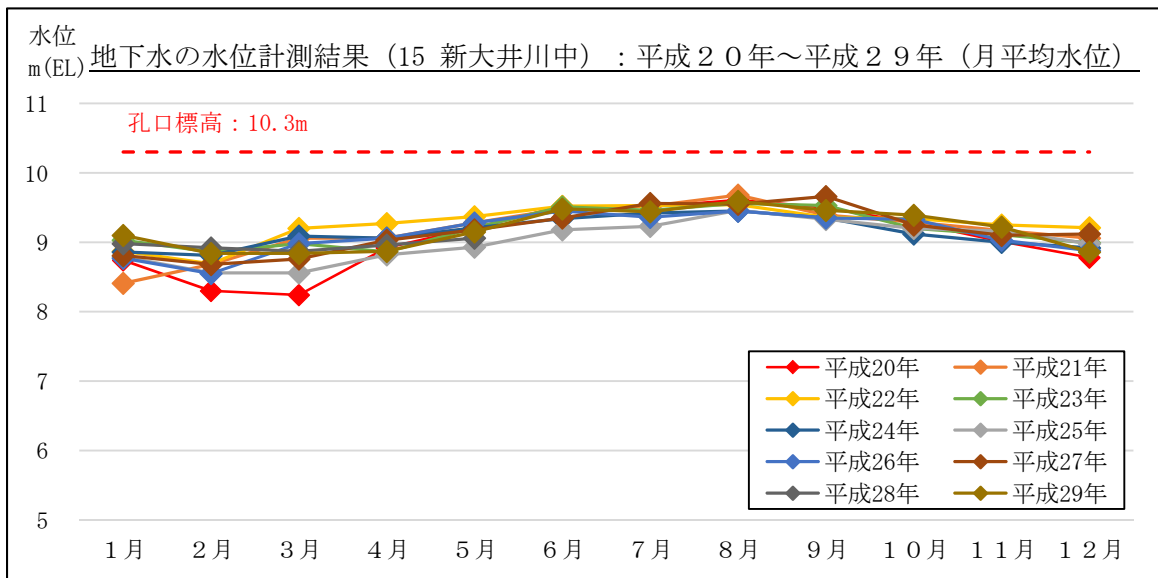
図 2-30 地下水の水位計測結果 (月平均水位) : 15 新大井川中 (焼津市下江留)
