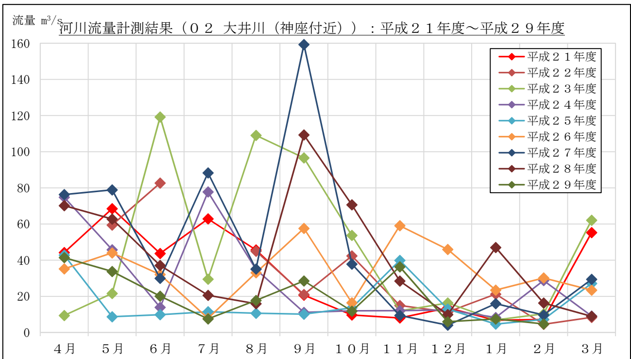
図 2-11 流量計測結果 : 02 大井川 (神座 かんざ 付近)
