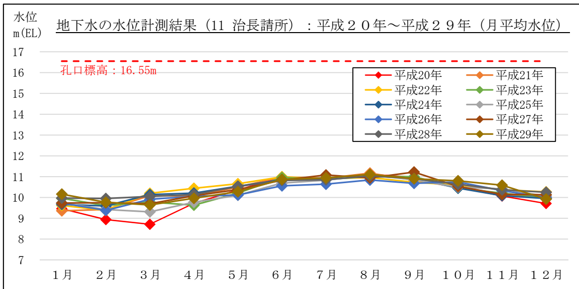
図 2-26 地下水の水位計測結果 (月平均水位) : 11 治長請所 (焼津市治長請所)
