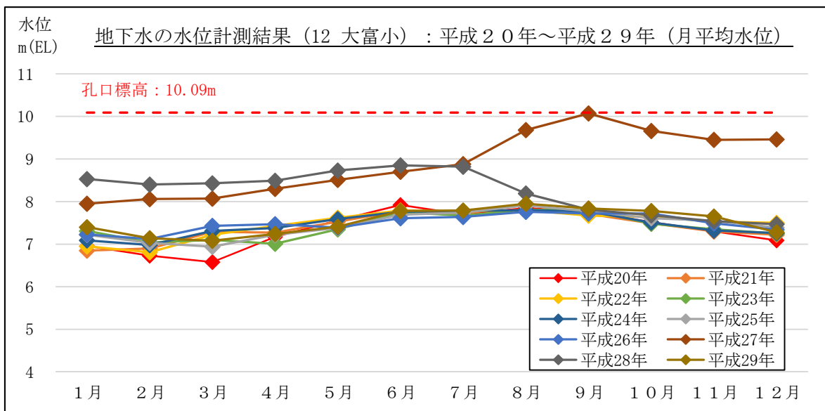
図 2-27 地下水の水位計測結果 (月平均水位) : 12 大富小 (焼津市中根新田)
