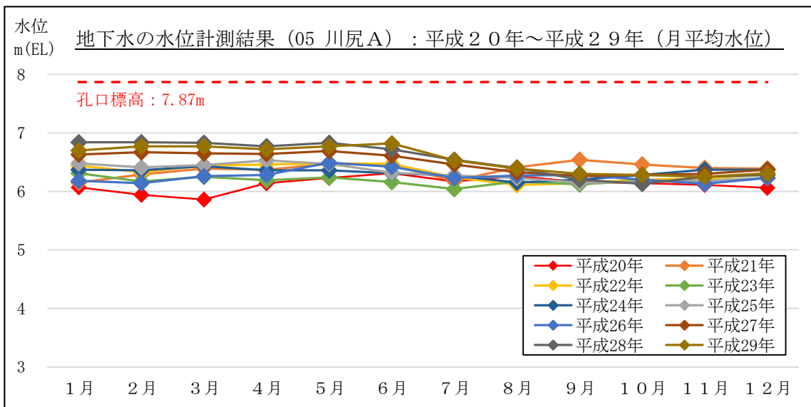
図 2-20 地下水の水位計測結果 (月平均水位) : 05 川尻A (吉田町川尻)
