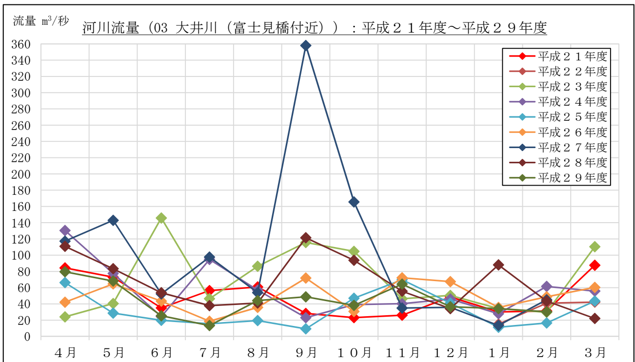
図 2-12 流量計測結果 : 03 大井川 (富士見 ふじみ 橋付近)
