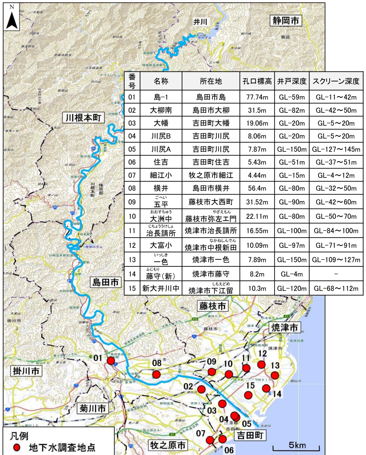
図 2-14 地下水の水位 調査地点図 (大井川下流域)
