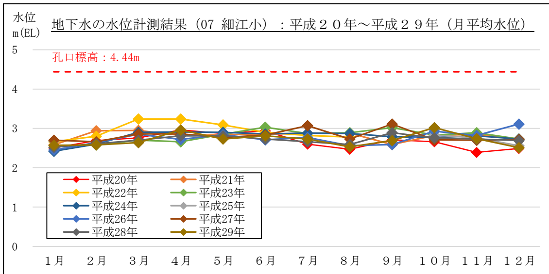
図 2-2 2 地下水の水位計測結果 (月平均水位) : 07 細江小 (牧之原市細江)
