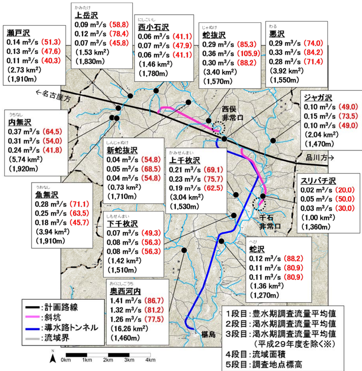
図 2-8 上流域の沢等の流量（年2回計測）調査結果
