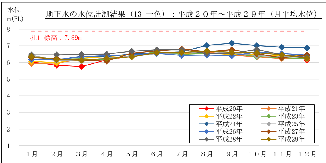
図 2-28 地下水の水位計測結果 (月平均水位) : 13 一色 (焼津市一色)
