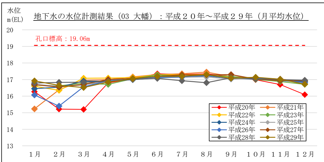
図 2-18 地下水の水位計測結果 (月平均水位) : 03 大幡 (吉田町大幡)
