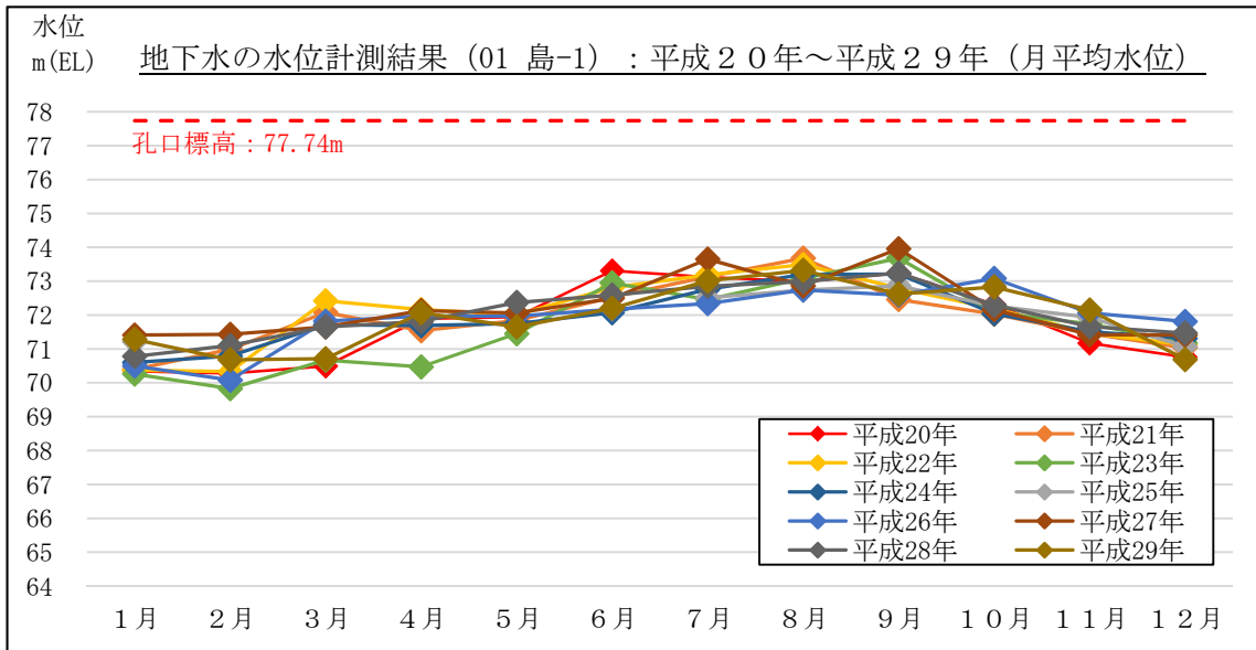
図 2-16 地下水の水位計測結果 (月平均水位) : 01 島-1 (島田市島)
