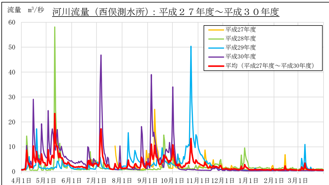
図 2-5 流量計測結果（常時計測：西俣測水所）
