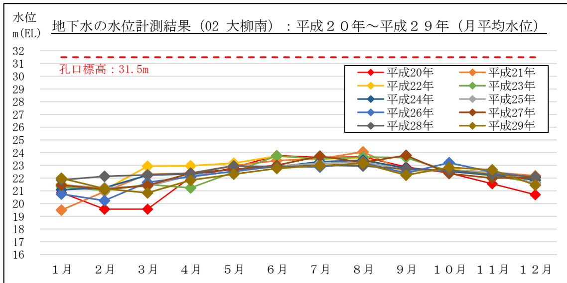
図 2-17 地下水の水位計測結果 (月平均水位) : 02 大柳南 (島田市大柳)
