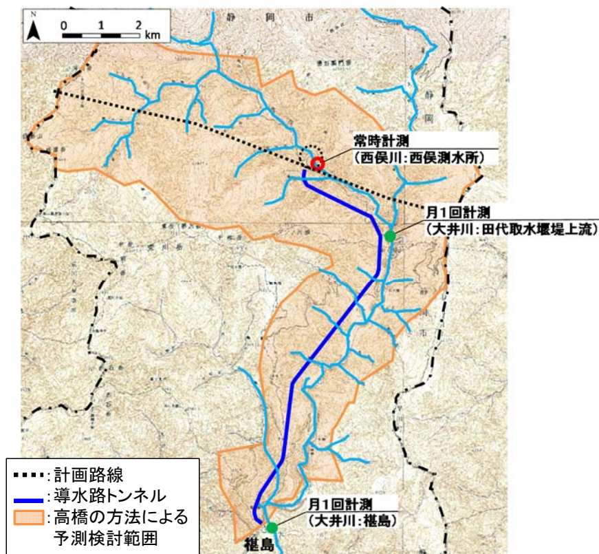
図 2-4 河川流量の調査地点
