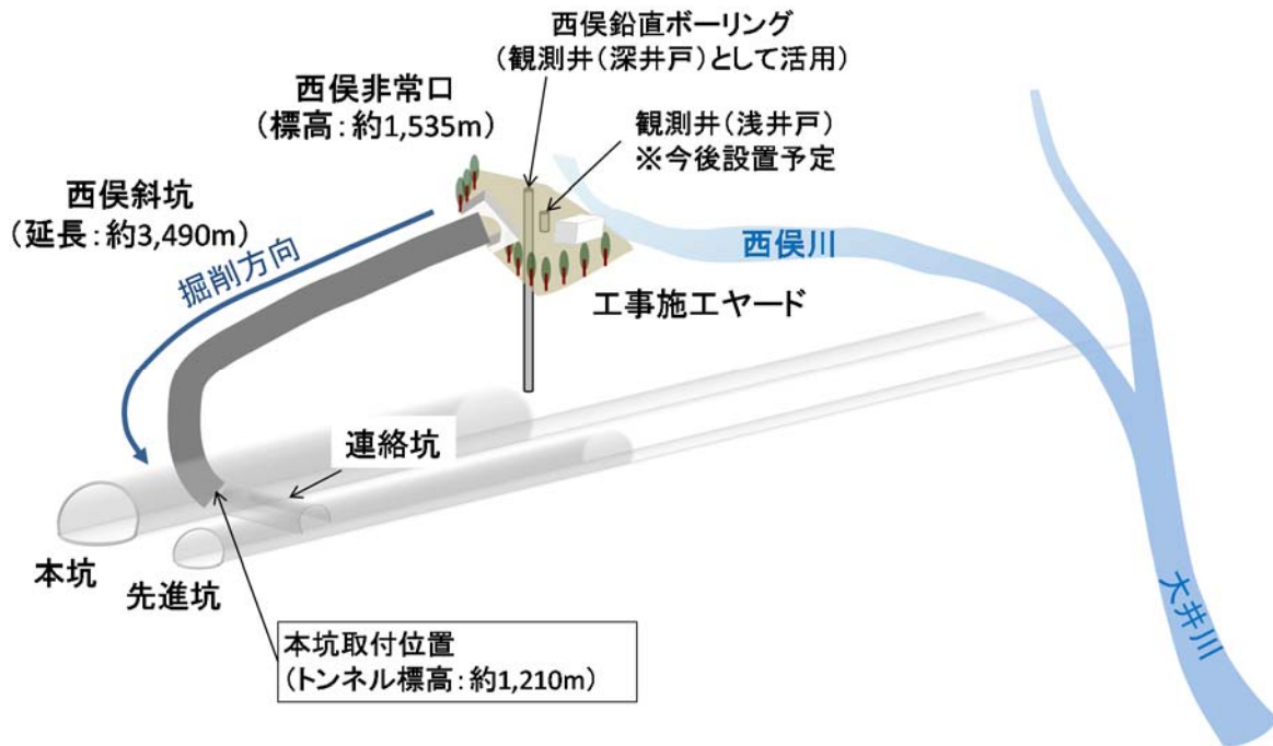
図 5.12 西俣斜坑 概念図
