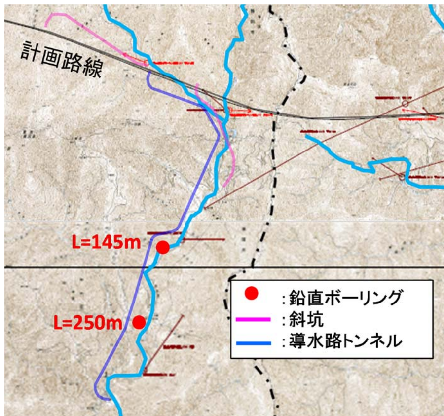
図 5.19 ボーリング調査平面図
