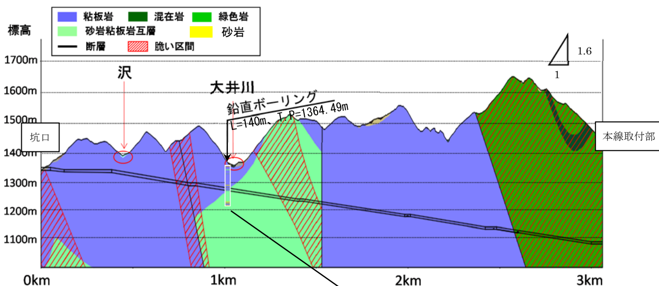
図 5.10 千石斜坑 縦断面図 拡大図
