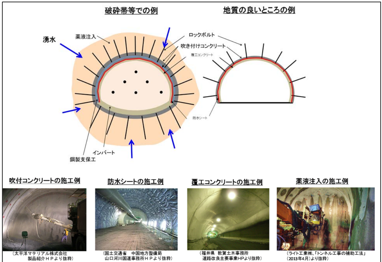
図 5.7 本坑におけるトンネル湧水量低減対策
