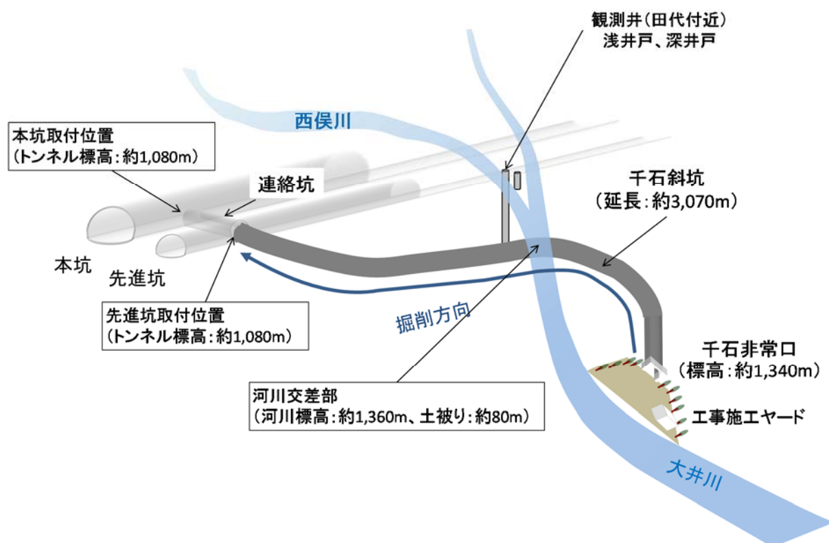
図 5.8 千石斜坑 概念図
