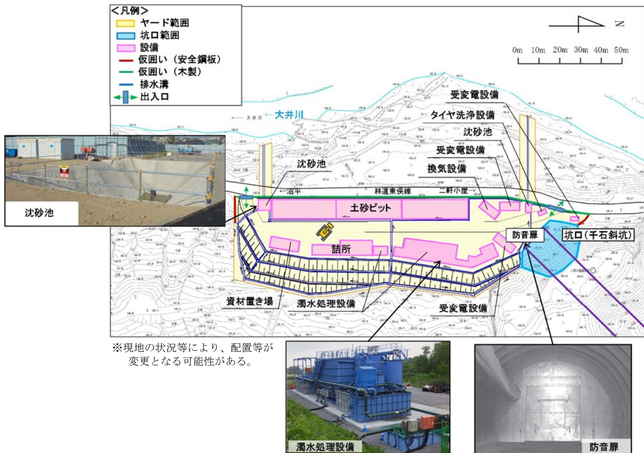
図 5.9 千石斜坑ヤードの計画図
