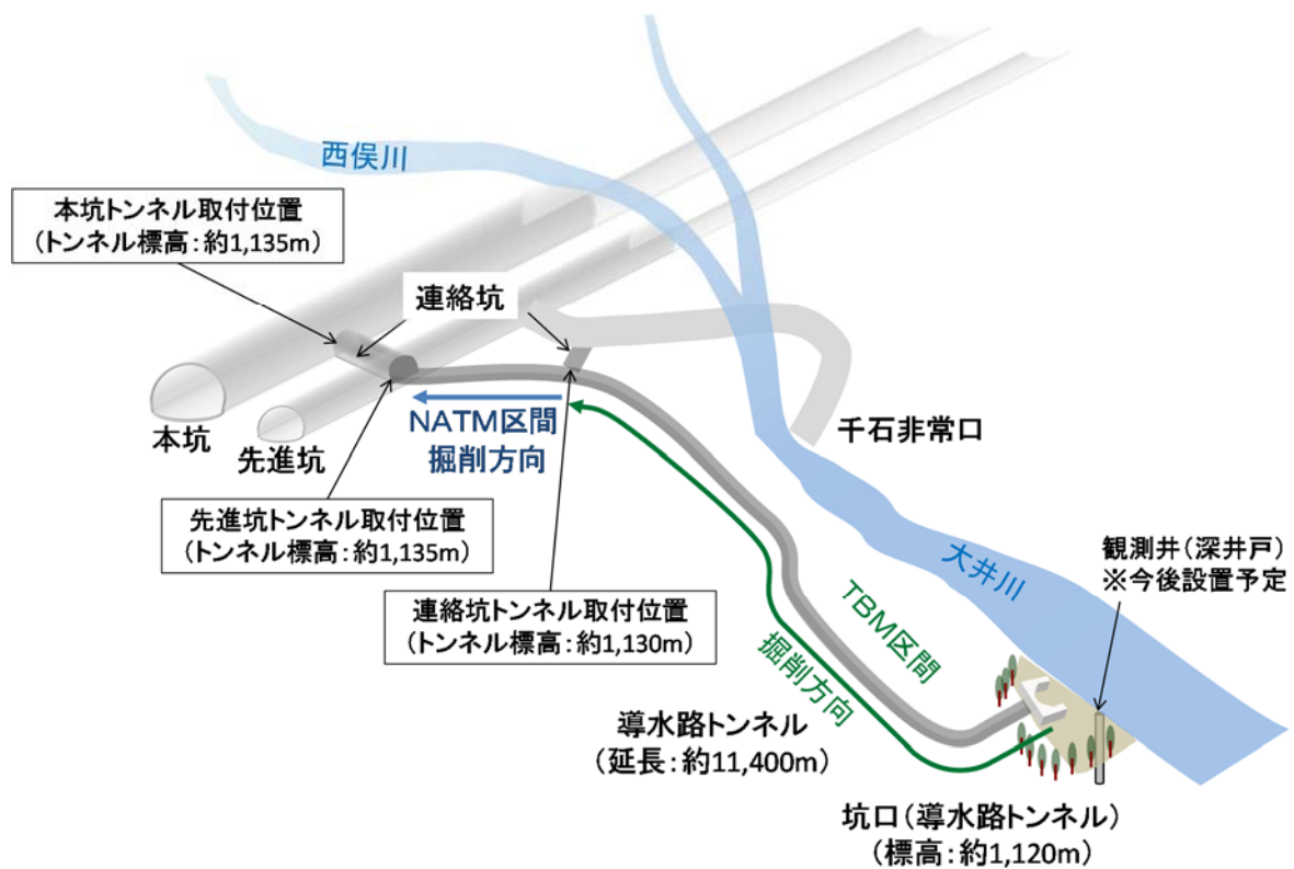
図 5.16 導水路トンネル 概念図
