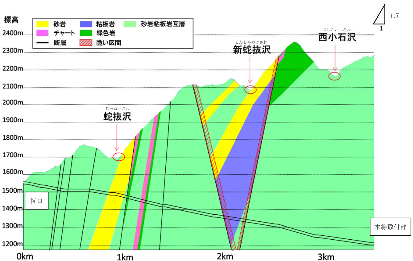
図 5.14 西俣斜坑 縦断図
