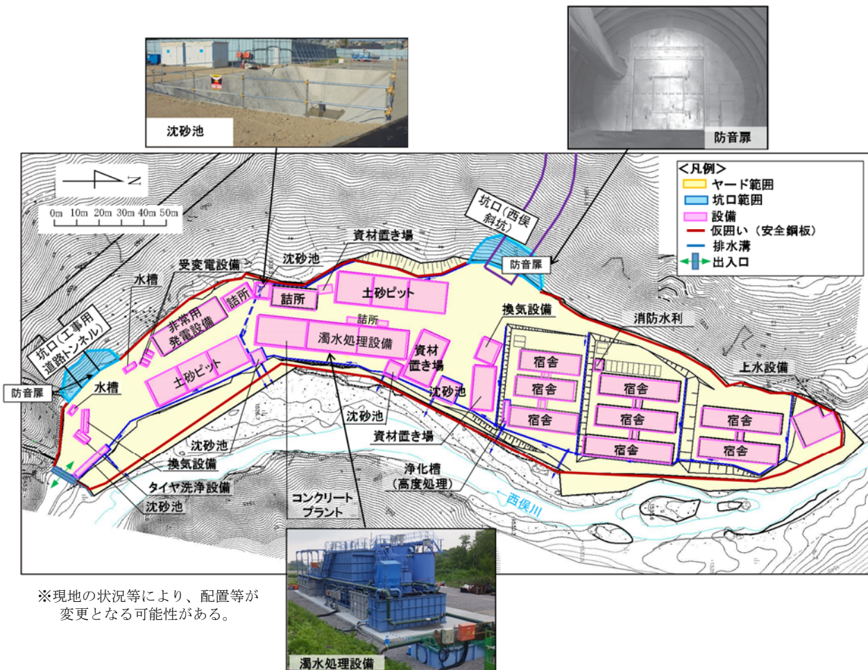
図 5.13 西俣斜坑ヤードの計画図
