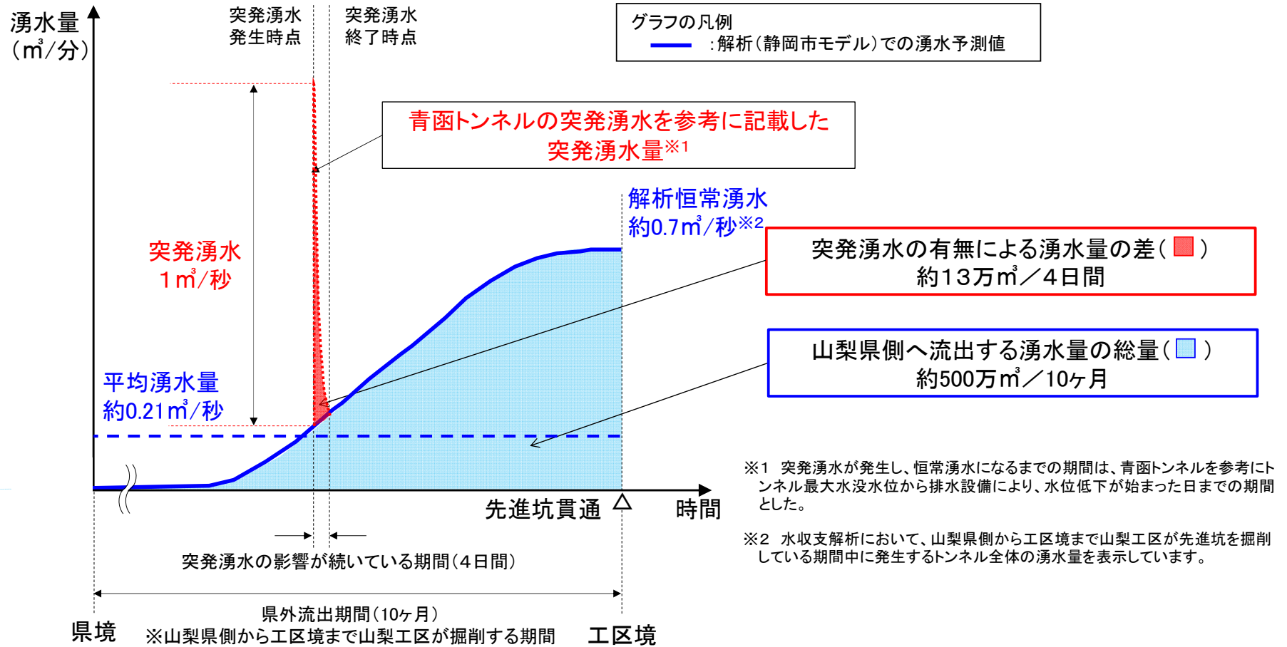
図 7-7 モデルケースによる突発湧水量と解析(静岡市モデル)による山梨県側へ流出する湧水量の総量の比較(イメージ)
