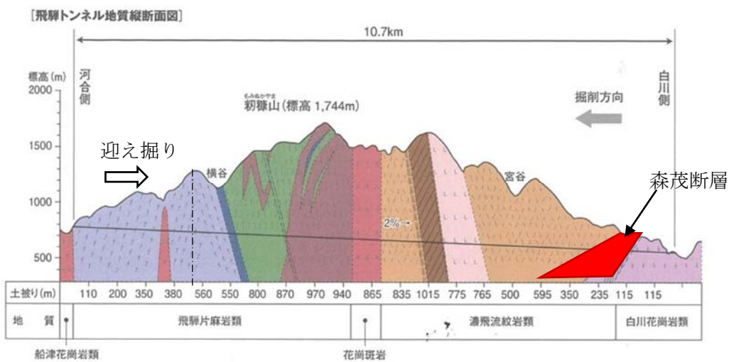
図 7-16 飛騨トンネル地質縦断面図
