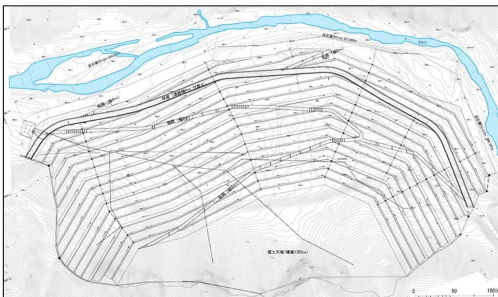
図 6-8 燕沢付近発生土置き場 計画平面図
