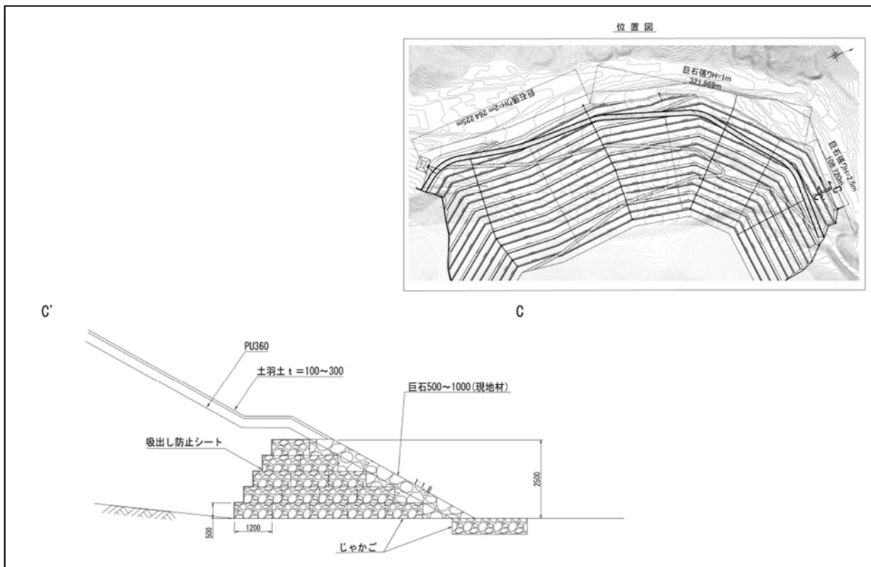
図 6-11 盛土のり尻巨石積み詳細図
