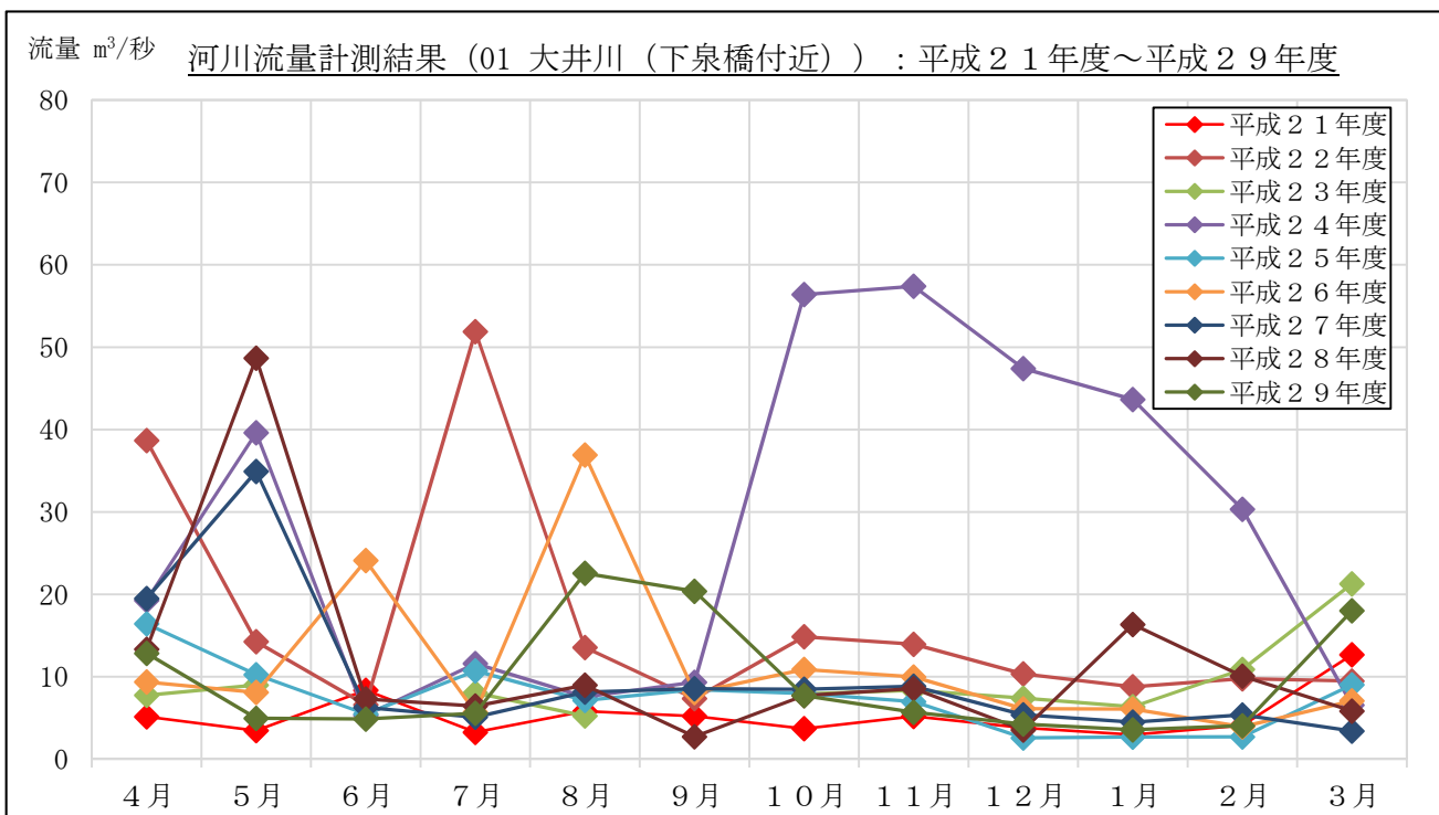
図 2-9 流量計測結果：01 大井川 (下泉橋付近)
