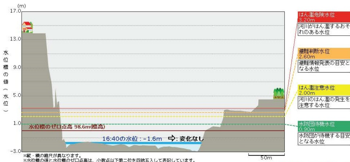
図 2-2 大井川（ かんざ 神座地点）の断面図
