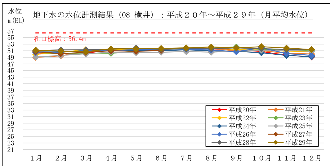
図 2-2 2 地下水の水位計測結果 (月平均水位) : 08 横井 (島田市横井)
