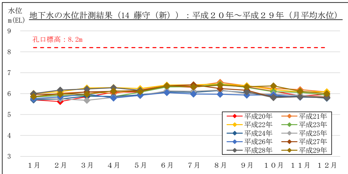
図 2-28 地下水の水位計測結果 (月平均水位) : 14 藤守 (新) (焼津市藤守)
