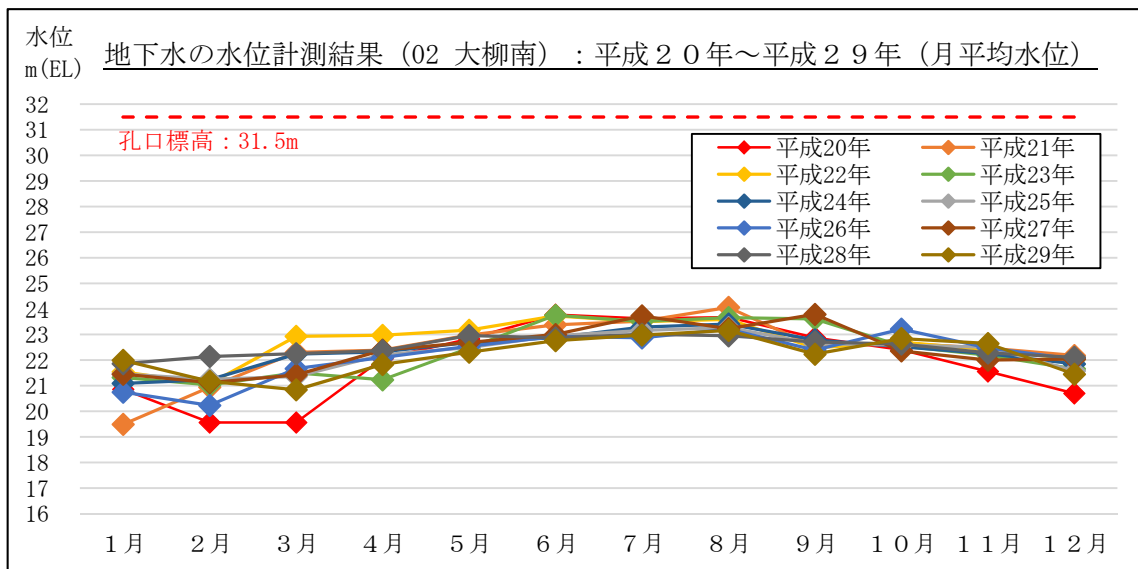
図 2-16 地下水の水位計測結果 (月平均水位) : 02 大柳南 (島田市大柳)
