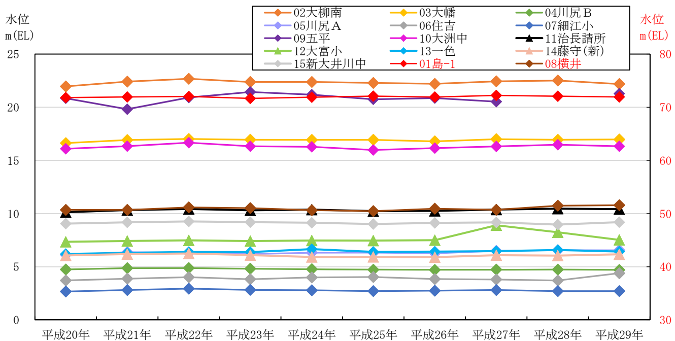
図 2-14 地下水の水位計測結果 (年平均水位)
