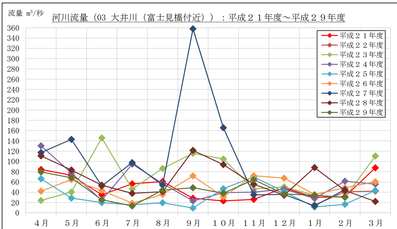
図 2-11 流量計測結果 : 03 大井川 (富士見橋 ふじみ 付近)
