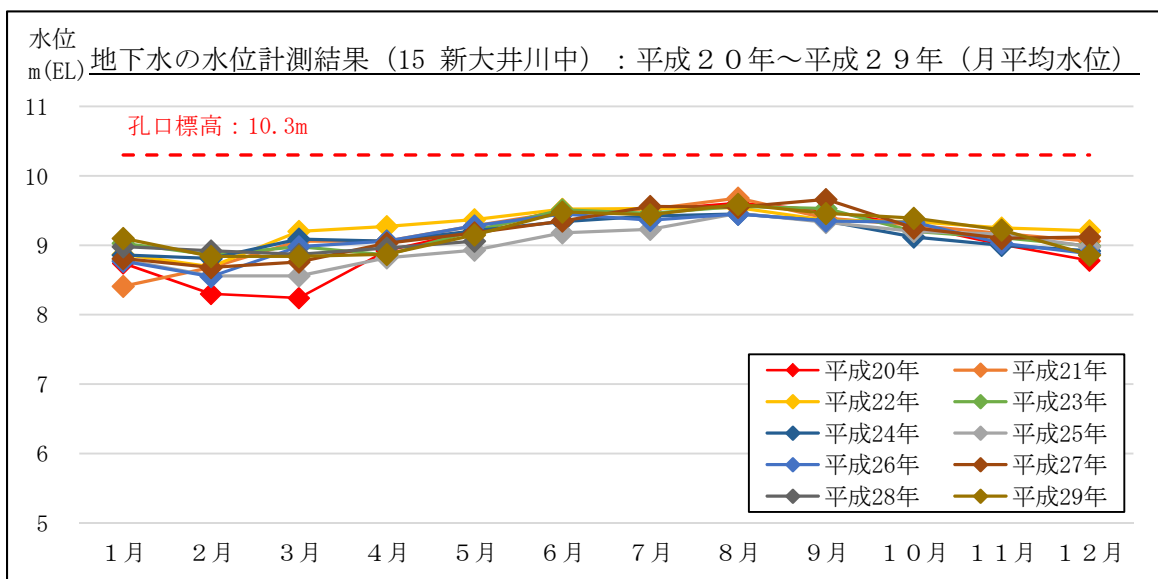
図 2-29 地下水の水位計測結果 (月平均水位) : 15 新大井川中 (焼津市下江留)
