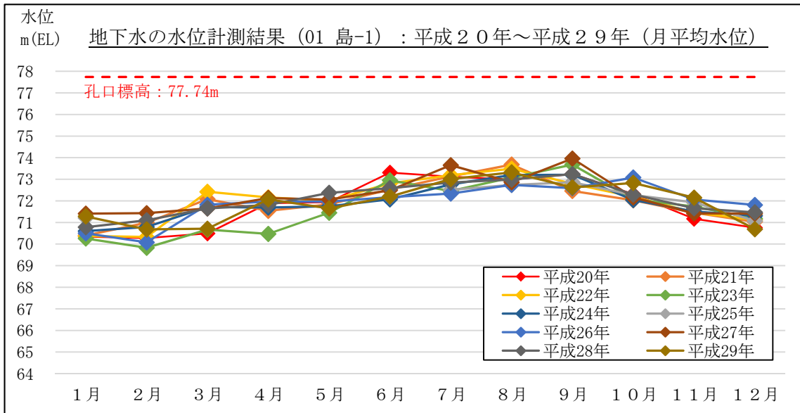
図 2-15 地下水の水位計測結果 (月平均水位) : 01 島-1 (島田市島)
