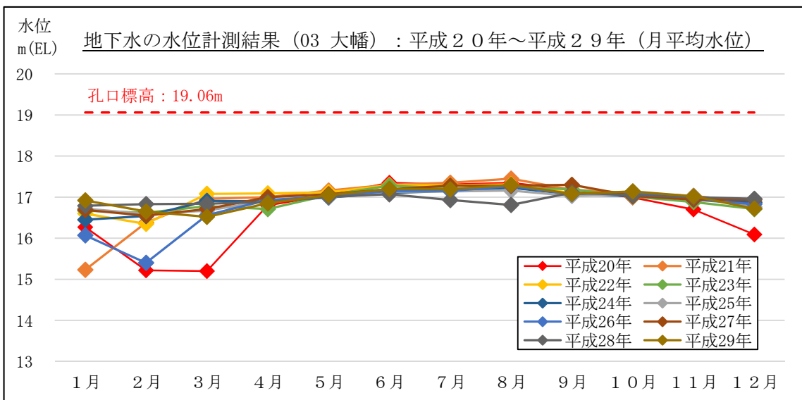
図 2-17 地下水の水位計測結果 (月平均水位) : 03 大幡 (吉田町大幡)
