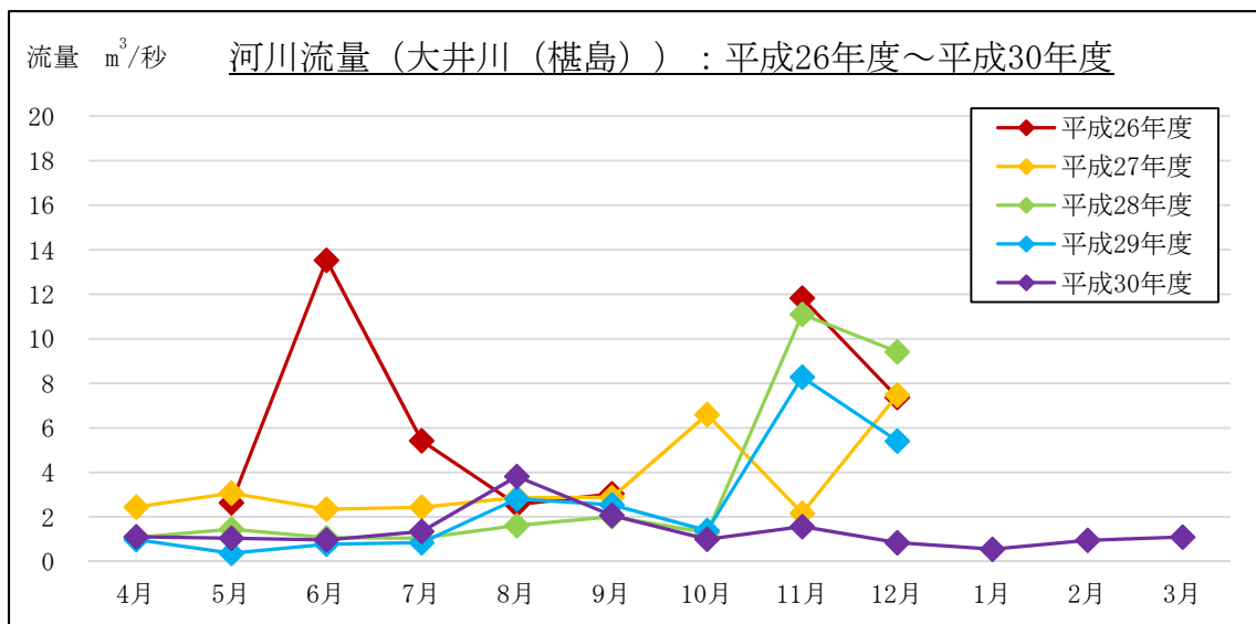
図 2-6 流量計測結果（月1回計測：榎島）
