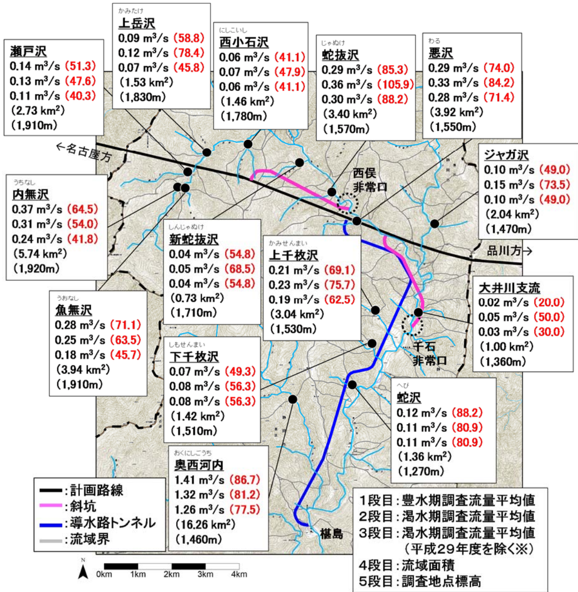
図 2-7 上流域の沢等の流量（年2回計測）調査結果
