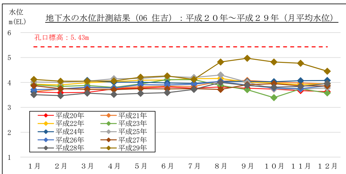
図 2-20 地下水の水位計測結果 (月平均水位) : 06 住吉 (吉田町住吉)
