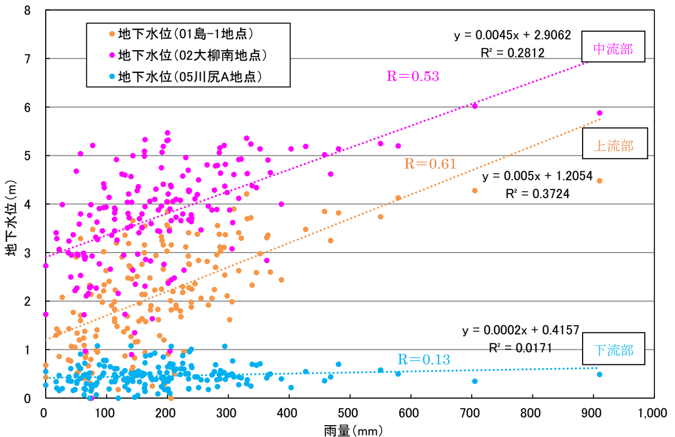
図 2.23 (2) 地下水位と島田観測所雨量の相関関係 (拡大図)
