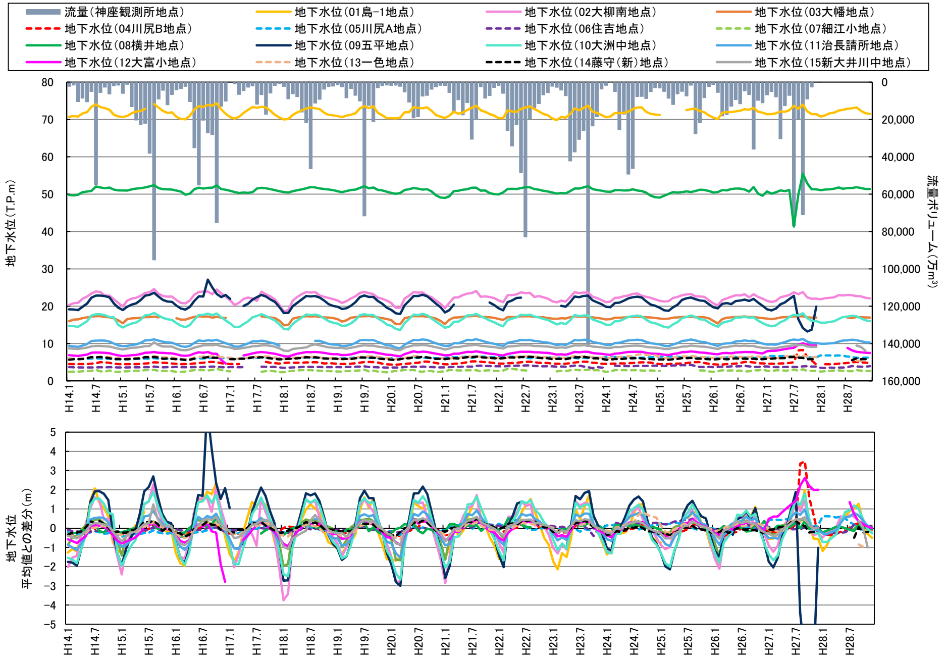
図 2.24 地下水位と神座地点流量の経年変化 (H14～H28)
