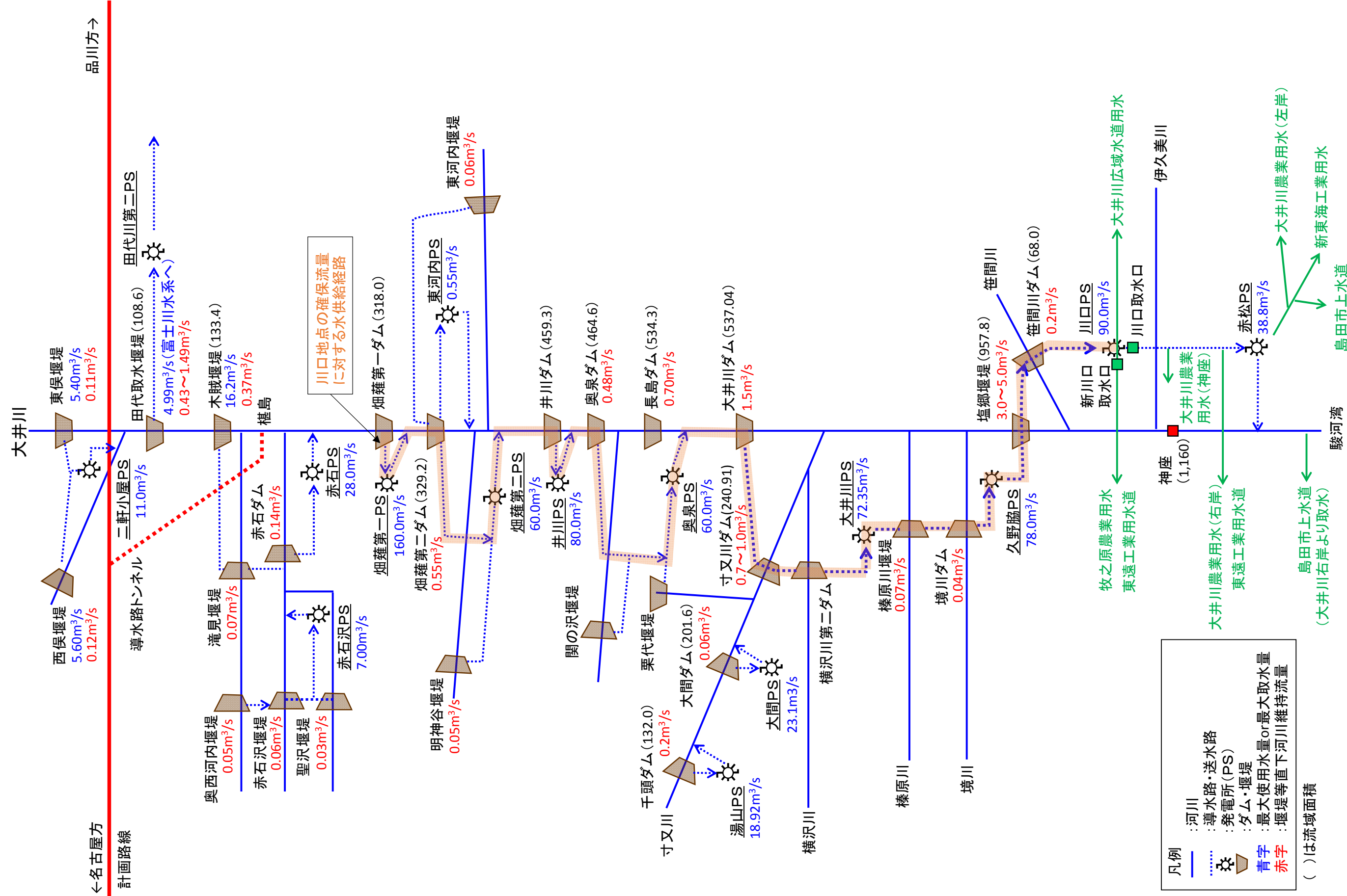
図 2.10 大井川水利模式図
