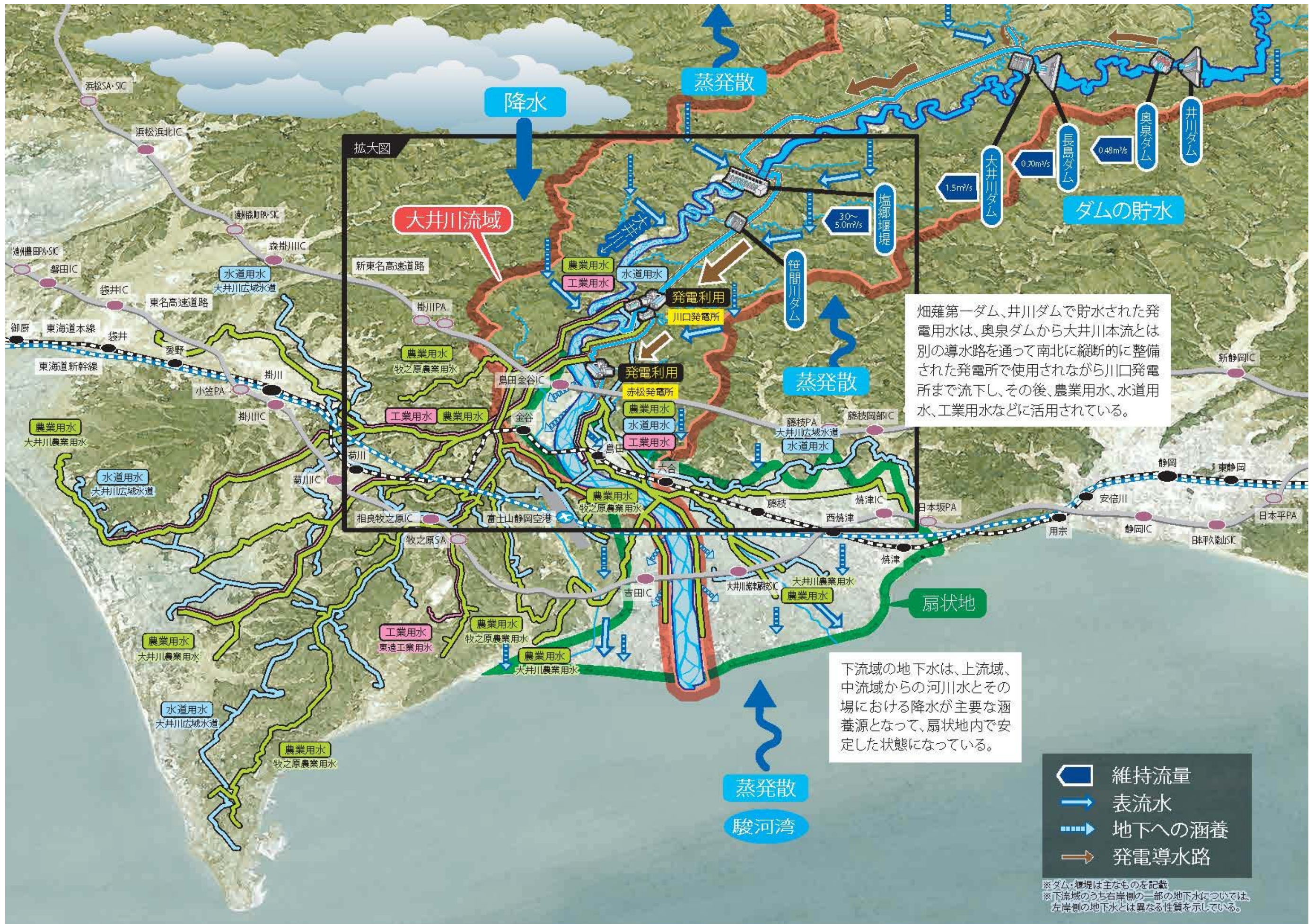
図 2.34 大井川流域の水循環の概念図 <鳥瞰図・井川ダム下流側>
