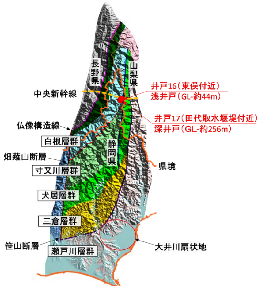
図 2.28 大井川流域の地層分布と上流域（榎島以北）の観測井の位置図
