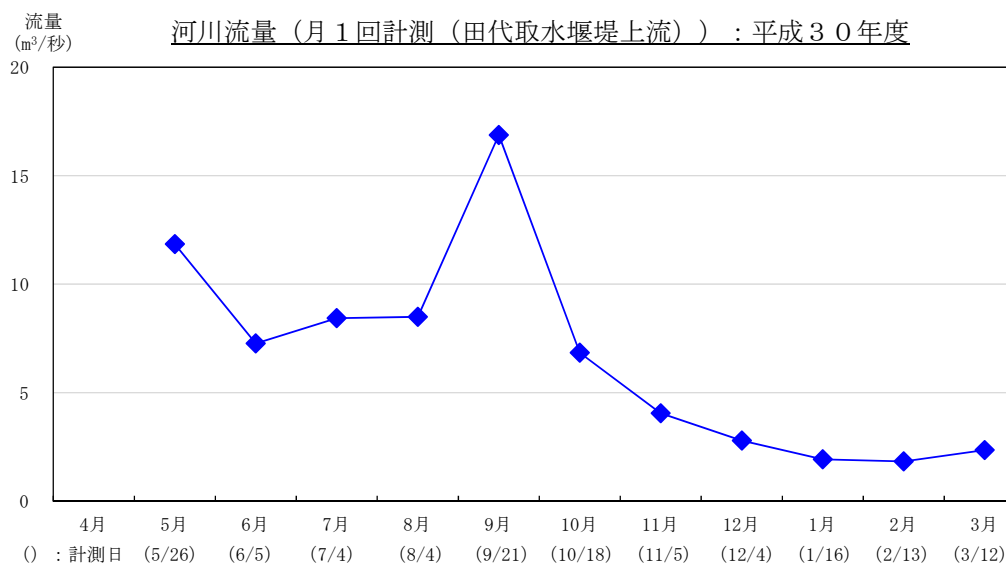
図 2-12 上流域の地下水位、河川流量調査結果（田代付近、平成30年度）
