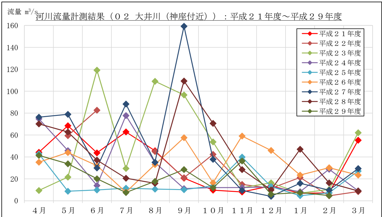
図 2-10 流量計測結果 : 02 大井川 (神座付近)
