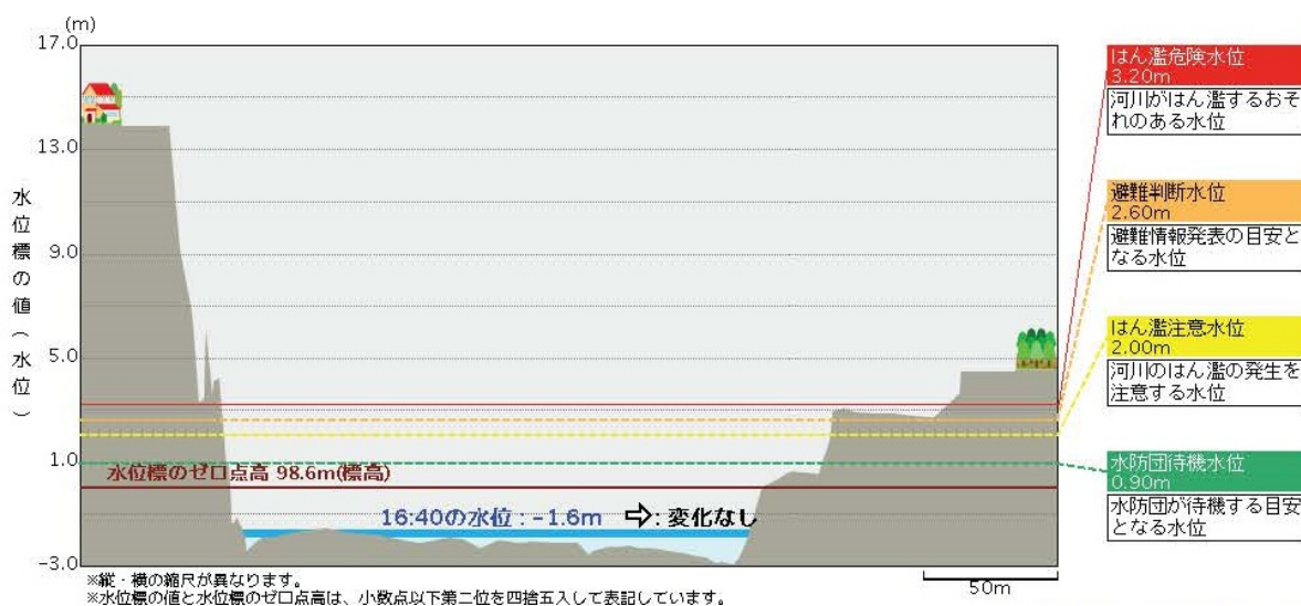
図 2-2 大井川（神座地点）の断面図
