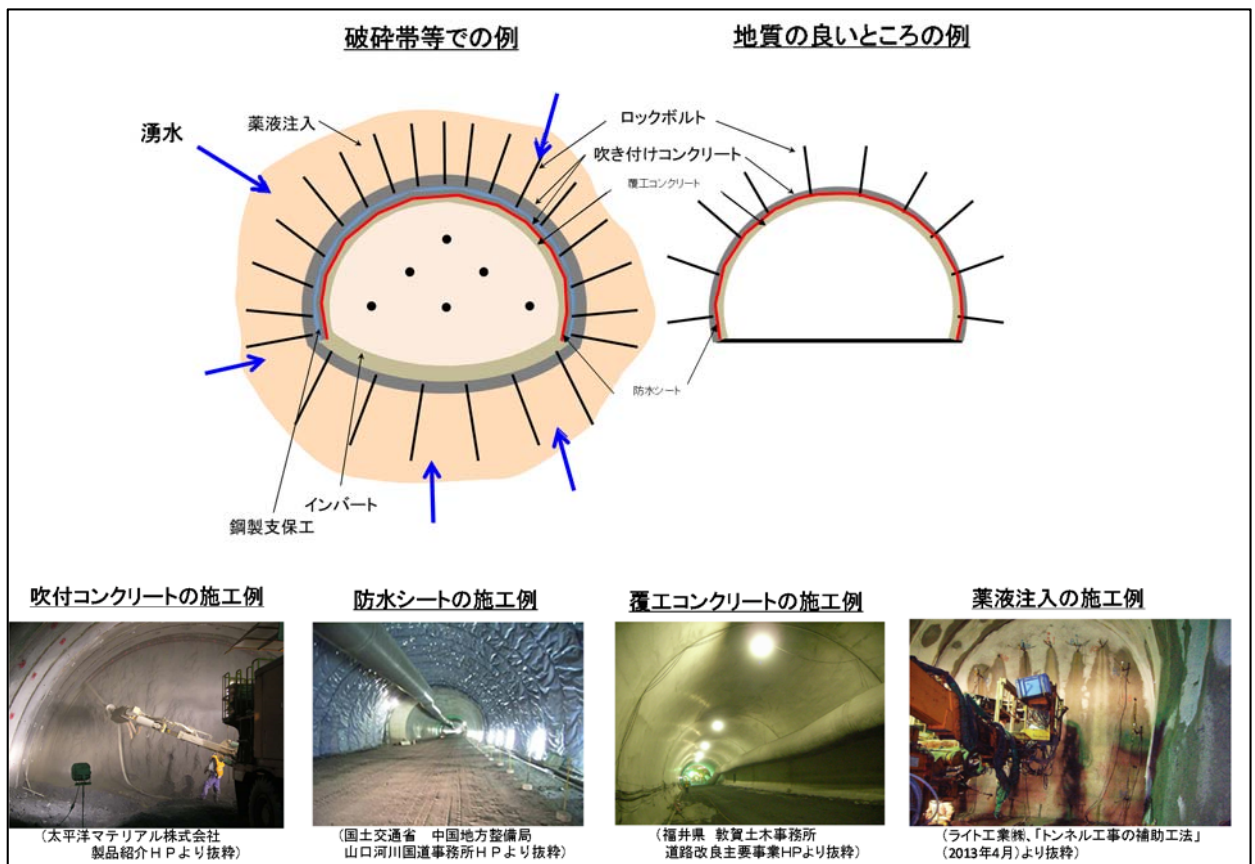
図 5.5 本坑におけるトンネル湧水量低減対策
