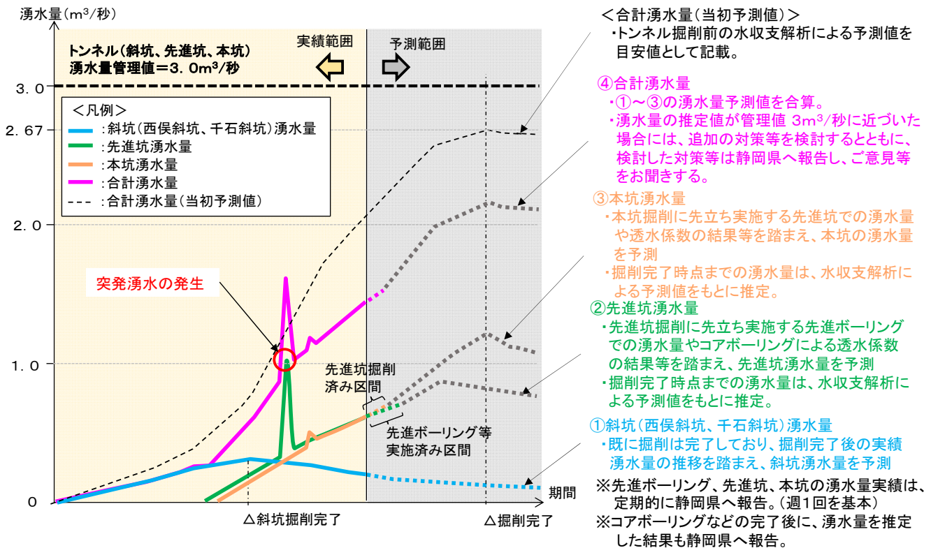
図 5.3 湧水量の管理曲線 (イメージ)
