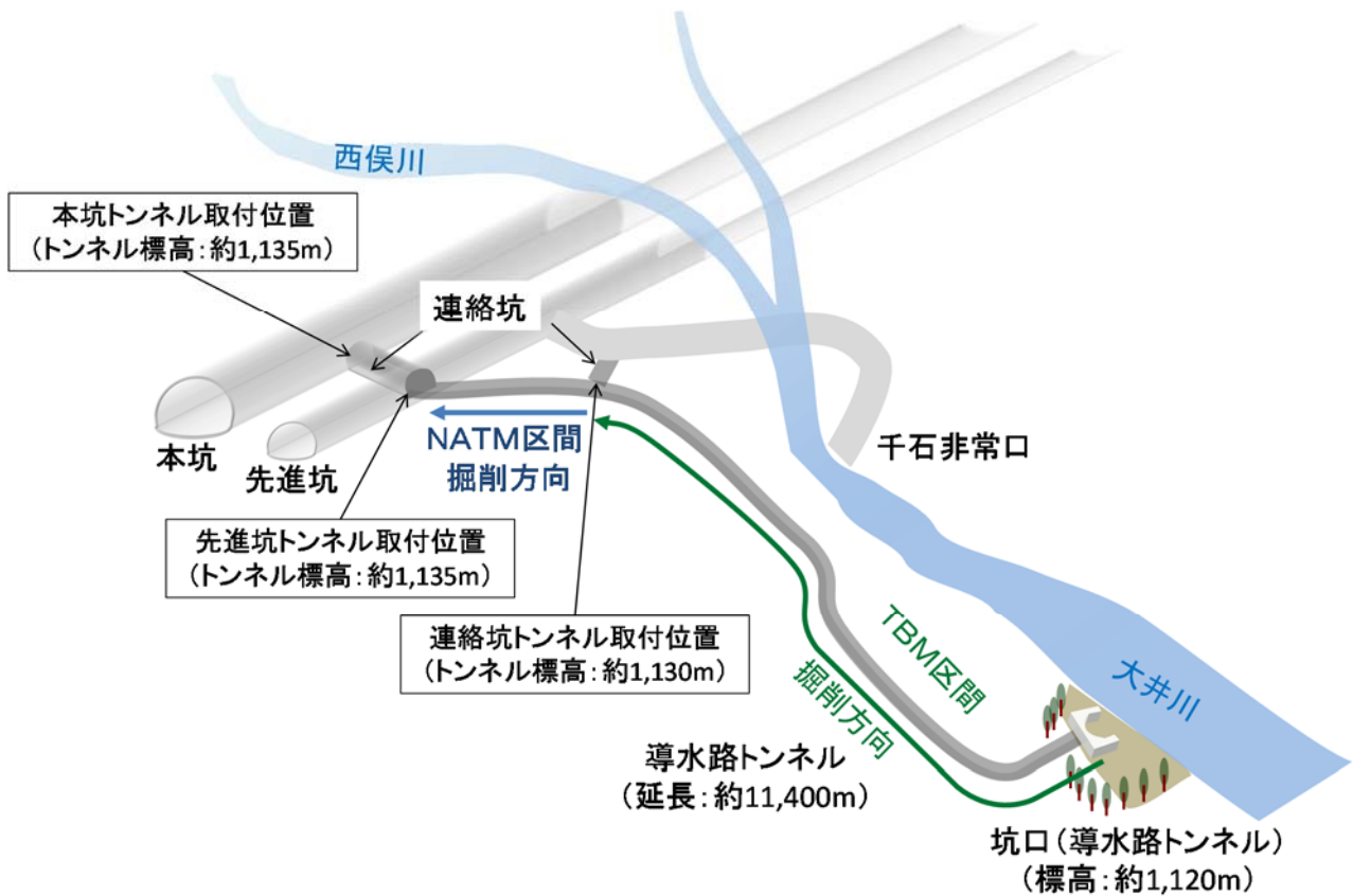
図 5.14 導水路トンネル 概念図
