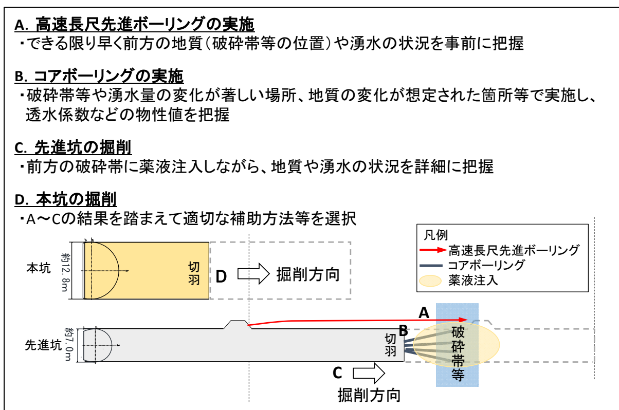
図 5.1 先進ボーリングを用いたトンネル掘削の手順
