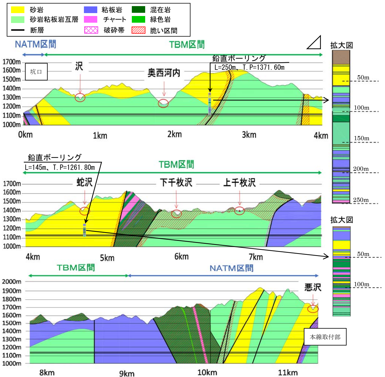
図 5.16 導水路トンネル 縦断図
