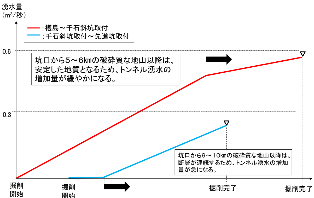
図 5.18 予測値から作成した導水路トンネルの湧水量の推移
