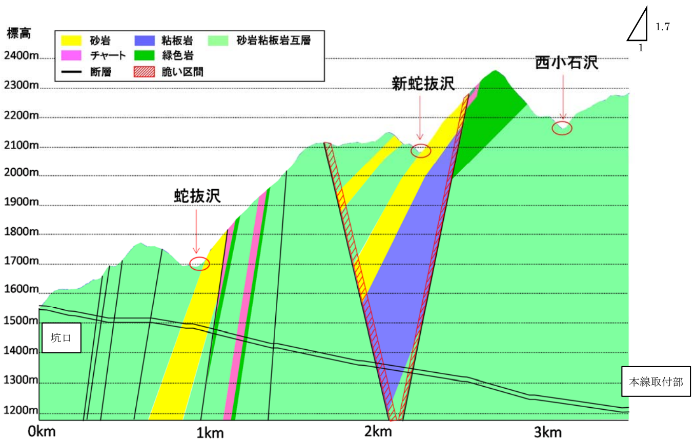
図 5.12 西俣斜坑 縦断図
