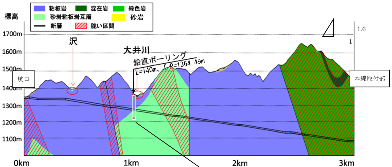
図 5.8 千石斜坑 縦断面図 拡大図
