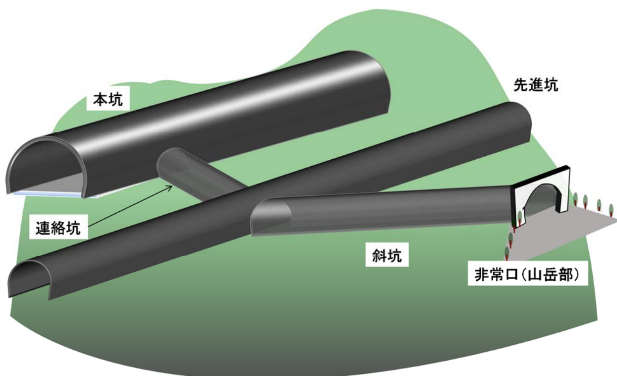
図 5. 2 0 本坑、先進坑、斜坑の位置関係
