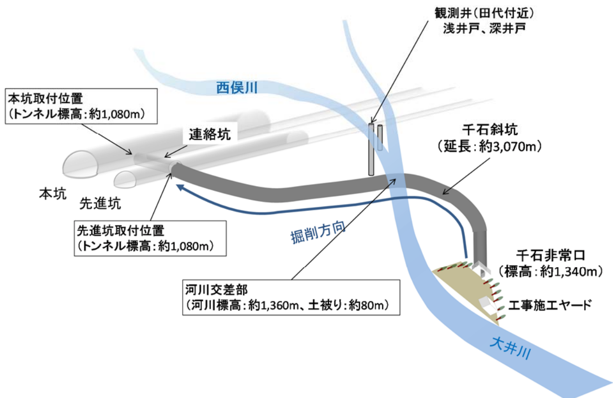
図 5.6 千石斜坑 概念図
