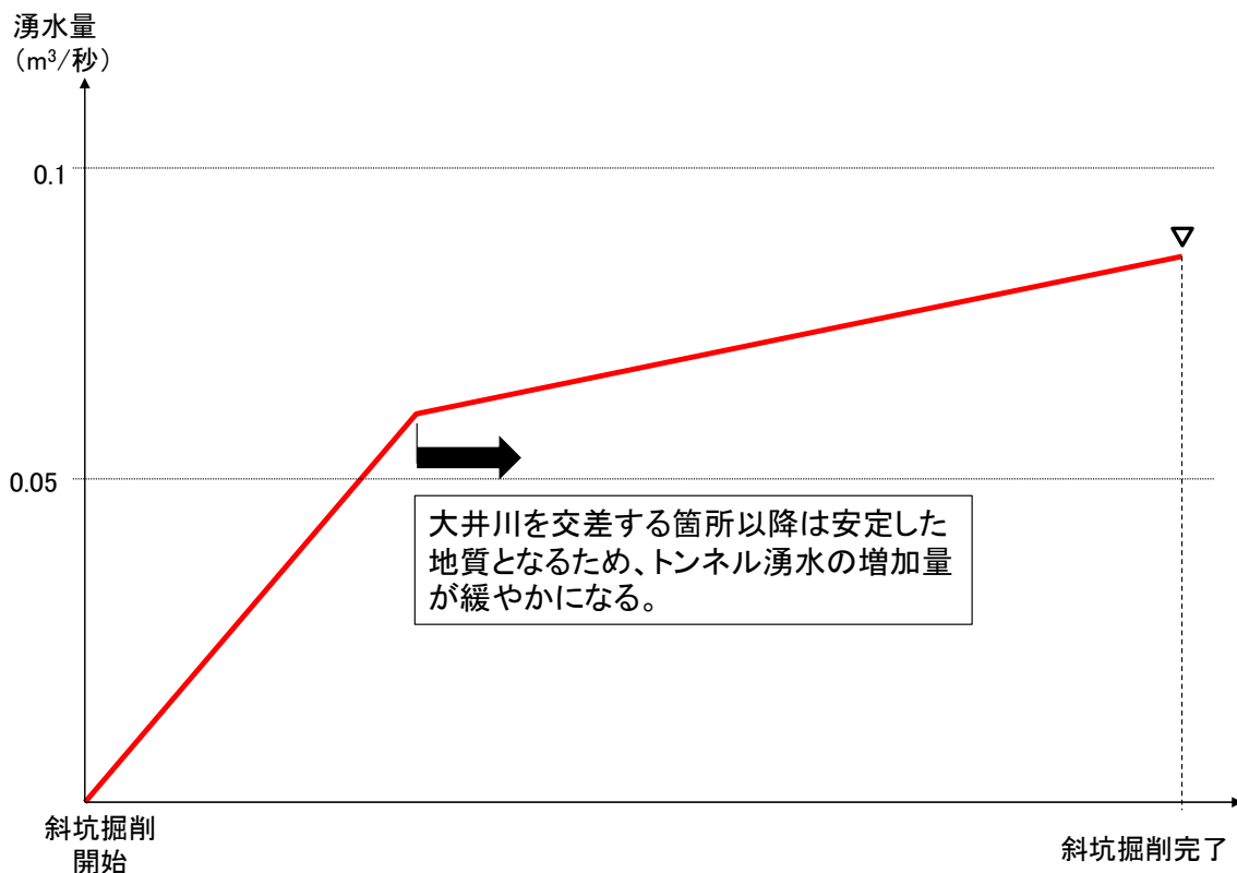
図 5.9 予測値から作成した千石斜坑の湧水量の推移
