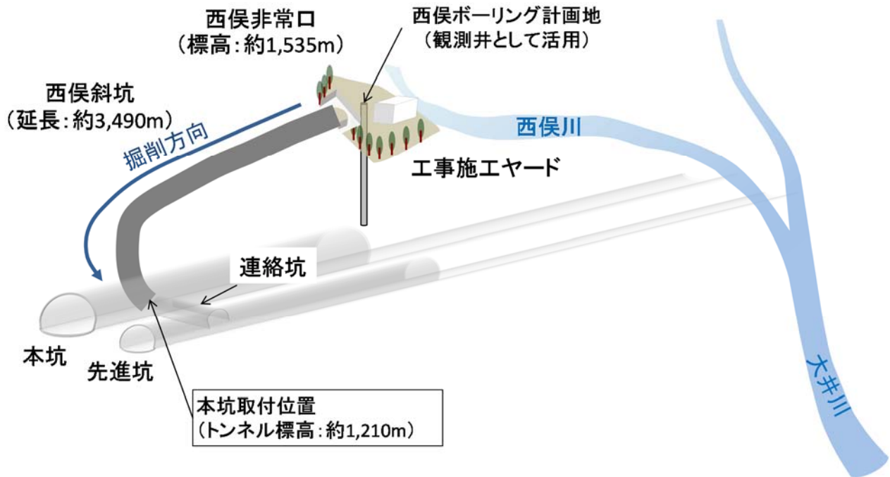
図 5.10 西俣斜坑 概念図
