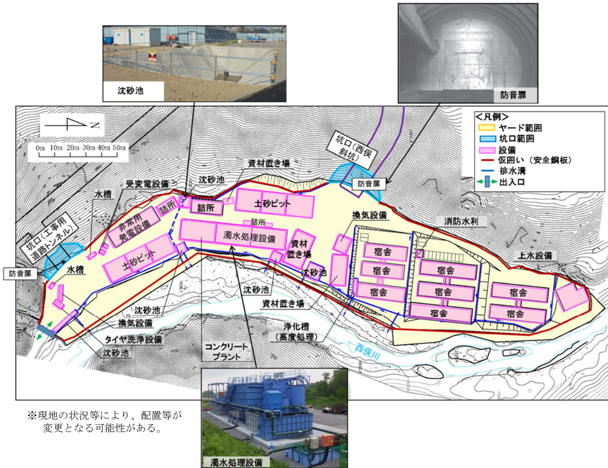
図 5.11 西俣斜坑ヤードの計画図
