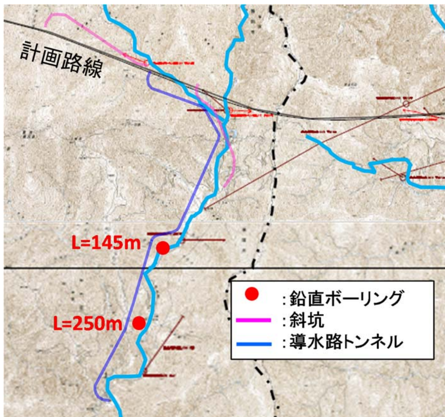
図 5.17 ボーリング調査平面図
