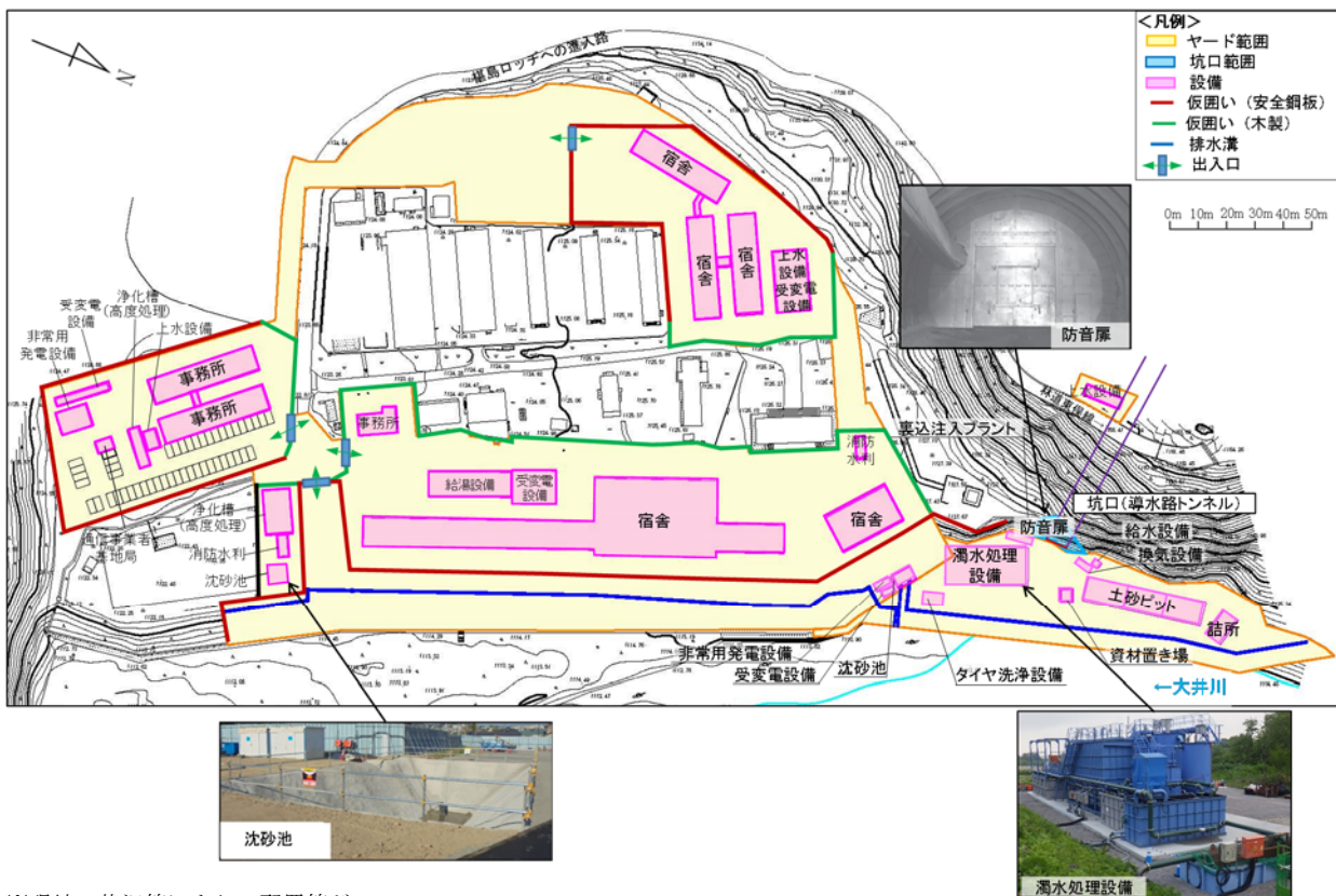
図 5.15 導水路トンネルヤードの計画図
