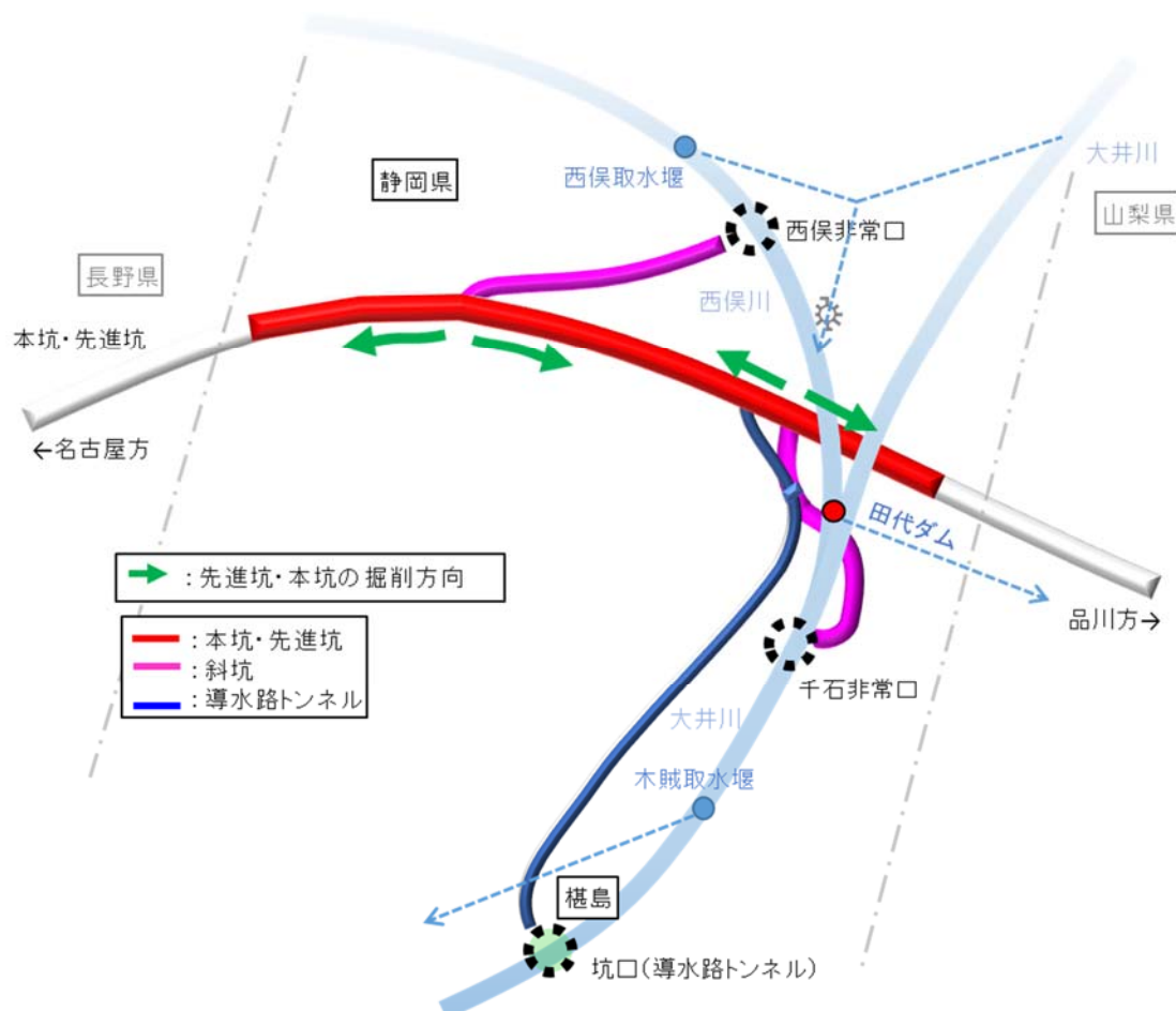
図 5. 19 本坑、先進坑、掘削方向図
