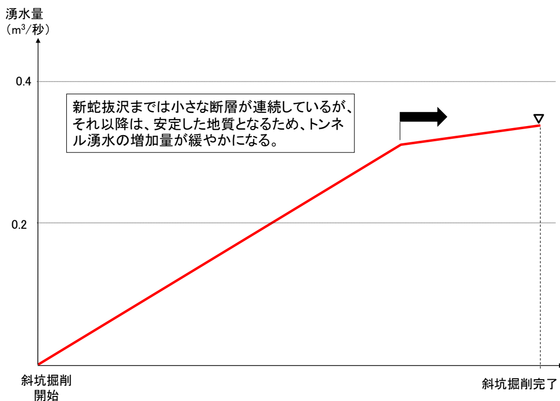
図 5.13 予測値から作成した西俣斜坑の湧水量の推移
