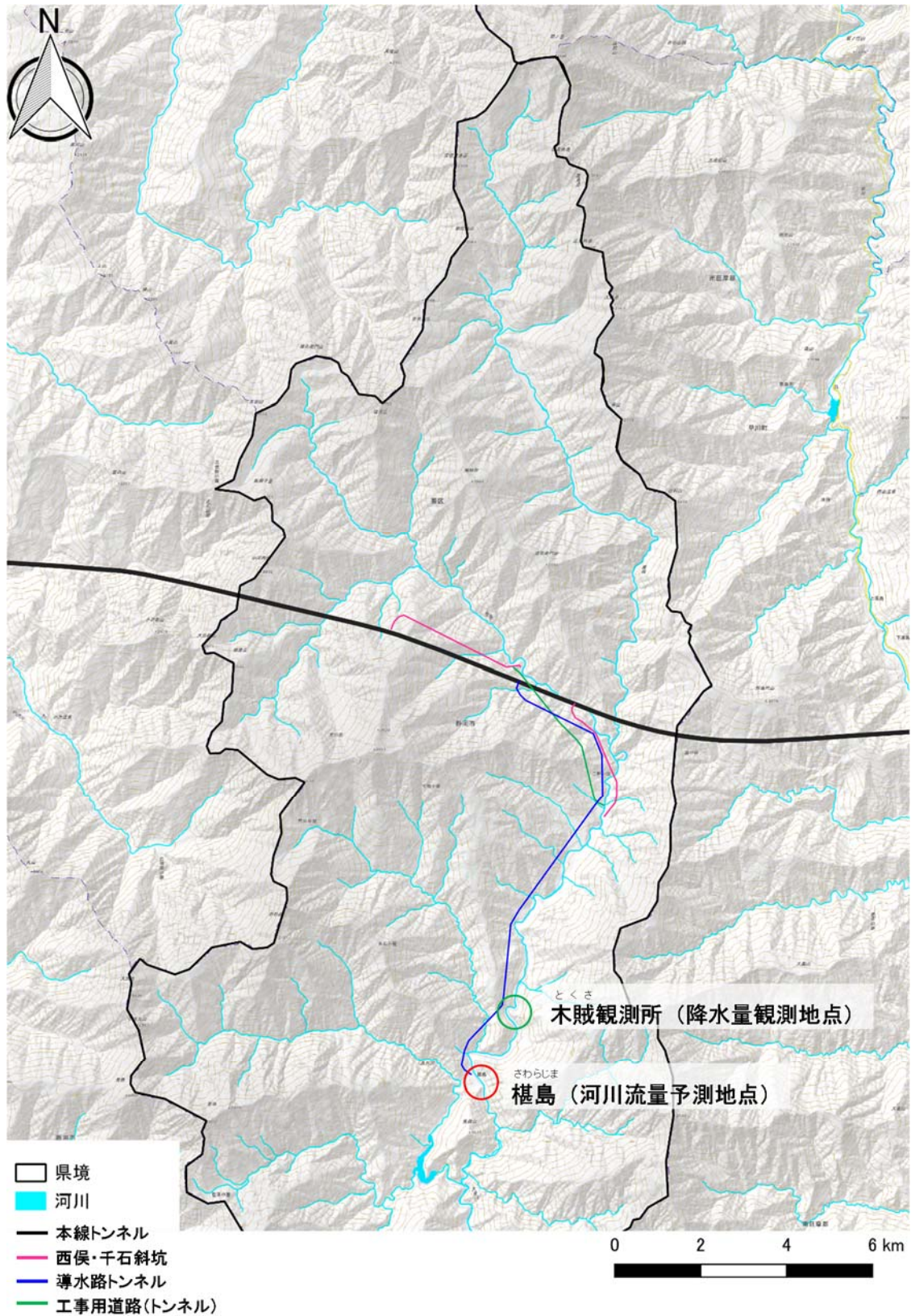
図 4.63 とくさ 木賊観測所(降水量観測地点)及び さわらじま 榎島(河川流量予測地点)の位置
