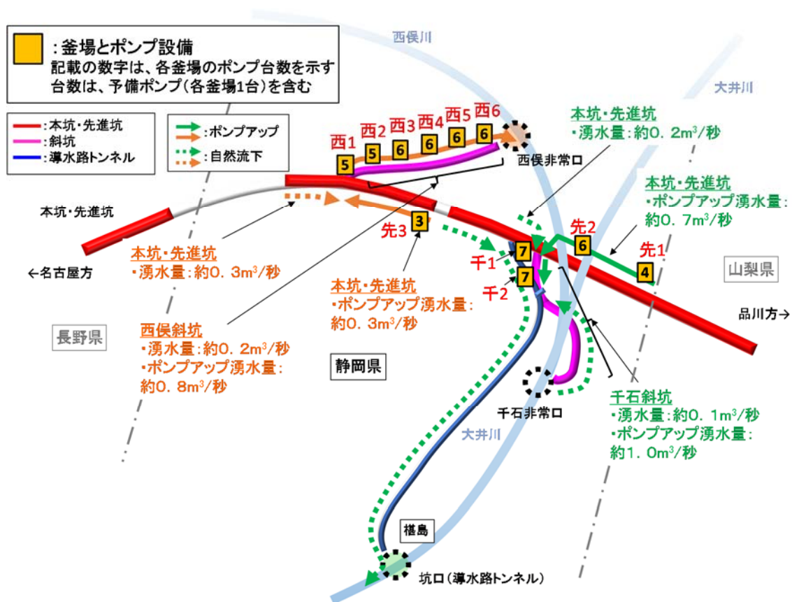
図 4.26 ポンプ配置図（西俣非常口～導水路トンネル間の貫通直前）
