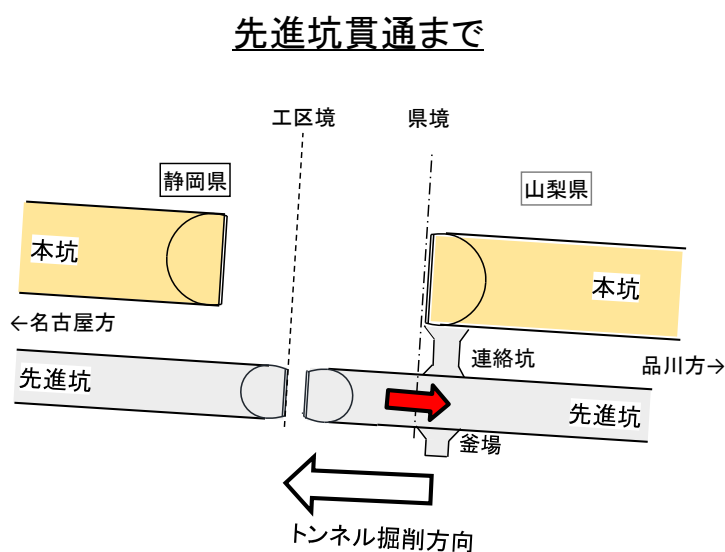
図 4.61 山梨県側へ流出する湧水（イメージ）
