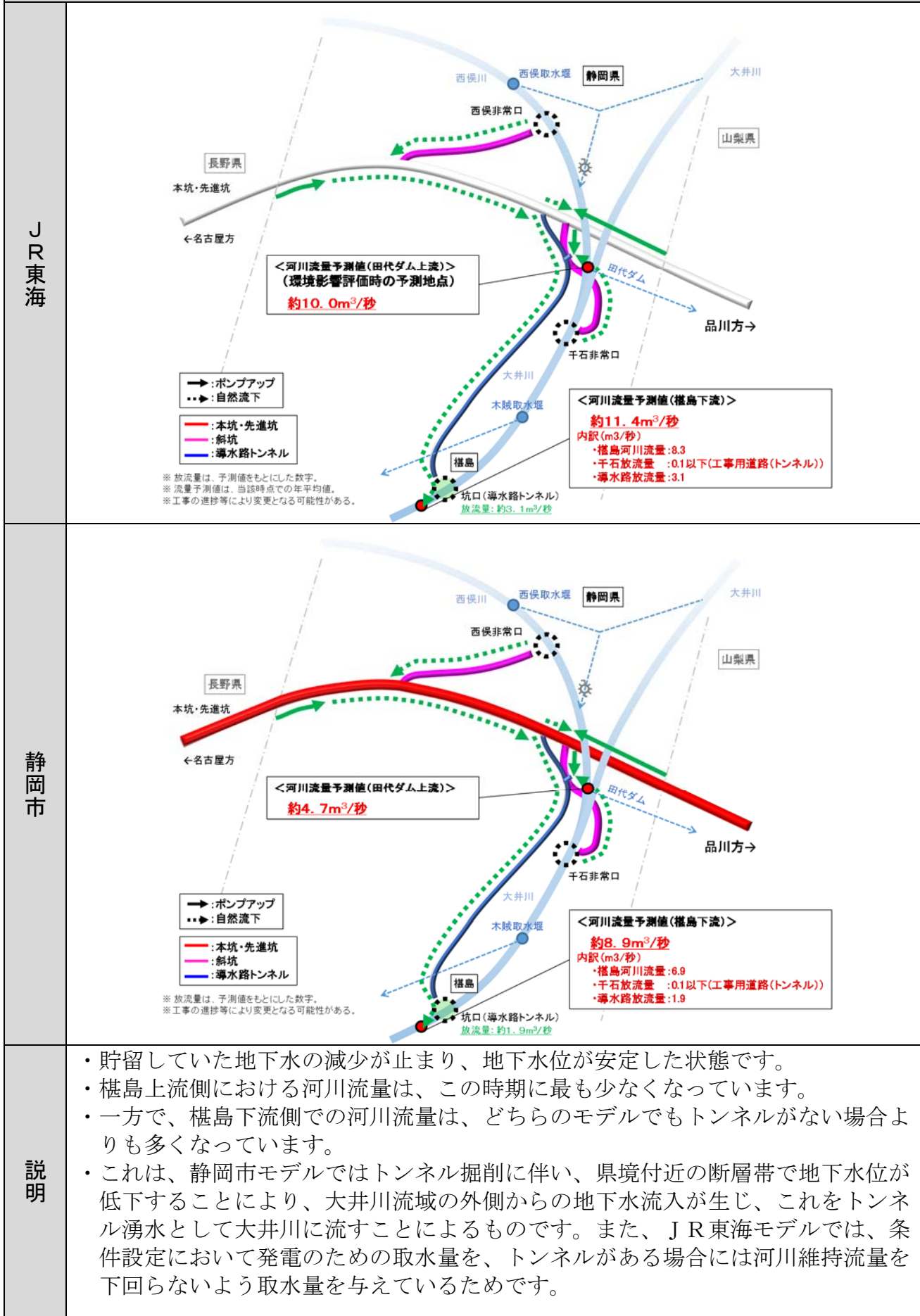
図 4.18 トンネル掘削完了後恒常時の予測結果
