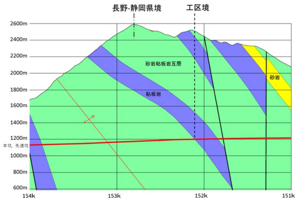
図 4.68 長野県境付近の地質縦断図
