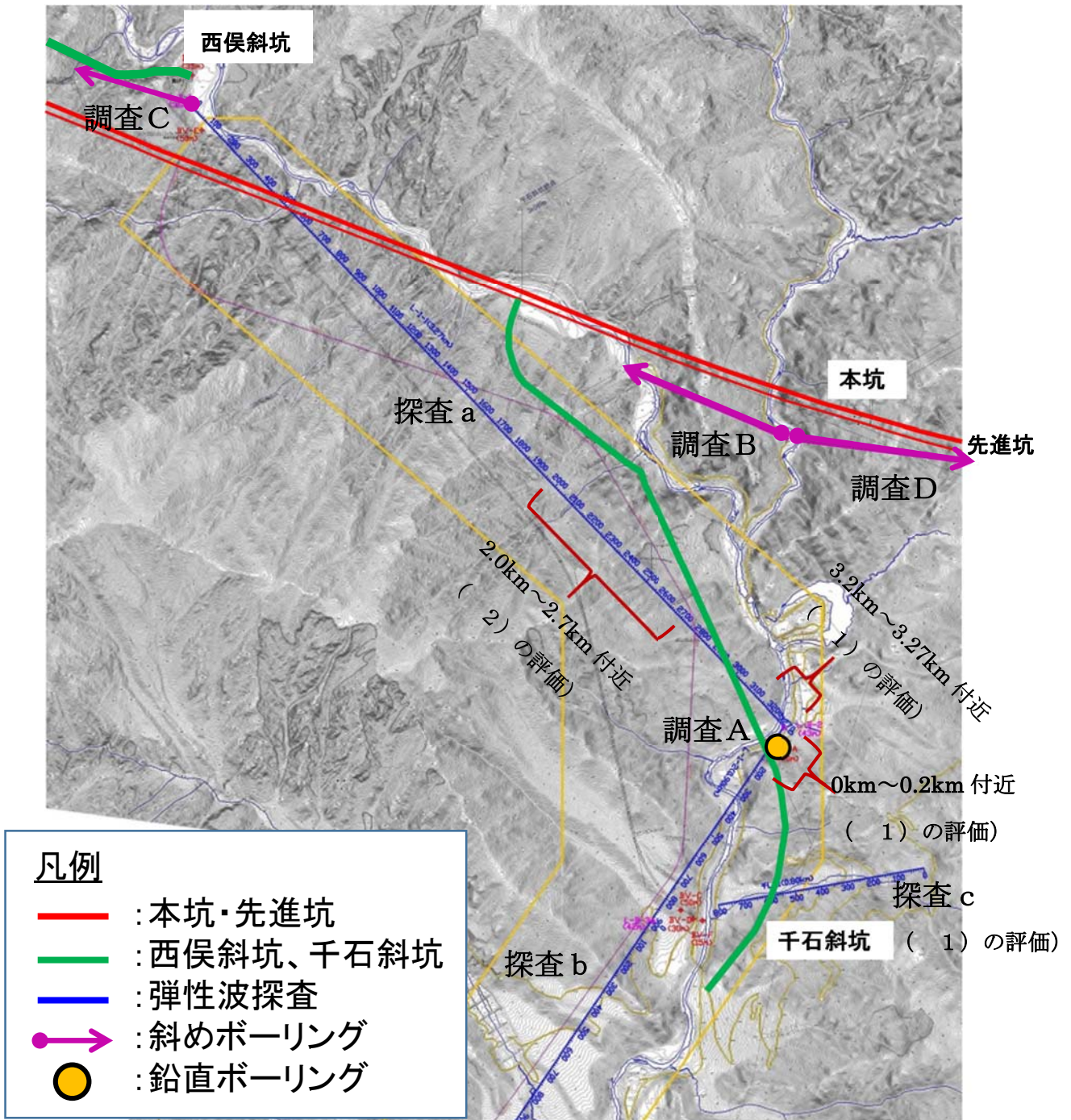
図 4.66 地質調査位置図
