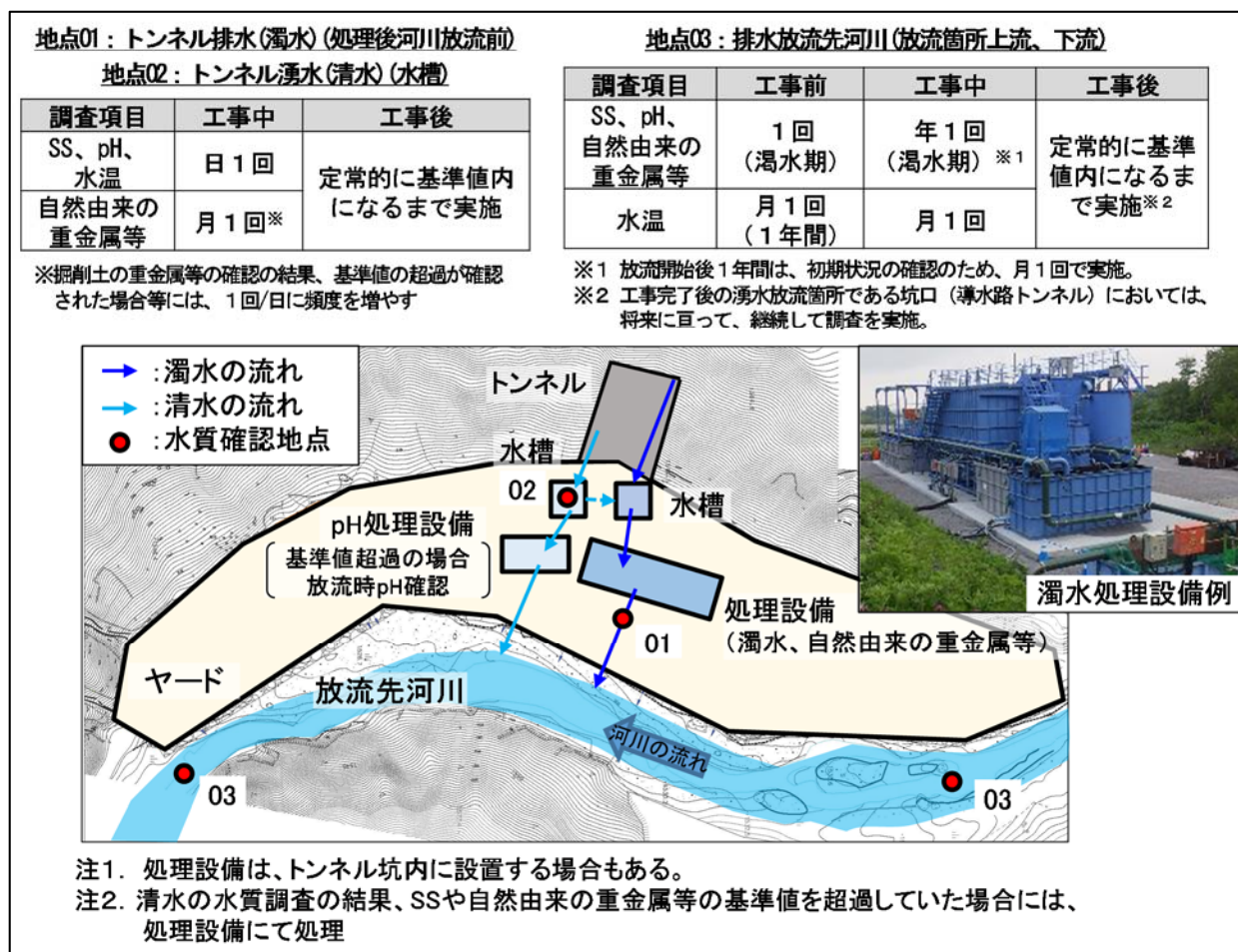
図 4.34 施工ヤードにおけるトンネル湧水等の処理の流れ（イメージ）
