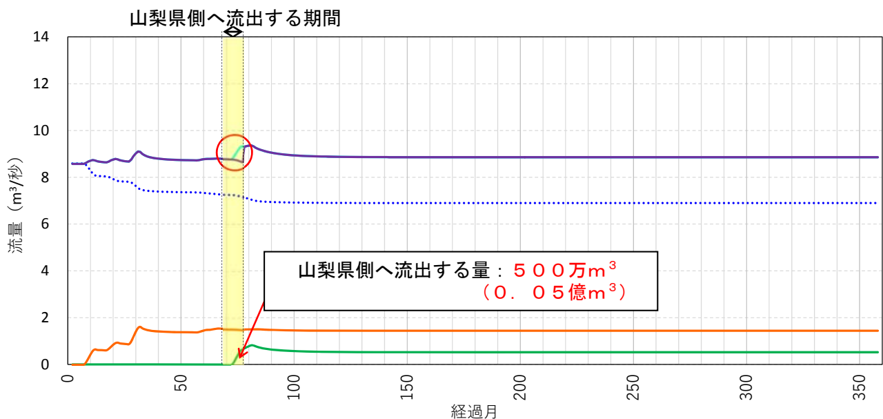
図 4.62 トンネル湧水が山梨県側へ流出しなかったと想定した場合の予測結果（静岡市モデル）
