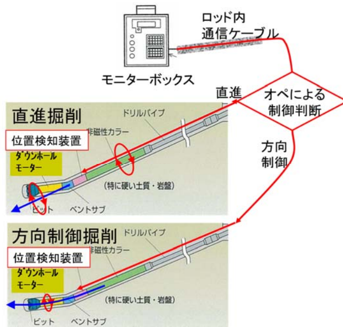
図 4.50 コントロールボーリングの方向制御イメージ
