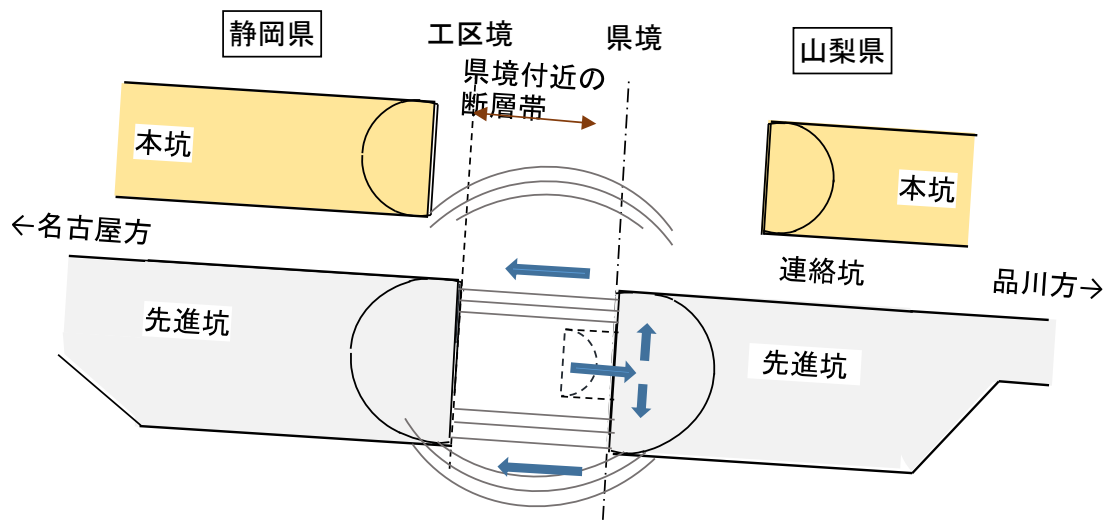
図 4.57 長尺ボーリングからの揚水検討図
