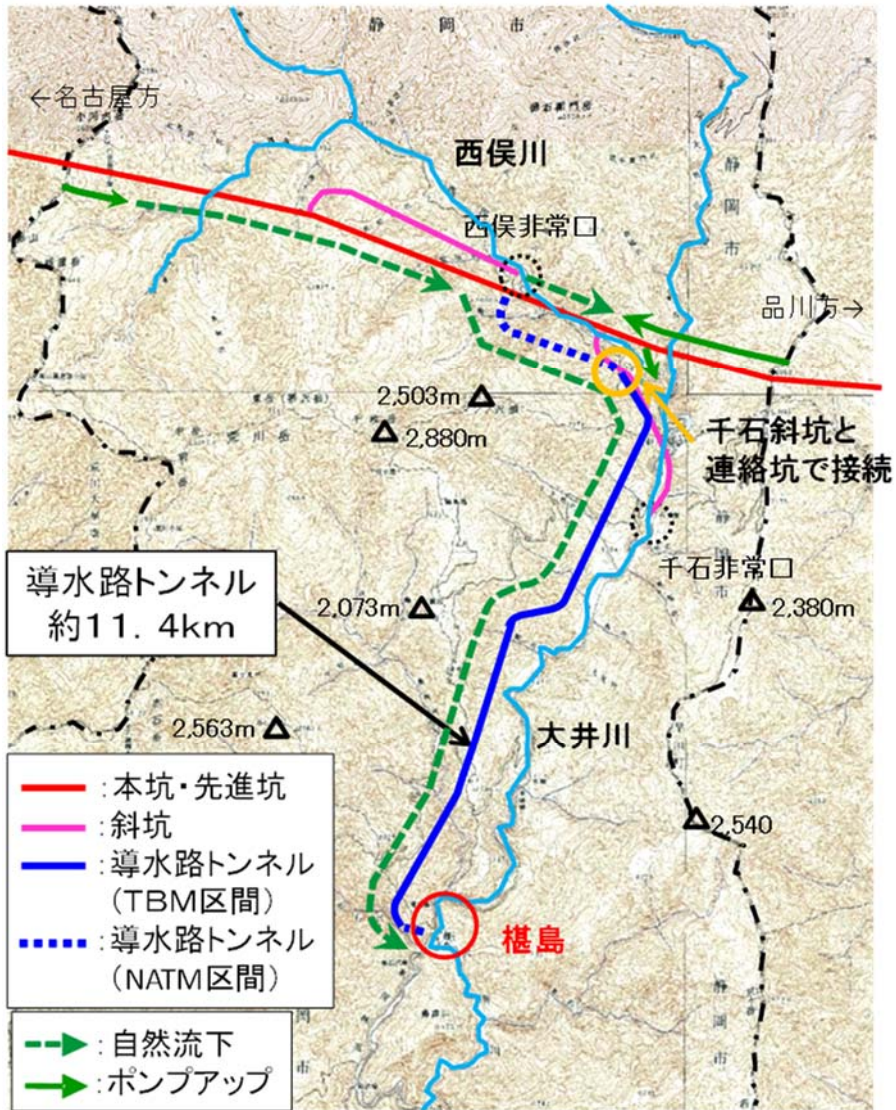
図 4.27 導水路トンネルの概要
