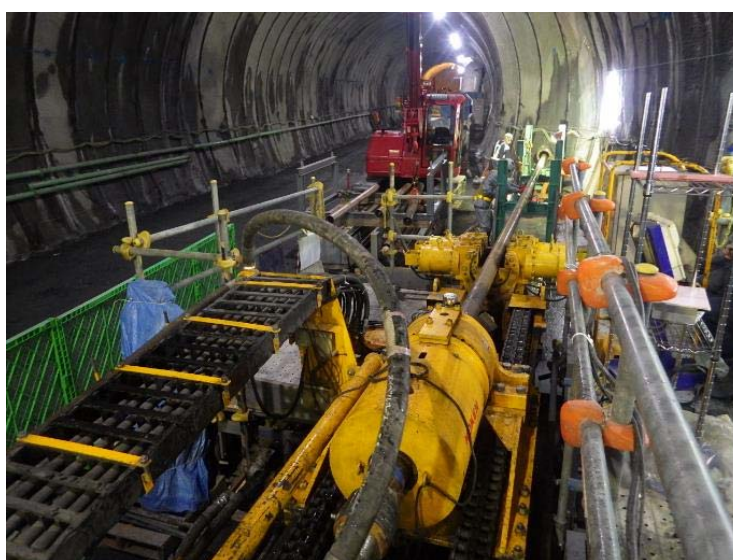
図 4.49 高速長尺先進ボーリング施工写真（山梨工区）
