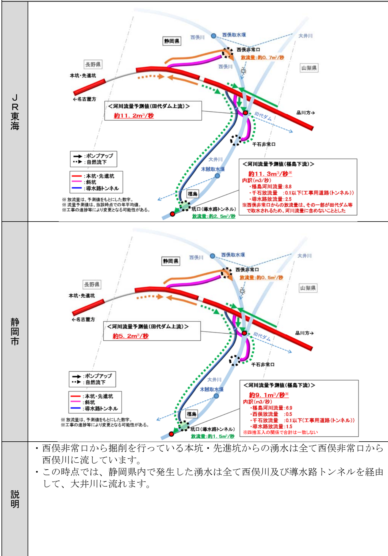
図 4.16 西俣非常口～導水路トンネル間が貫通する時期の予測結果
