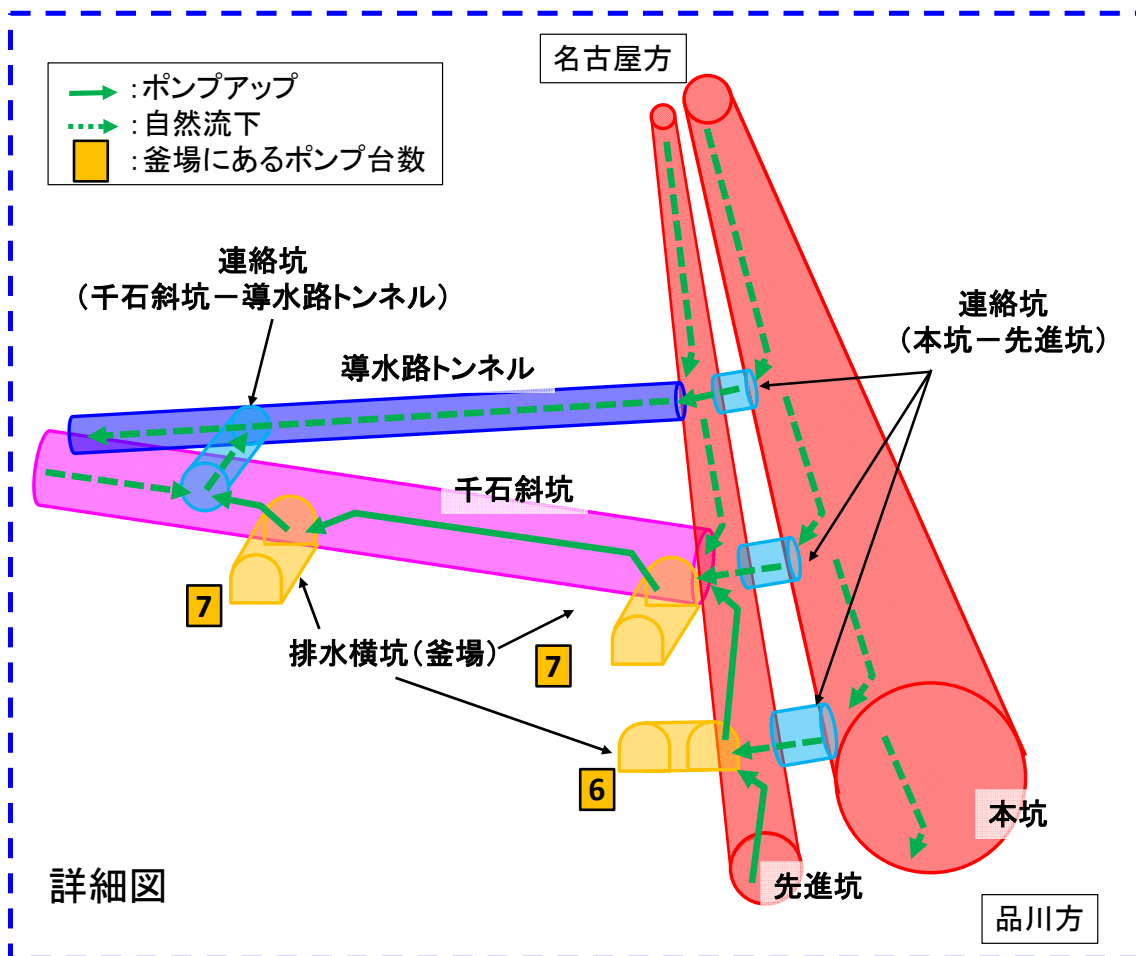
図 4.25 ポンプ配置図 (トンネル工事完了後)
