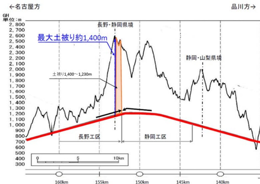
図 4.67 南アルプストンネル縦断面図
