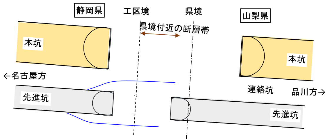
図 4.46 静岡県側先進坑からのポンプアップ
