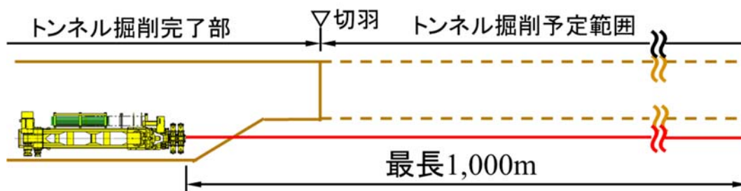
図 4.48 高速長尺先進ボーリング平面イメージ図
