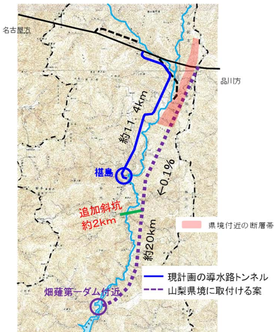
図 4.56 山梨県境付近へ導水路トンネルを取付ける計画
