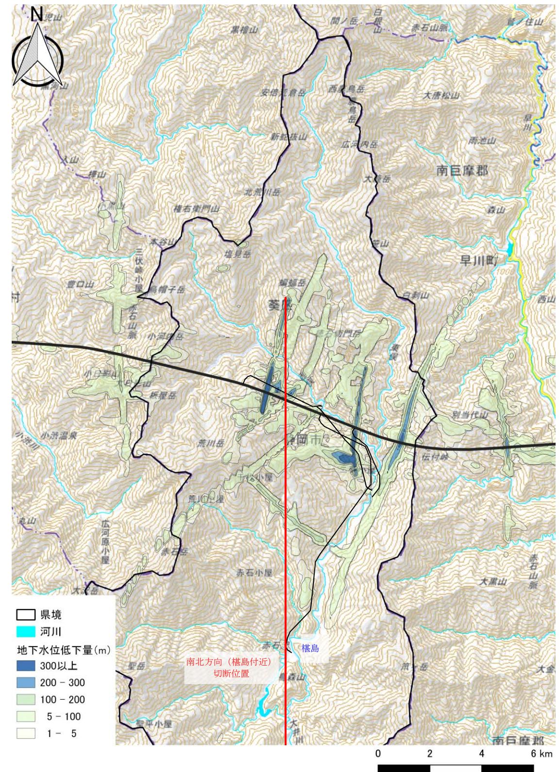
図 4.20 静岡市モデル 地下水位低下量平面図（トンネル掘削完了後の定常状態）
