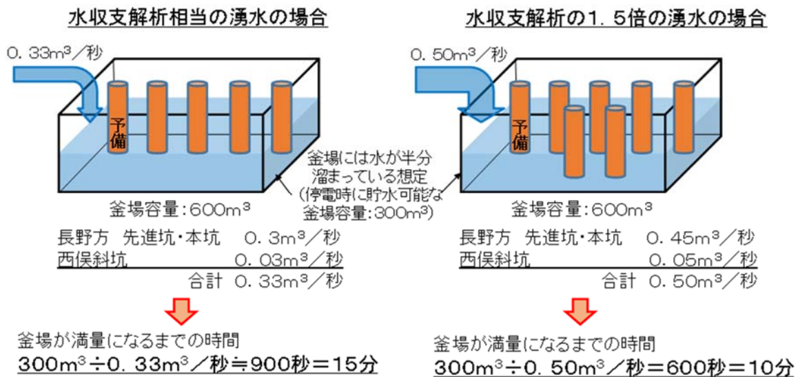
図 4.33 水収支解析より多い湧水が想定される場合（停電時）
