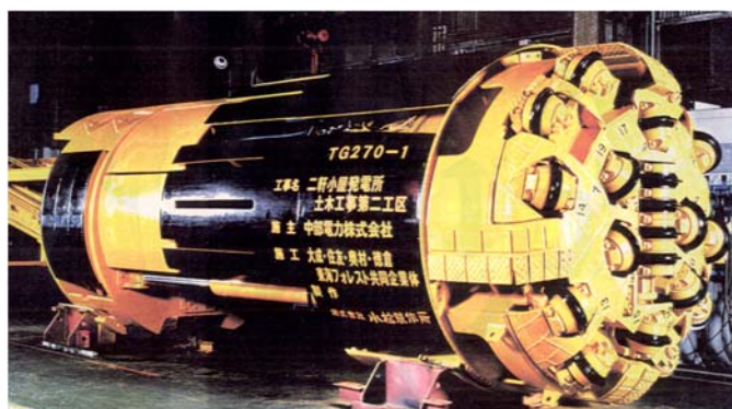
図 4.42 二軒小屋発電所のTBM (φ2.6m)
