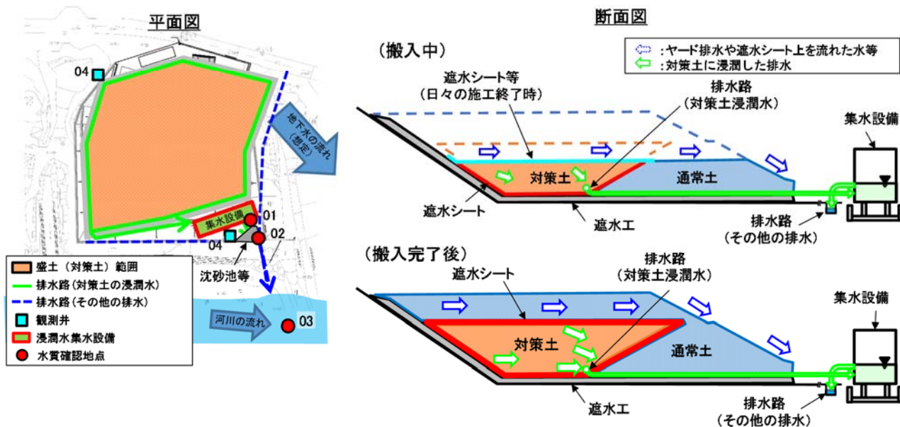
図 4.40 排水処理計画及び水質観測（イメージ）
