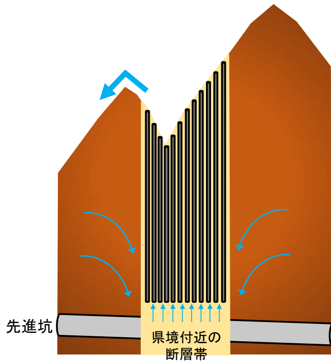
図 4.58 深井戸のイメージ
