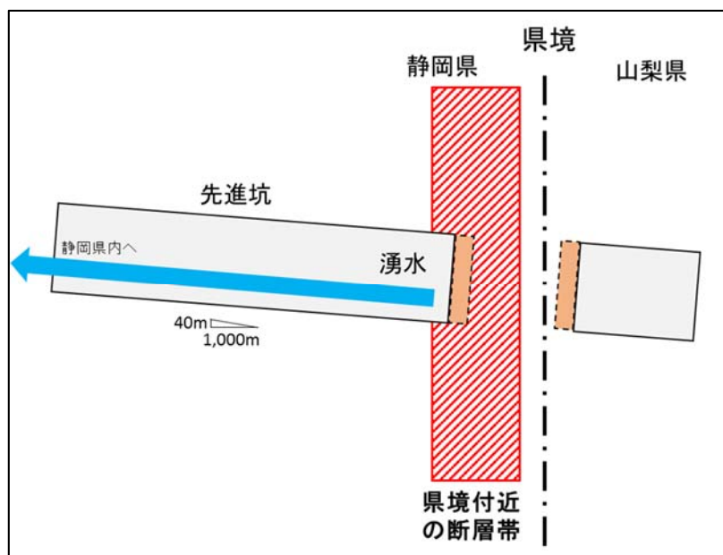
図 4.41 静岡県側からNATMで下向きに掘削する工法
