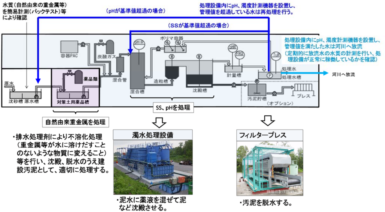
図 4.35 処理設備における処理のフロー (イメージ)
