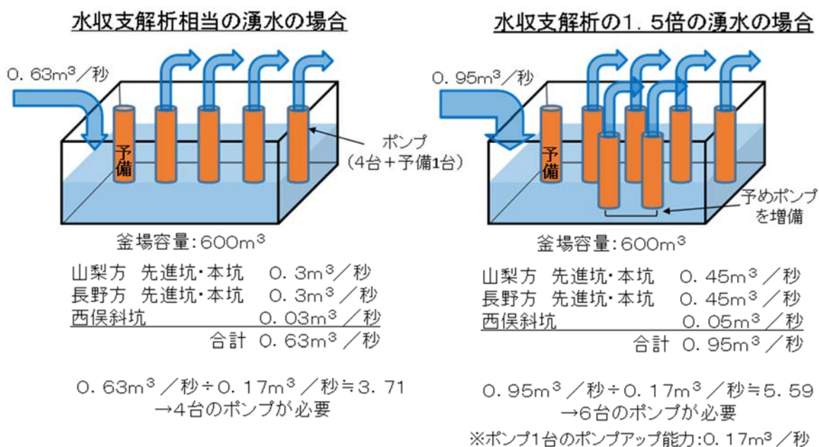
図 4.32 水収支解析より多い湧水が想定される場合
