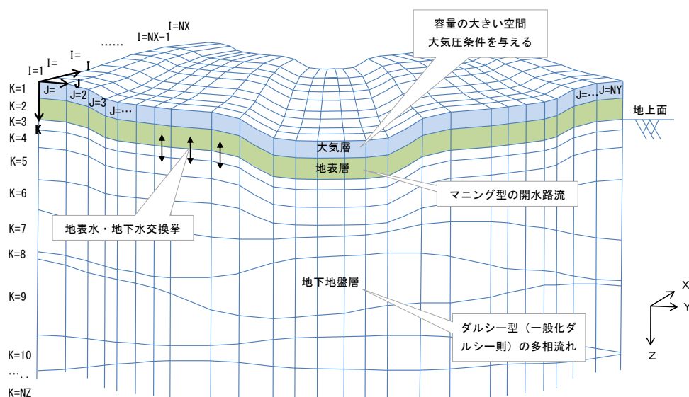
図 4.10 静岡市モデルのイメージ
