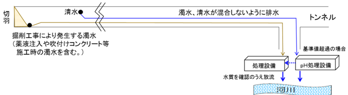
図 4.36 トンネル湧水の清濁分離 (イメージ)
