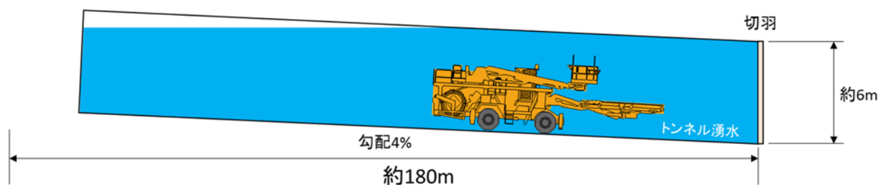
図 4.44 突発湧水発生1時間後のトンネル坑内の状況
