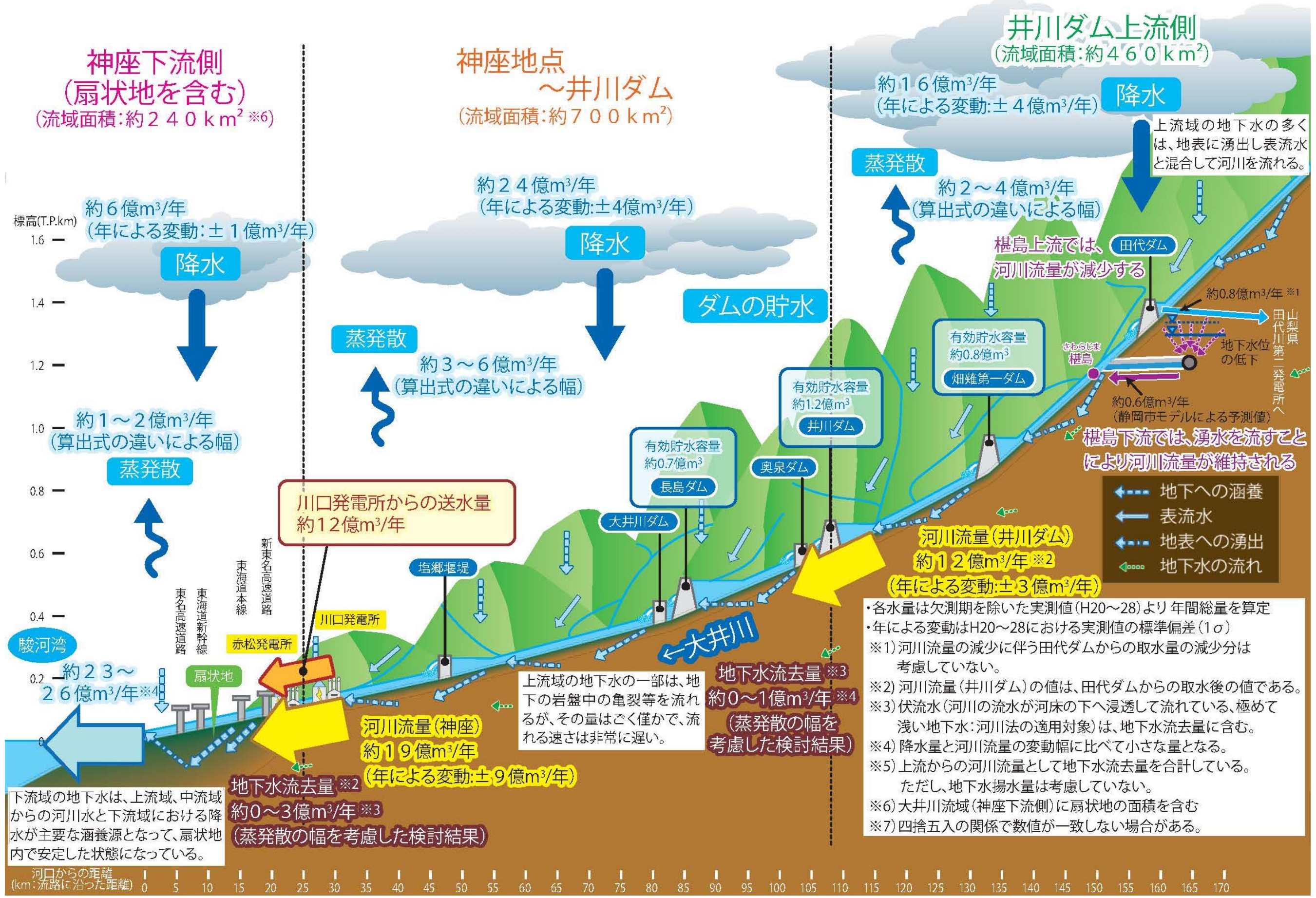
図 4.23 大井川流域の水循環の概念図 (掘削完了時の水循環量)
