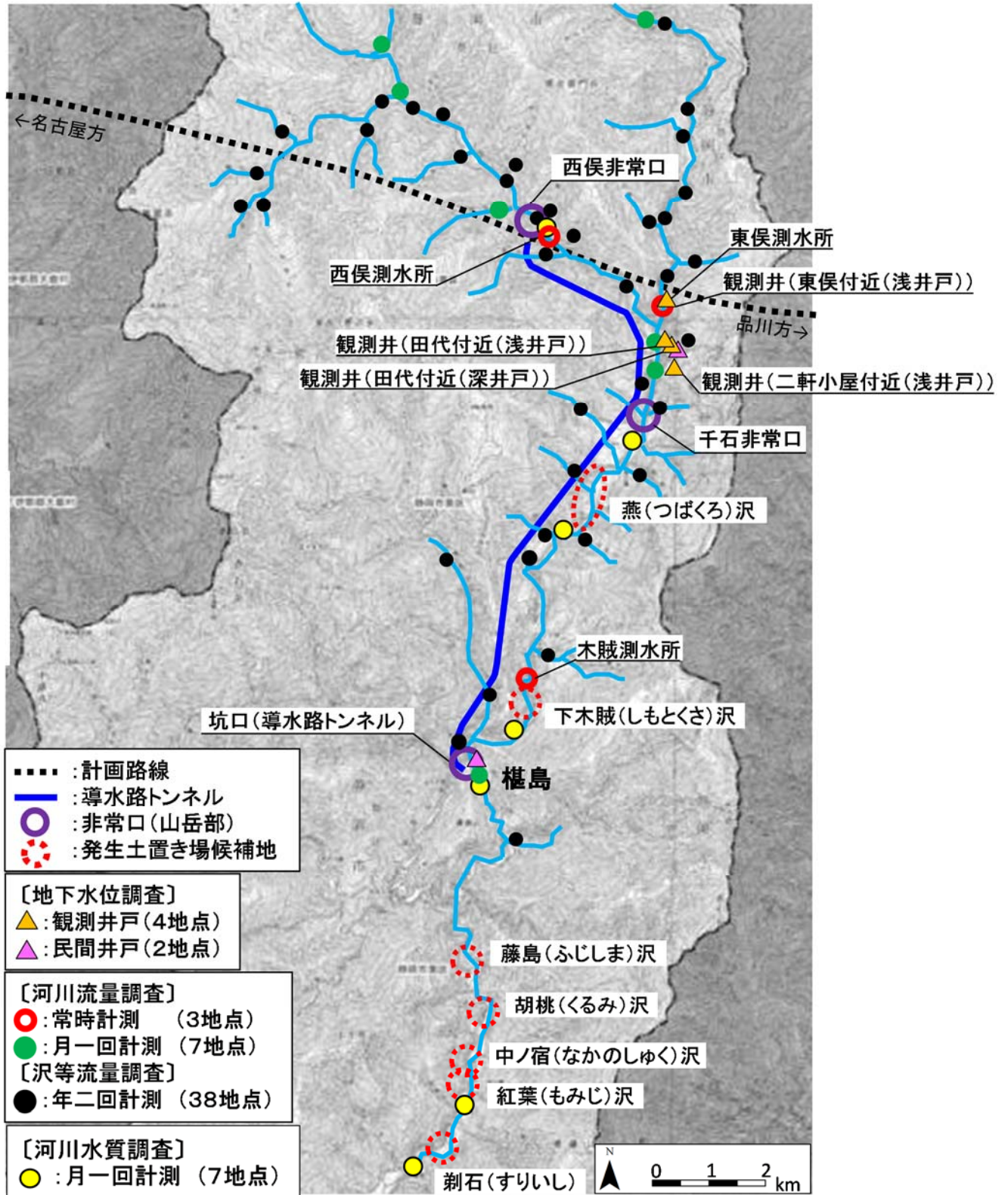
図 4.2 工事着手前に実施した調査地点図(上流域)
