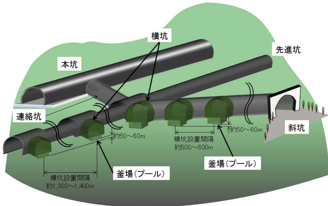
図 4.28 横坑と釜場（プール）の設置イメージ図
