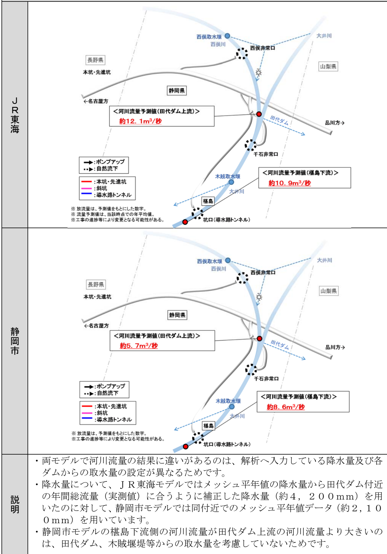
図 4.13 トンネル掘削前の予測結果
