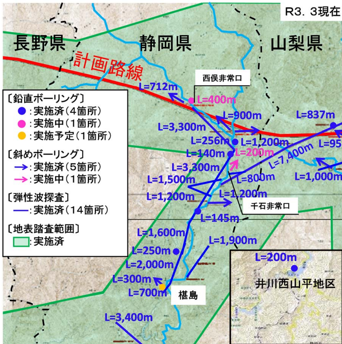
図 4.1 静岡県内の地質調査位置図
