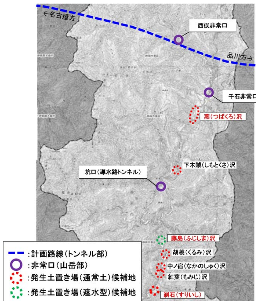
図 4.38 発生土置き場計画位置図
