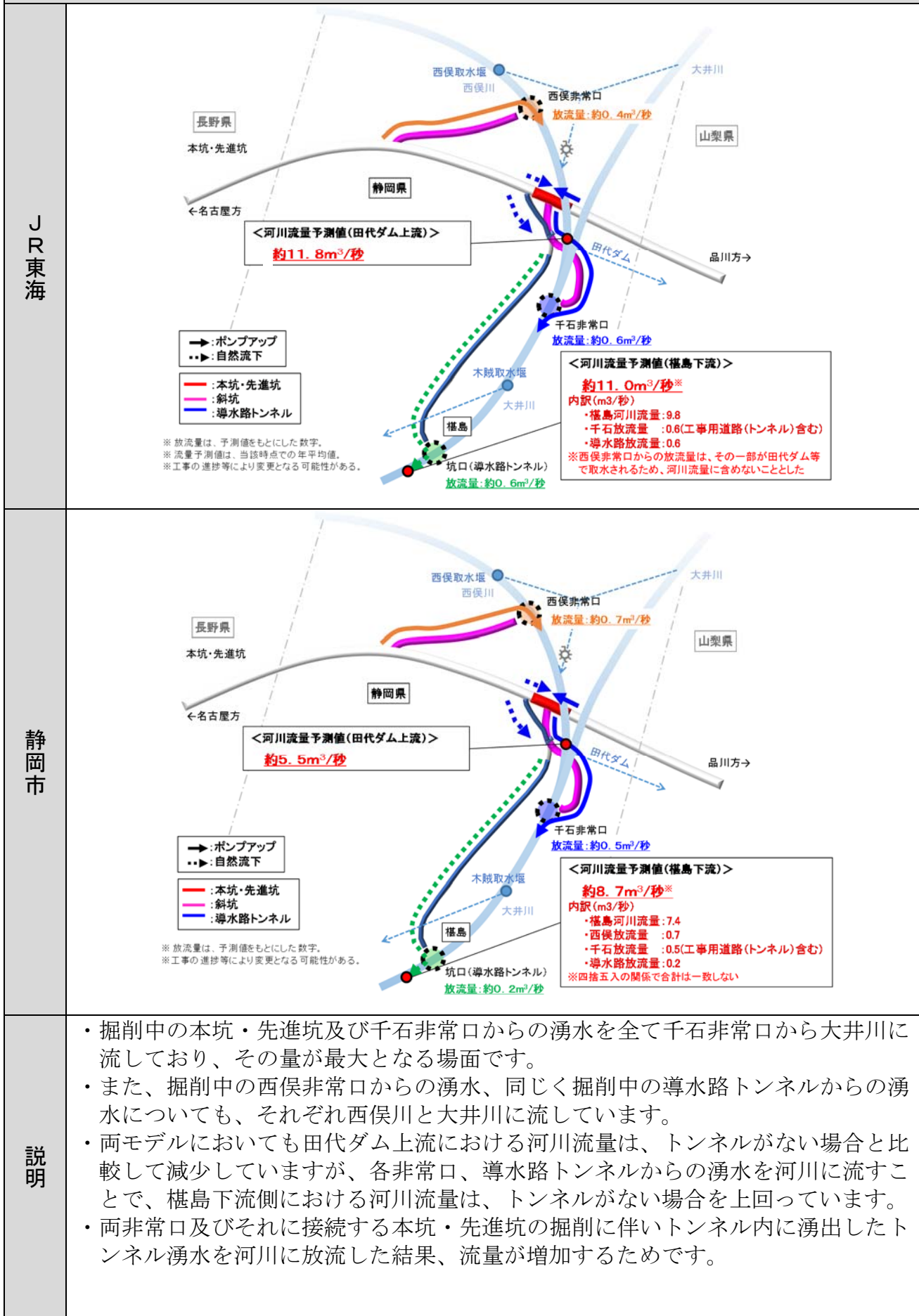
図 4.14 千石非常口～導水路トンネル間が貫通する時期の予測結果
