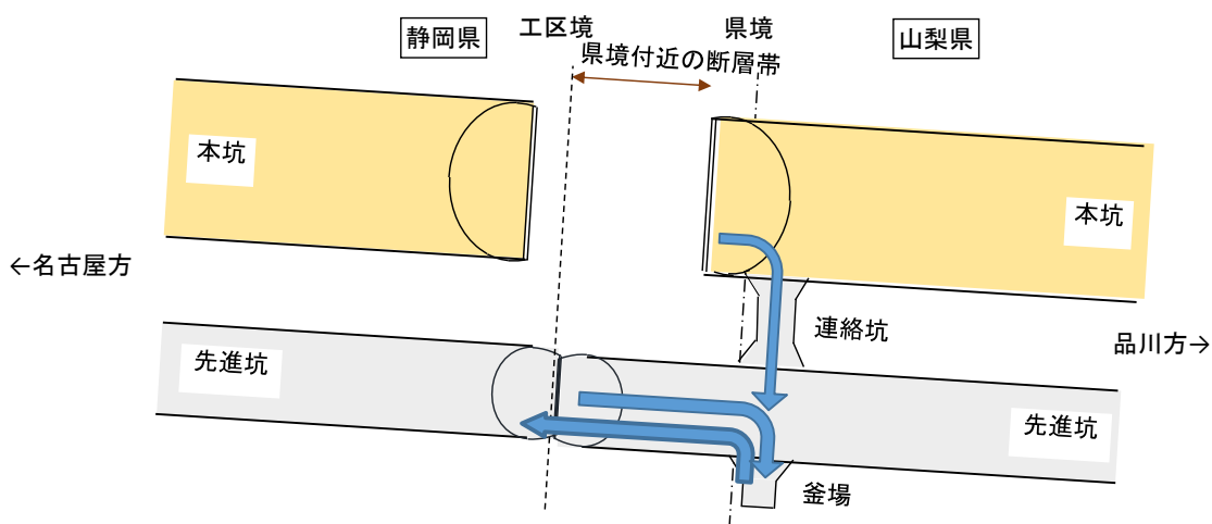
図 4.47 先進坑貫通後のトンネル湧水ポンプアップ
