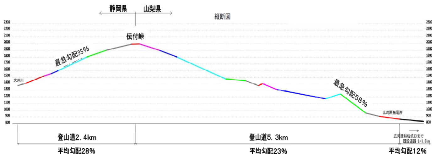
図 4.55 計画縦断面図
