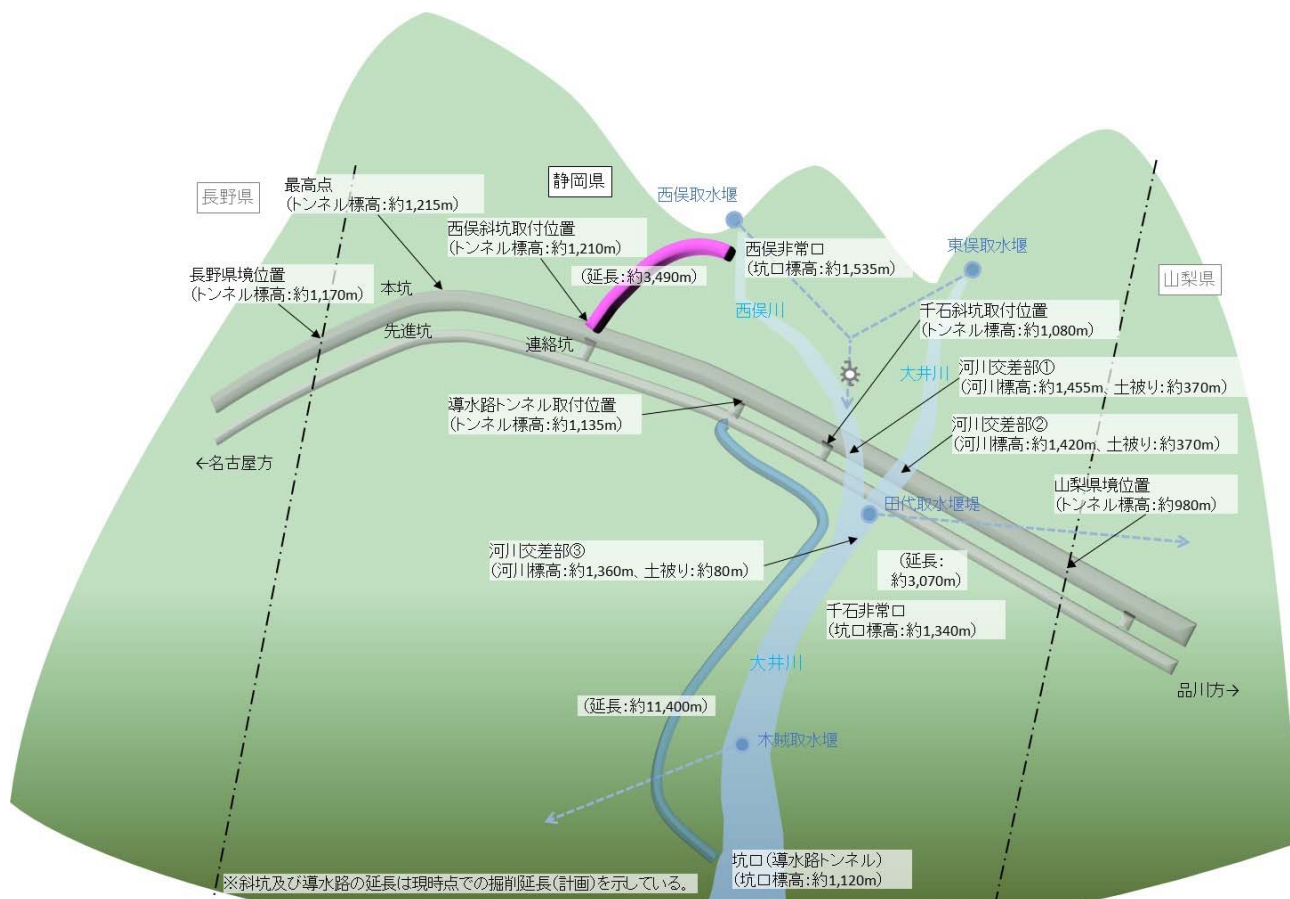
図 4.12 【参考】トンネルの位置関係図
