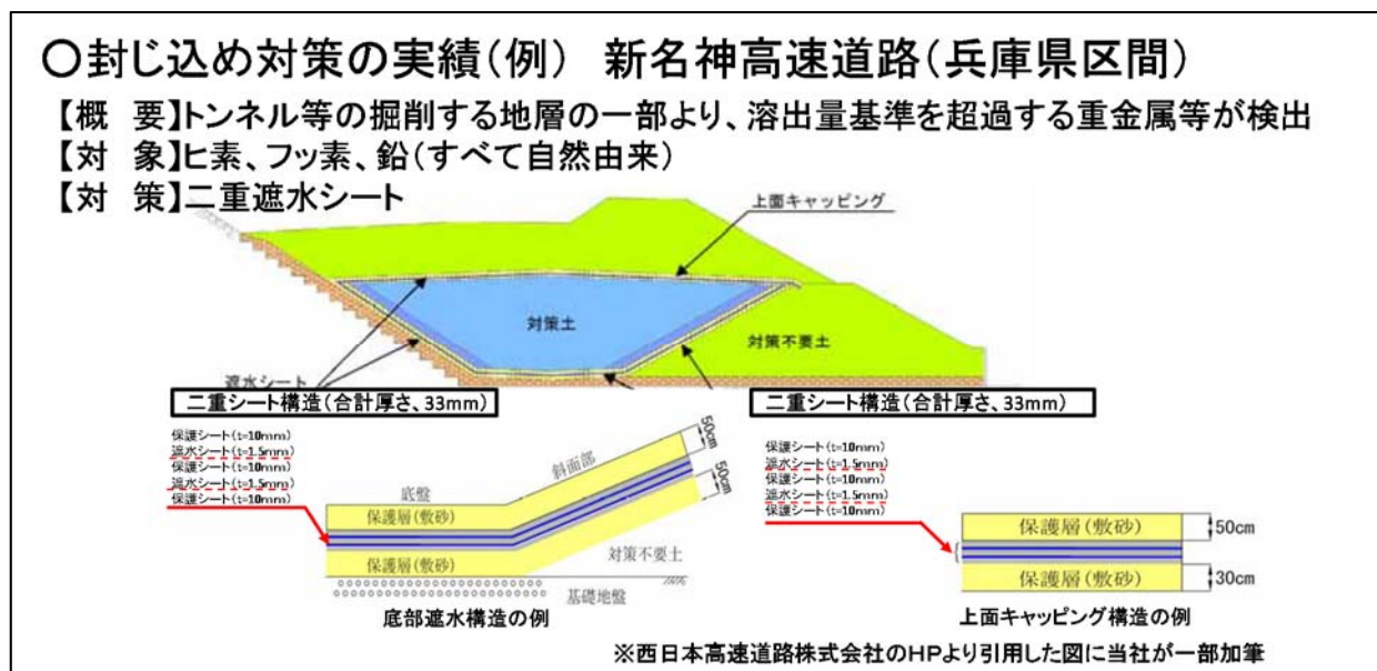
図 4.39 封じ込め対策の実績例
