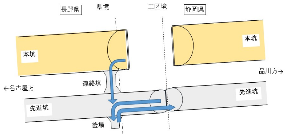
図 4.69 長野県側先進坑貫通後のトンネル湧水ポンプアップ
