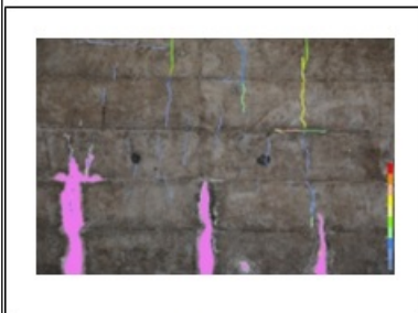
図3 ひびわれ・遊離石灰
