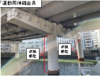
梯子が無い橋脚柱内部を橋梁より点検
