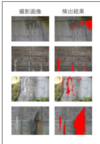
図5 遊離石灰検出例
