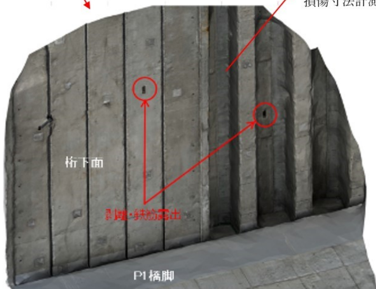
損傷寸法計測
