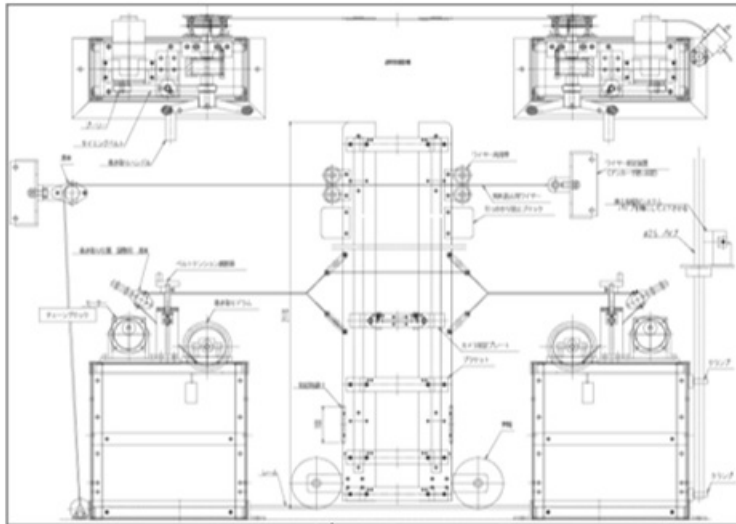
ビデオスコープガイド・巻取り機 詳細図
