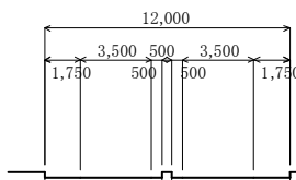
標準断面図
