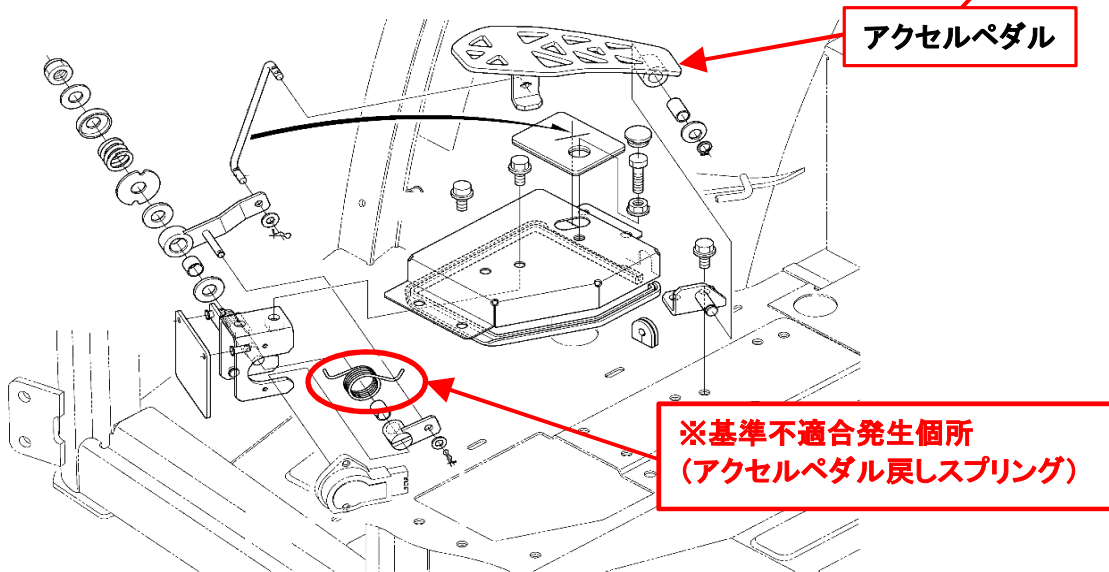
図3. アクセルペダル周辺の部品図
