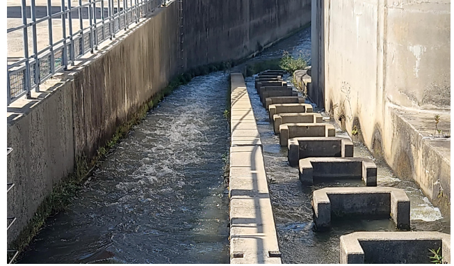
牟呂松原頭首工魚道
