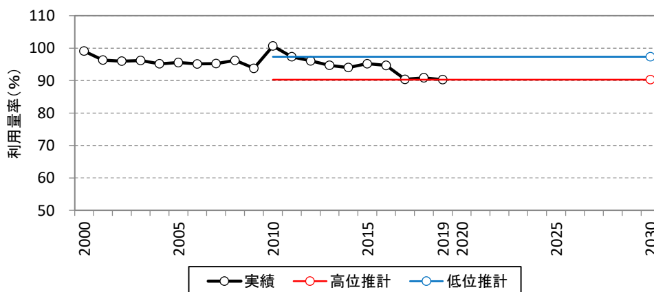
図 87 次期フルプランにおける工業水道利用率（佐賀県）
