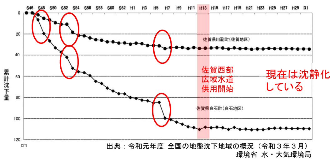
佐賀地区及び白石地区における地盤沈下の推移
