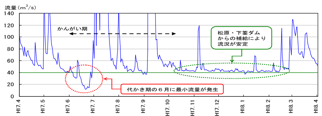
筑後川瀬ノ下地点実測流量図(平成17年度)
