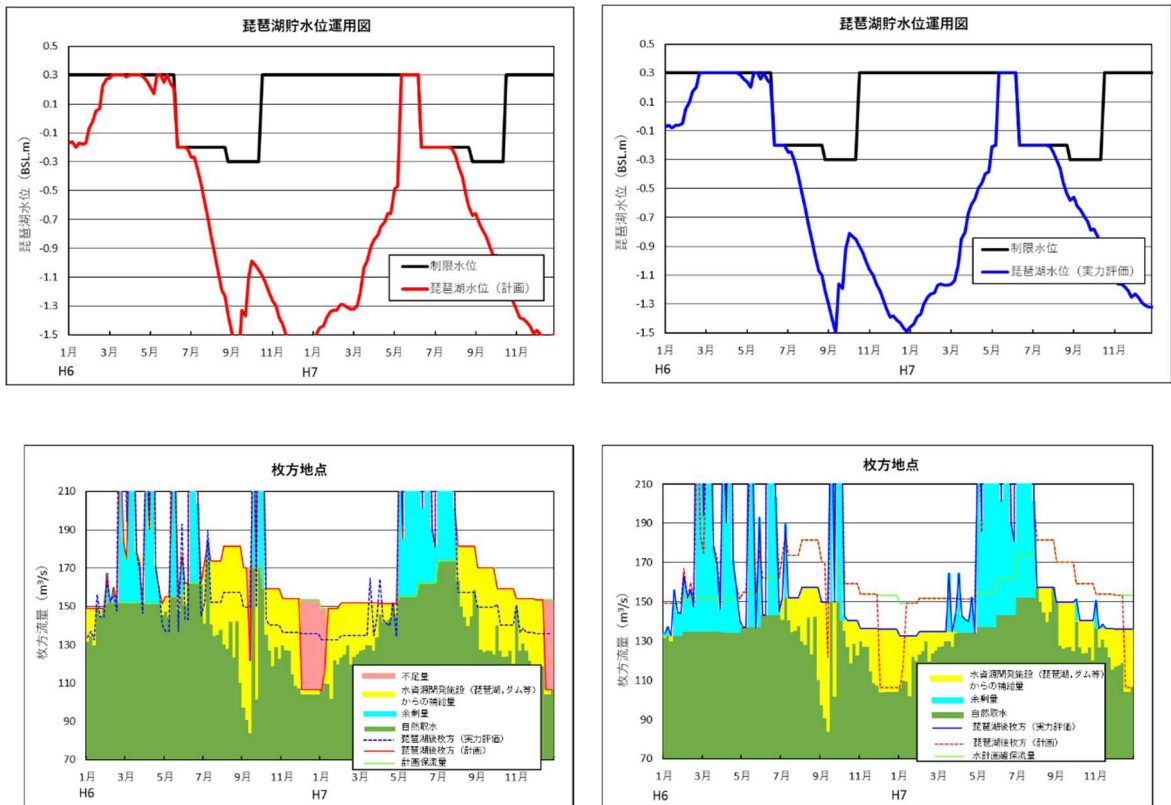
図 128 ダム開発水量と供給可能量（淀川水系：枚方地点の例）【1/10】
