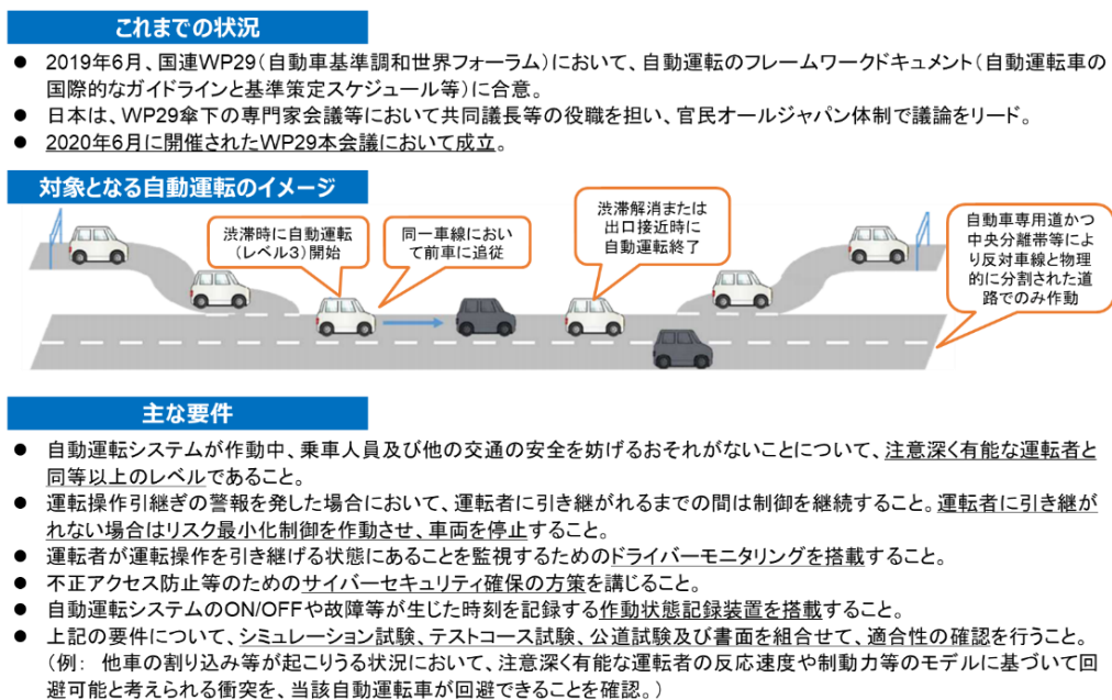
図 2-1-11. 自動運行装置の保安基準等の概要
