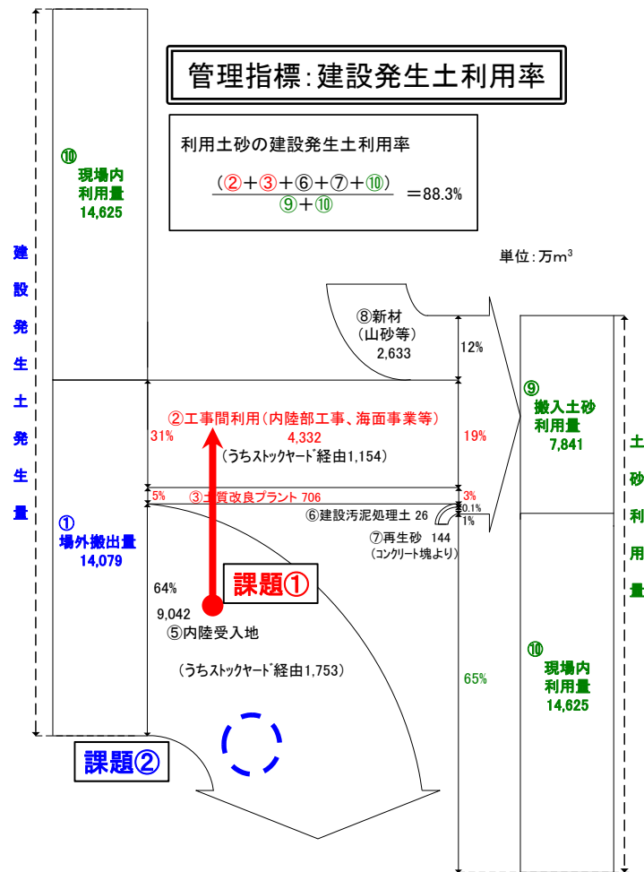
建設発生土のリサイクルフロー
