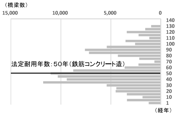
橋梁の平均年齢：約60年
