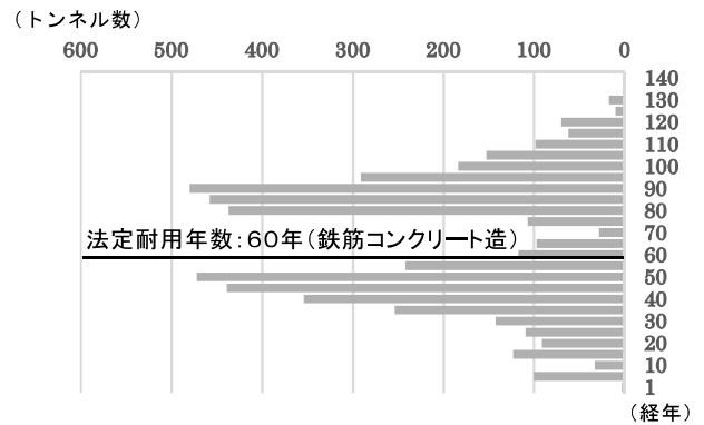
トンネルの平均年齢：約70年
