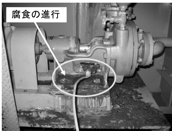
排水設備の劣化
