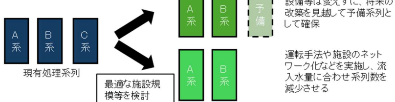
図 3-2 現有処理能力と流入水量実績による現状評価の例
