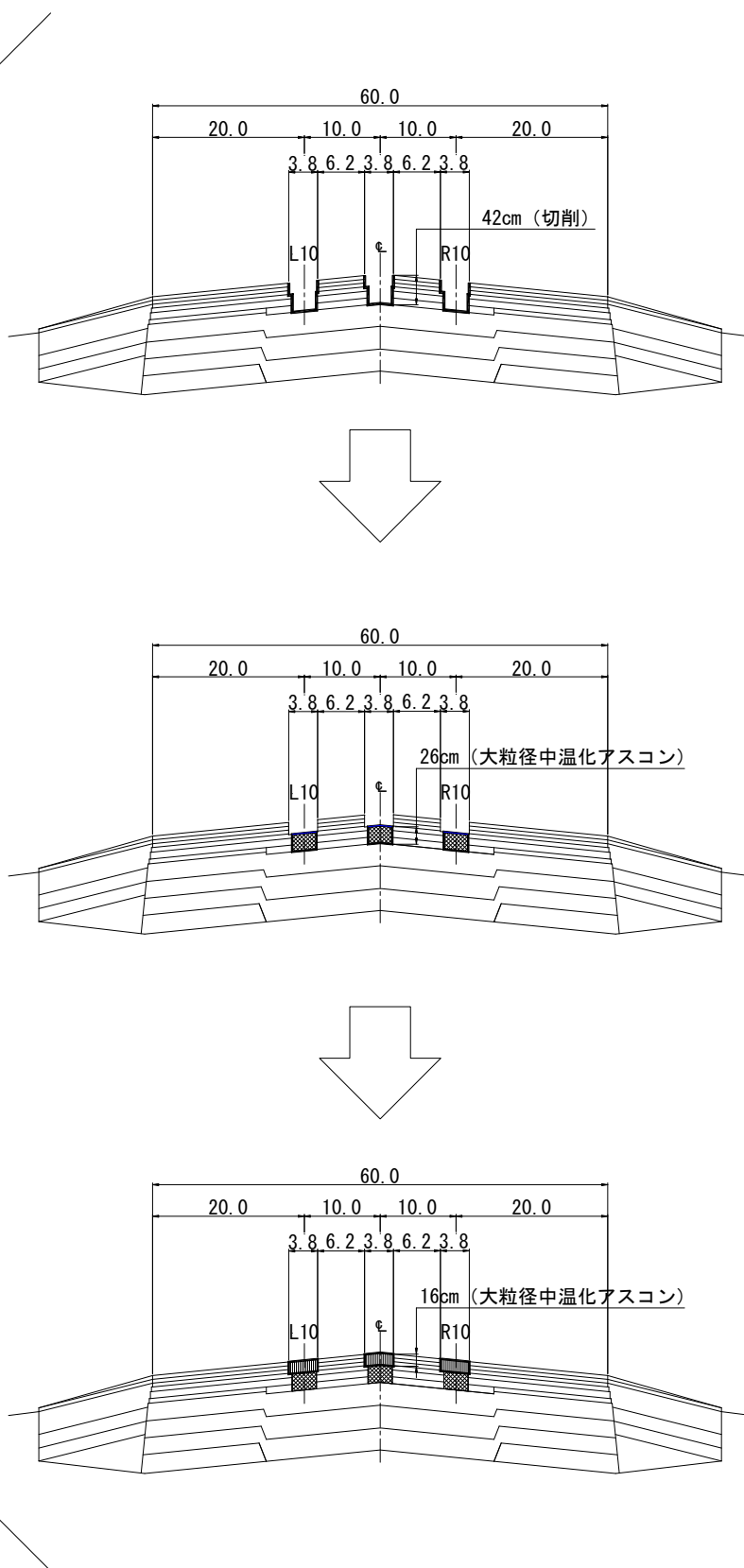
例図-7.2.2 第1工程
