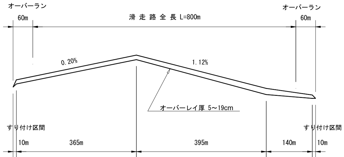
例図-7.1.3 滑走路オーバーレイ縦断面図
