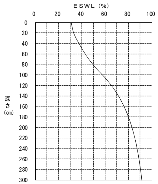
例図-1.8 B747-400D
