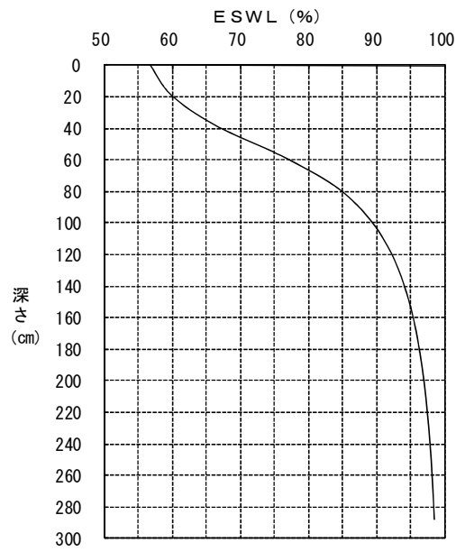
例图-1.32 MD81
