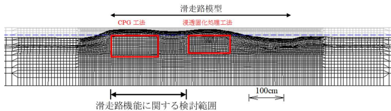
(c) Y1 断面の解析結果（沈下後）
