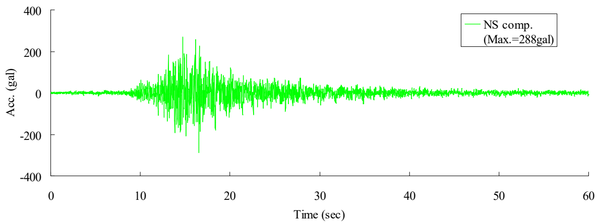
(a) NS 成分
