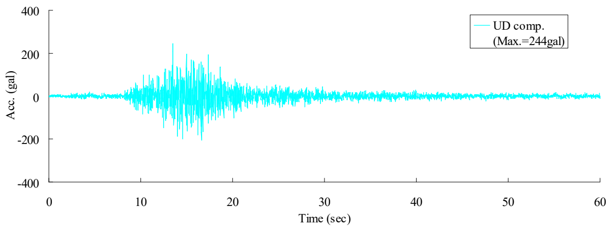
(c) UD 成分
