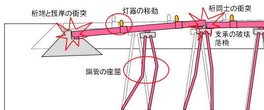
図-付 6.2 被災例
