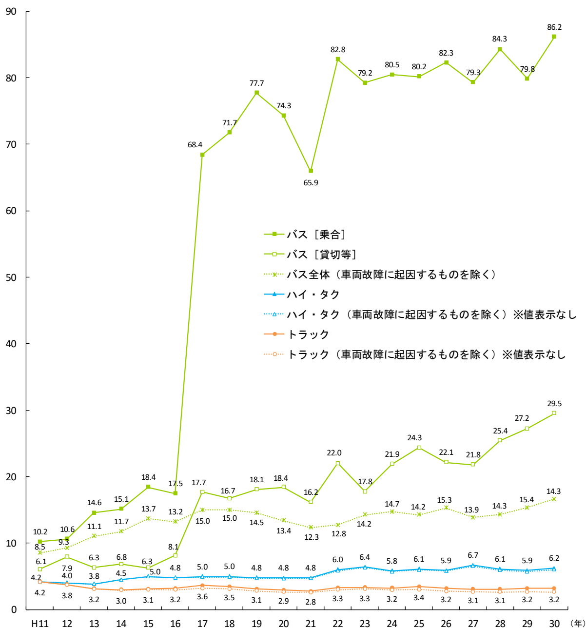
〔図 2-3〕 事業の種類別の事業用自動車 1 億走行キロ当たり重大事故件数の推移
