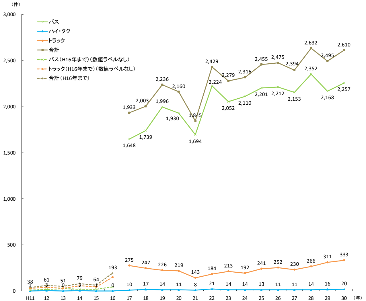
〔図3-18〕 事業の種類別の車両故障に起因する重大事故発生状況の推移
