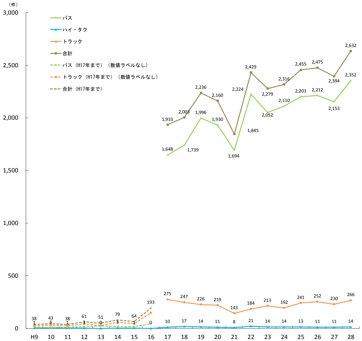
〔図3-18〕 事業の種類別の車両故障に起因する重大事故発生状況の推移
