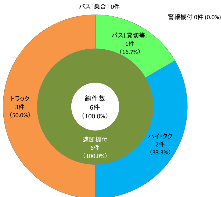
〔図3-6〕 事業の種類別、踏切種類別の踏切事故発生状況（乗務員に起因するもの）
