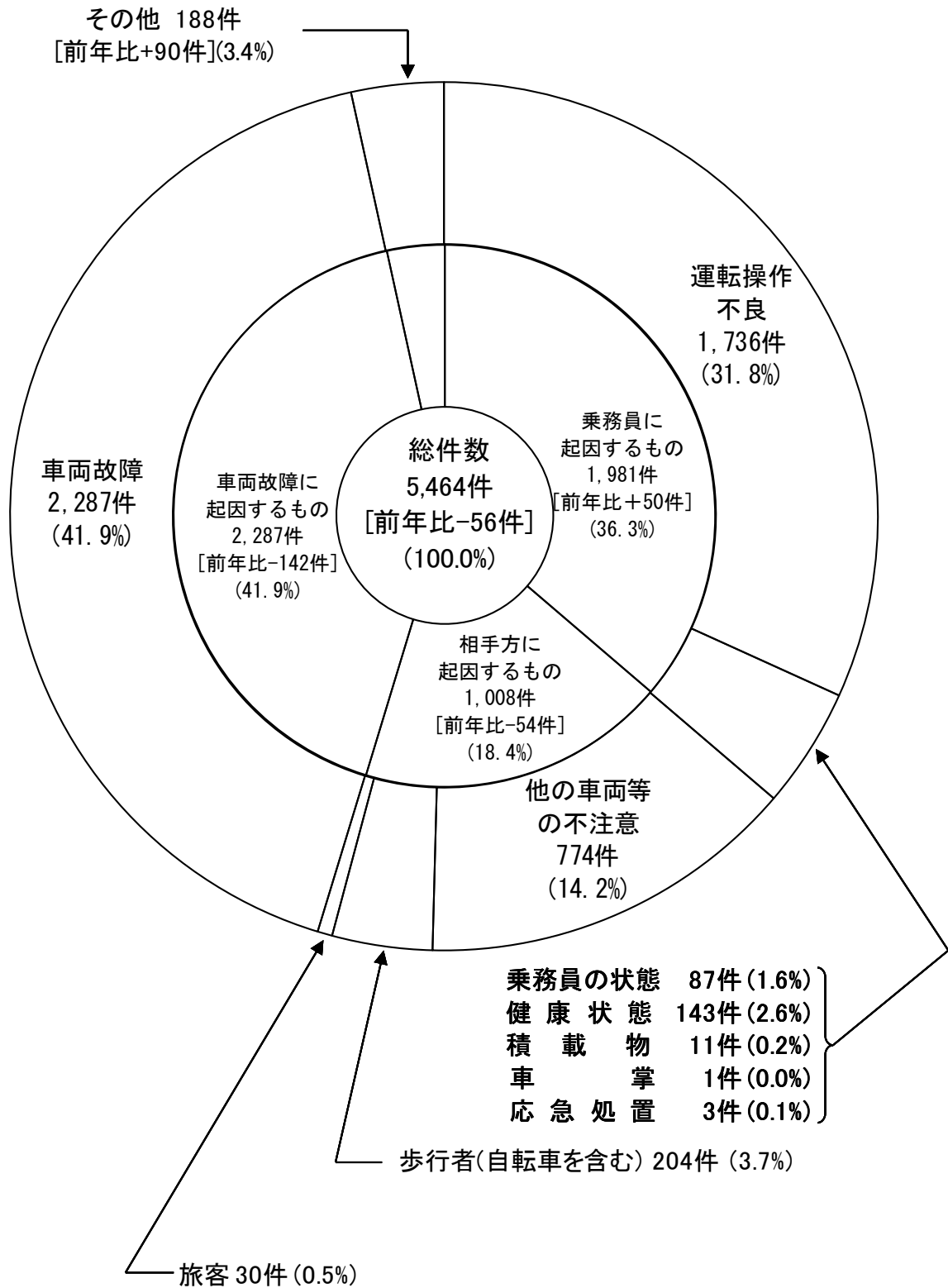
[図 3-1] 原因別重大事故発生状況
