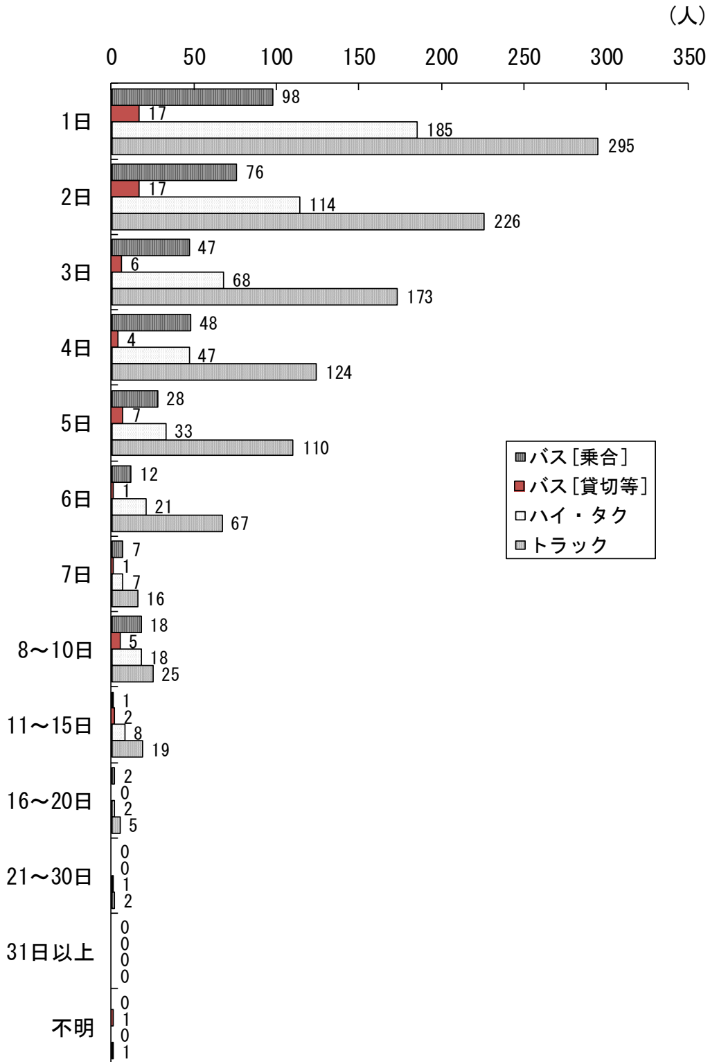
〔図3-16〕 事業の種類別の事故発生運転者の休日から事故までの勤務日数の分布
