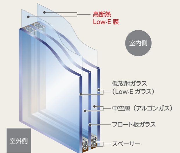
Low-E 三層複層ガラス (Low-E 2枚) アルゴンガス封入
